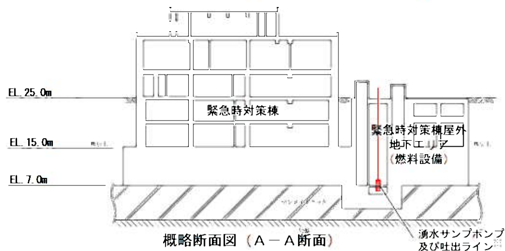
建屋諸元
