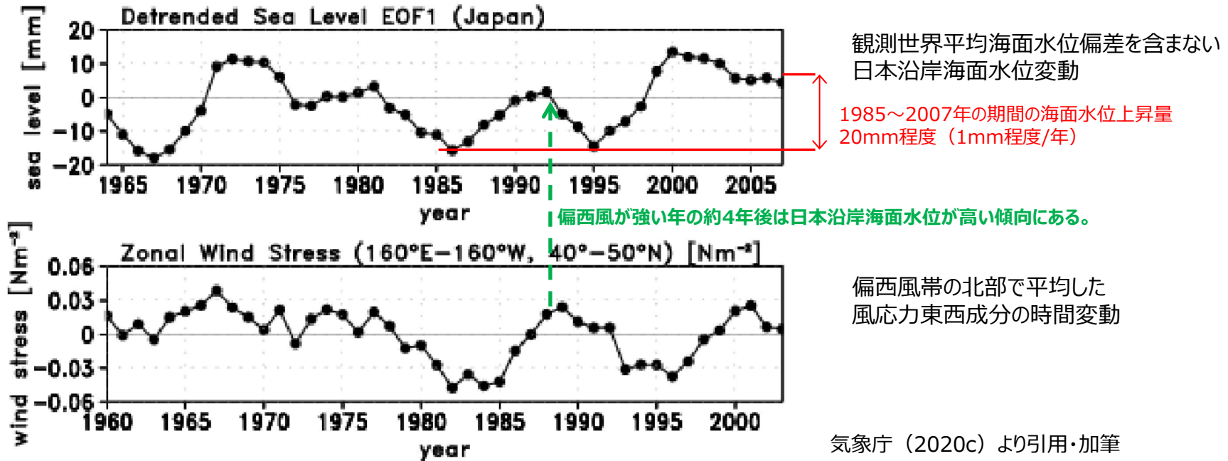
北太平洋の冬季偏西風の強度変動
