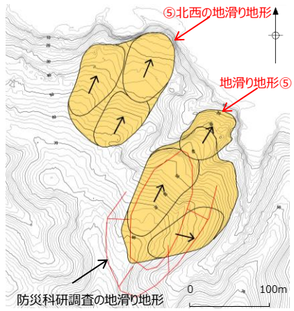
地滑り地形⑤及び 敷地北西方の地滑り地形周辺の 旧地形図
