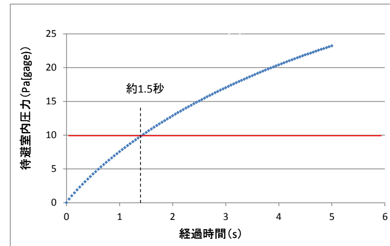
第3図 待避室内圧力変化
