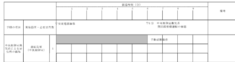
第 1.16-2 図 中央制御室換気系による居住性の確保タイムチャート (全交流動力電源が喪失した場合)
