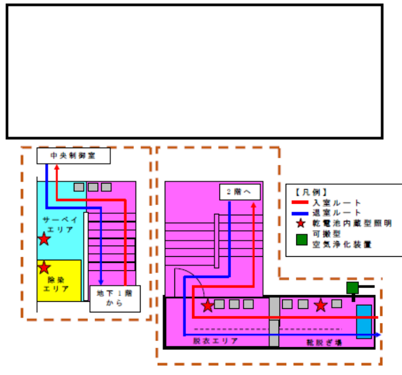
図 2.3-1 中央制御室チェンジングエリア設営場所及び概略図
