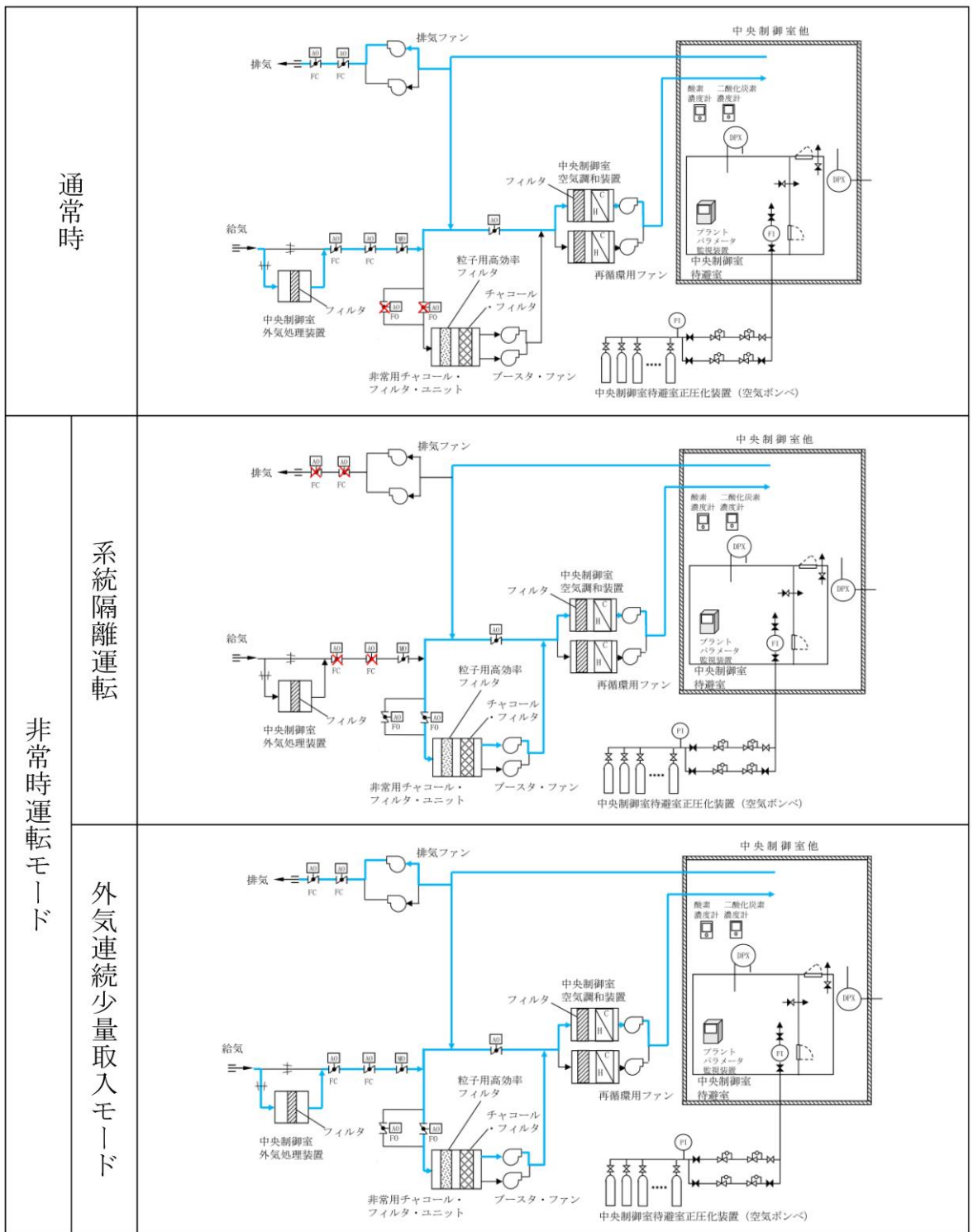
図 3.4-1 運転モード毎の中央制御室換気系 系統概要図
