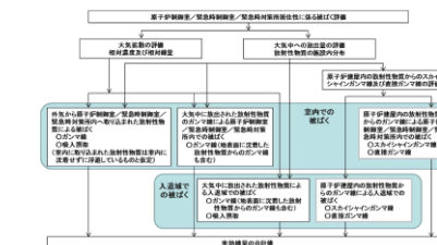
図3 原子炉制御室/緊急時対策室/緊急時対策所の居住性に係る被ばく評価手順
