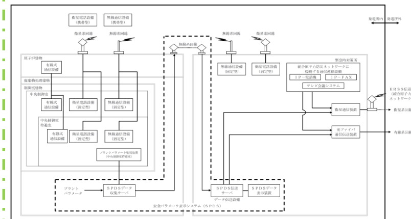
図 2.4-19 プラントパラメータ監視装置 (中央制御室待避室) のデータ伝送 概要図
