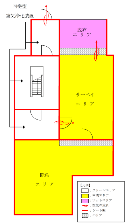
第 3.3-12 図 中央制御室へアクセスする階段の周囲の区画
