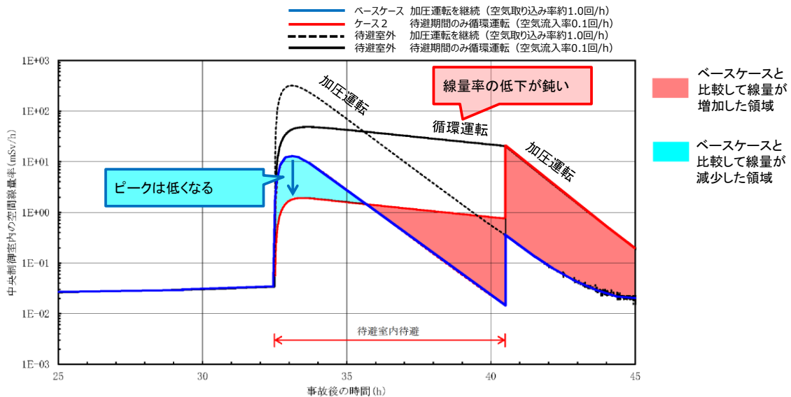
図 24-1 中央制御室内の空間線量率の推移
