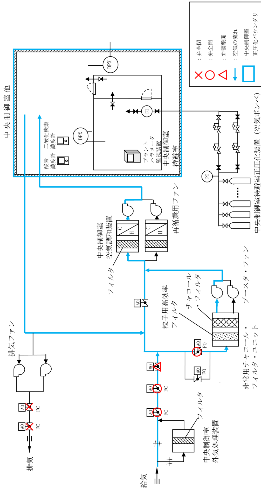
図 59-4-4 中央制御室換気系及び中央制御室待避室正圧化装置（空気ポンプ）概略系統図 （非常時運転モード（加圧運転（プルーム通過前及びプルーム通過後）））
