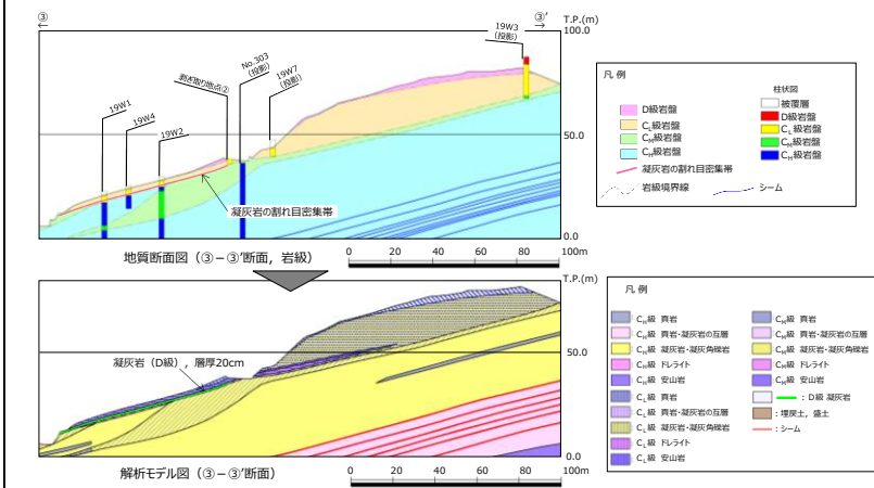
図2-36 ③-③'断面のモデル化
