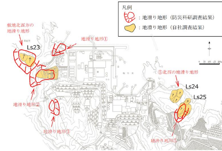
図2-49 敷地周辺地すべり位置図
