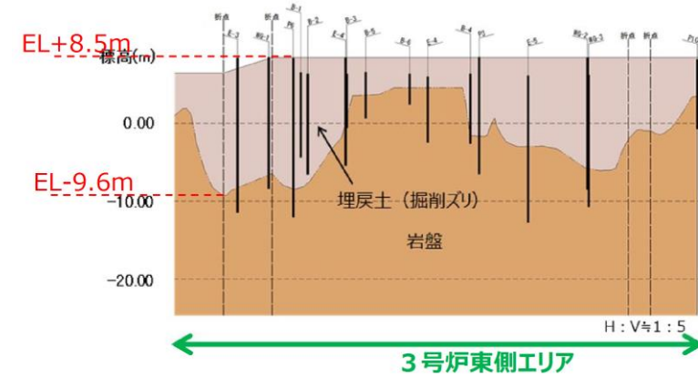
図 3-9 (1) 地質断面図 (3号炉東側エリア)
