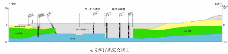
添付第4-7 図(2) 地質断面図 (3, 4号炉汀線直交断面図)
