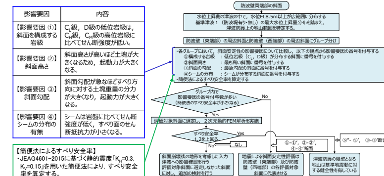
図2-25 評価対象斜面の選定に用いる影響要因等
