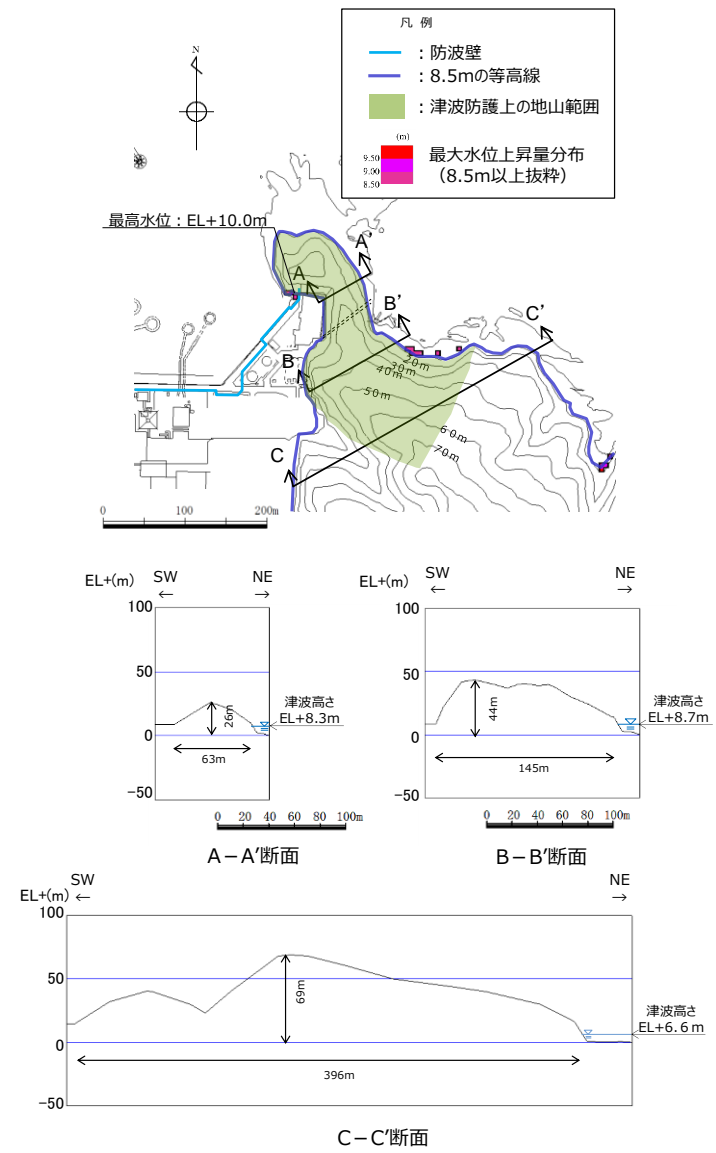
図2-5(1) 防波壁(東端部)の地形断面図
