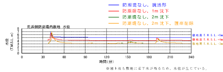
添付第 4-40 図 沈下・斜面崩壊の有無に対する水位時刻歴波形の比較
