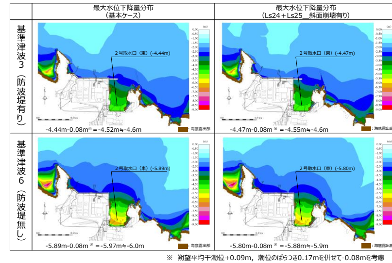
図 2-51 (4) 斜面崩壊 (Ls24+Ls25) の有無による最大水位下降量分布の比較 (基準津波 3 (防波堤有り) 及び基準津波 6 (防波堤無し))
