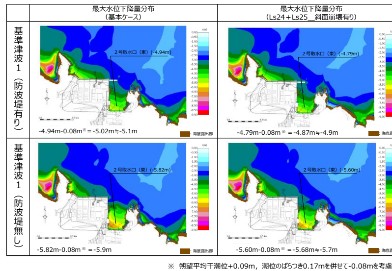
図2-51 (3) 斜面崩壊 (Ls24+Ls25) の有無による最大水位下降量分布の比較 (基準津波1 (防波堤有り) 及び基準津波1 (防波堤無し))
