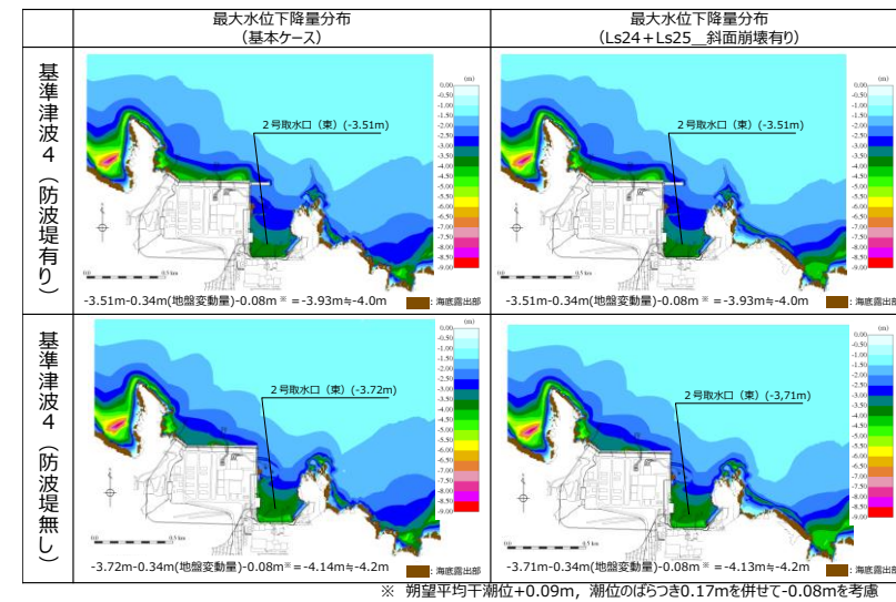
図 2-51 (5) 斜面崩壊 (Ls24+Ls25) の有無による最大水位下降量分布の比較 (基準津波 4 (防波堤有り) 及び基準津波 4 (防波堤無し))
