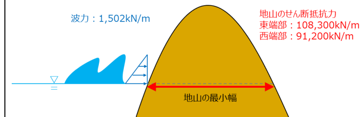
図2-44 波力と地山のせん断抵抗力の比較計算に関するイメージ
