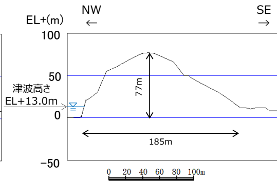
F-F'断面
