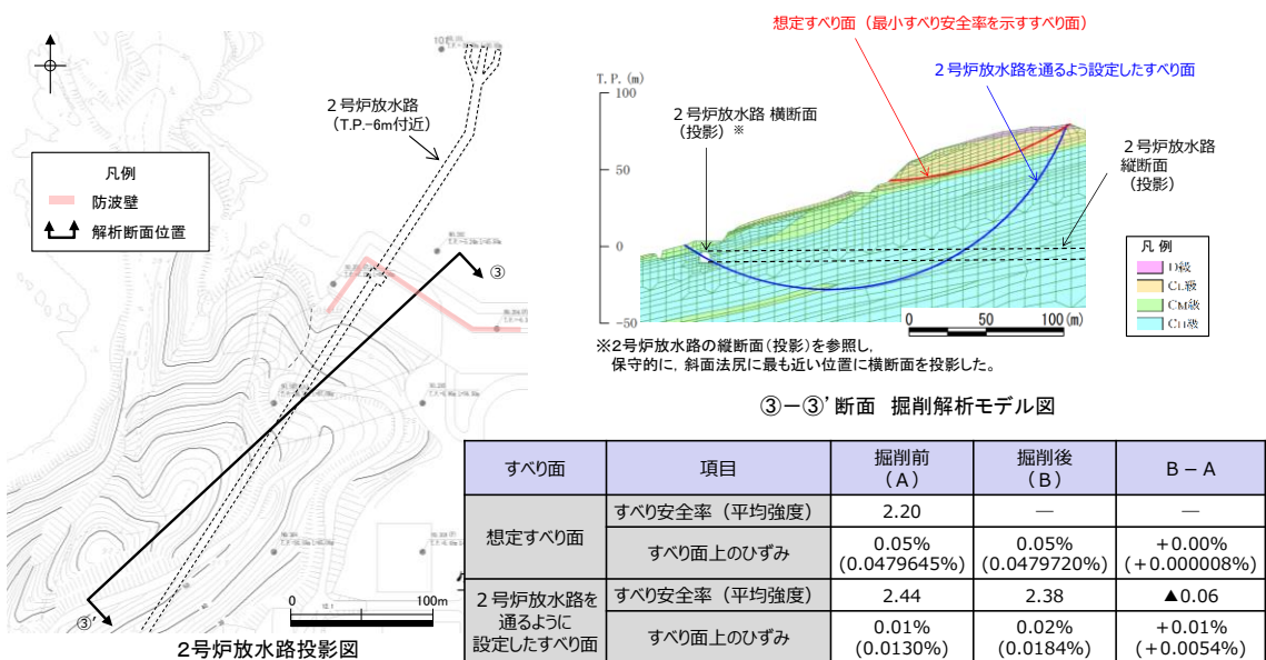
図 2-48 ③-③' 断面における 2 号炉放水路の影響検討結果
