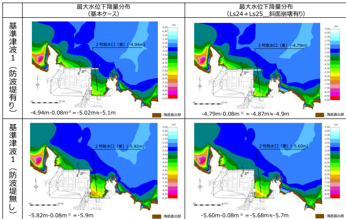
図2-51 (3) 斜面崩壊 (Ls24+Ls25) の有無による最大水位下降量分布の比較 (基準津波1 (防波堤有り) 及び基準津波1 (防波堤無し))
