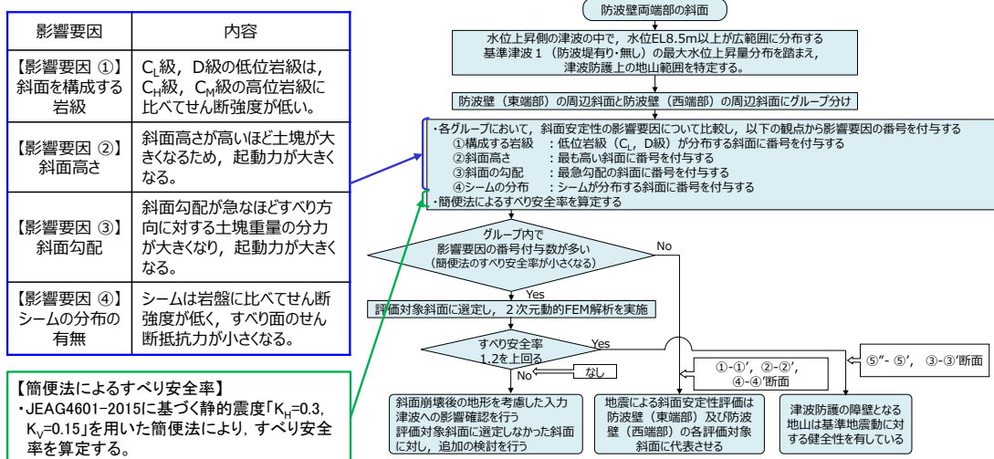
図 2-25 評価対象斜面の選定に用いる影響要因等
