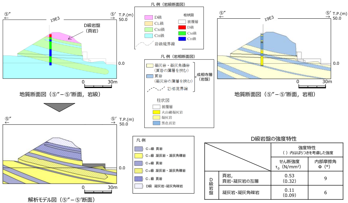
図 2-32 ⑤-⑤' 断面のモデル化
