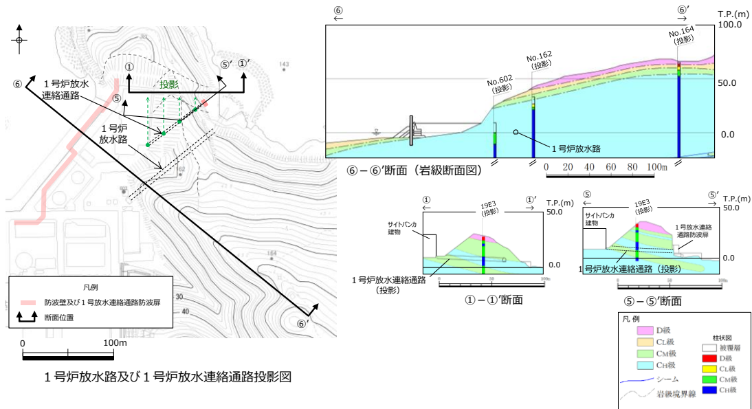
図 2-46 防波壁（東端部）のトンネルの代表性
