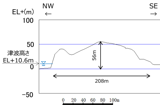
E-E'断面※
