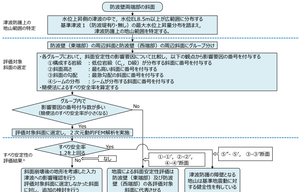
図2-23 検討フロー
