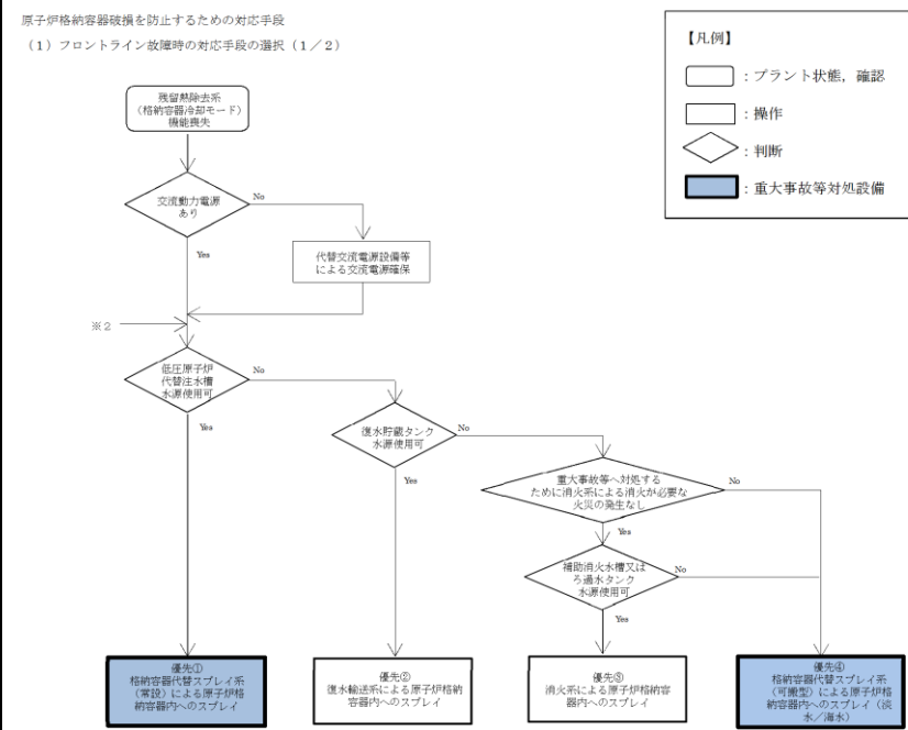
原子炉格納容器破損を防止するための対応手段 (1) フロントライン故障時の対応手段の選択 (2/2)
