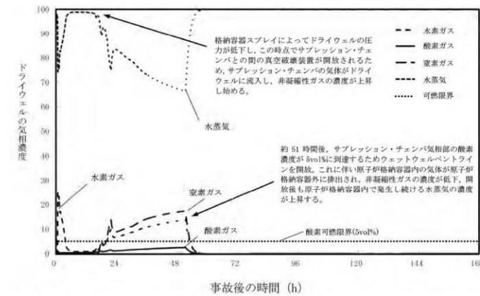
図2.3.1-3 G値を設計基準事故ベースとした場合のドライウェルの気相濃度の推移 (ウェット条件)
