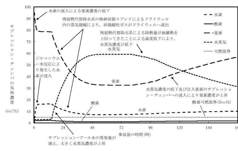
図 2.3.1-2 サブプレッション・チェンバの気相濃度の推移 (ウェット条件) 格納容器過圧・過温破損 (残留熱代替除去系を使用する場合)
