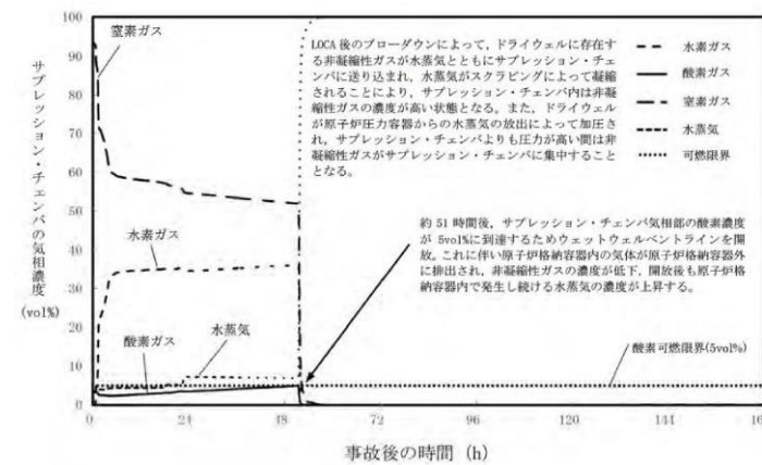
図2.3.1-4 G値を設計基準事故ベースとした場合のサプレッション・チェンバの気相濃度の推移 (ウェット条件)
