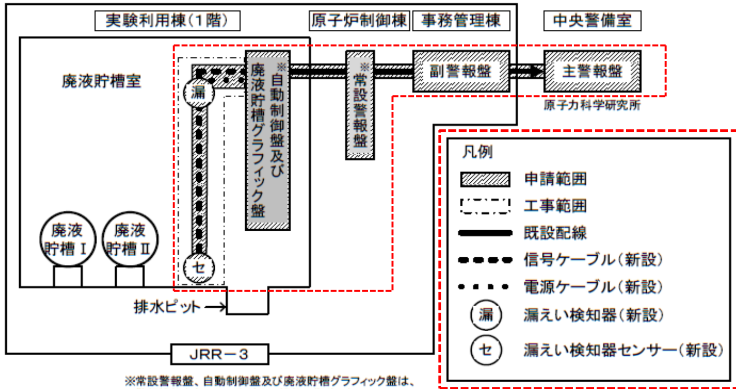
漏えい検知器の設置概要図
