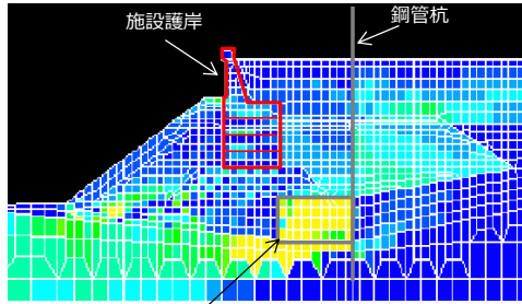
鋼管杭が海側へ変形した場合
