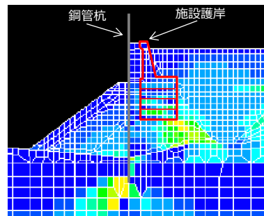
鋼管杭が陸側へ変形した場合
