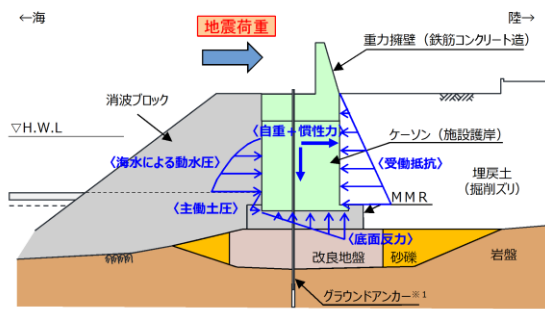
荷重図
