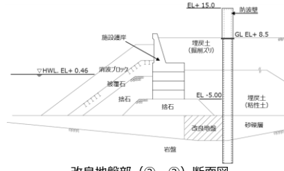
改良地盤部 (2-2) 断面図
