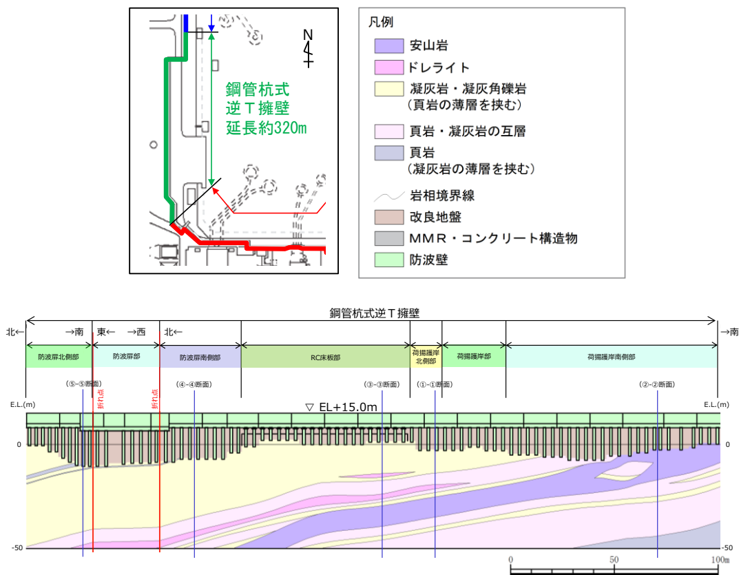
第 1-59 図 防波壁（鋼管杭式逆T擁壁）の岩相縦断図
