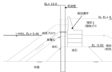
施設護岸前出し部 (3-3) 断面図
