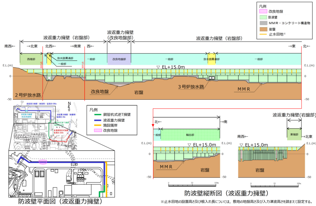
第 1-19 図 防波壁（波返重力擁壁）の縦断図
