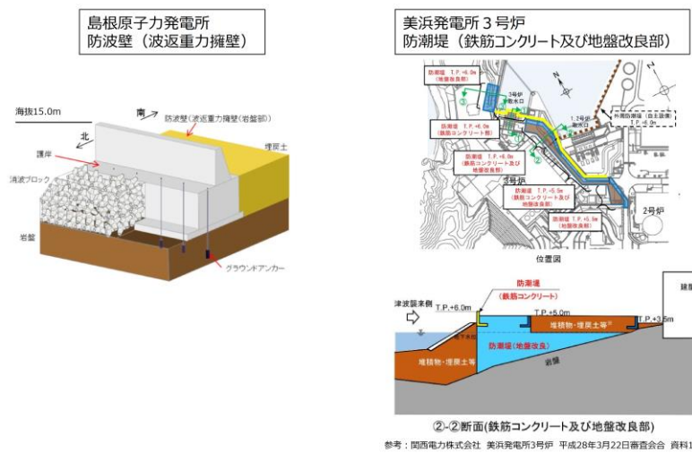
第3図 構造イメージ（島根原子力発電所 防波壁（波返重力擁壁）及び美浜発電所 防潮堤（鉄筋コンクリート及び地盤改良部））
