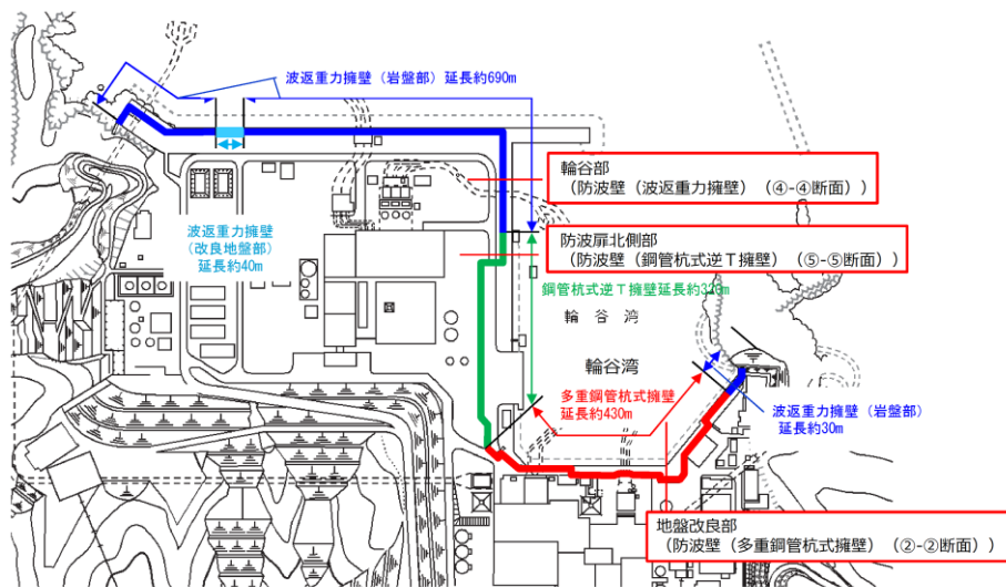
第 1-48 図 各構造形式において最大相対変形が生じる断面位置
