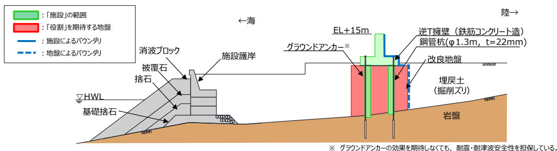
第 1-4 図 防波壁（鋼管杭式逆T擁壁）の役割を期待する範囲
