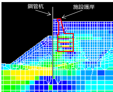
鋼管杭が海側へ変形した場合
