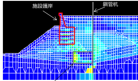
鋼管杭が陸側へ変形した場合
