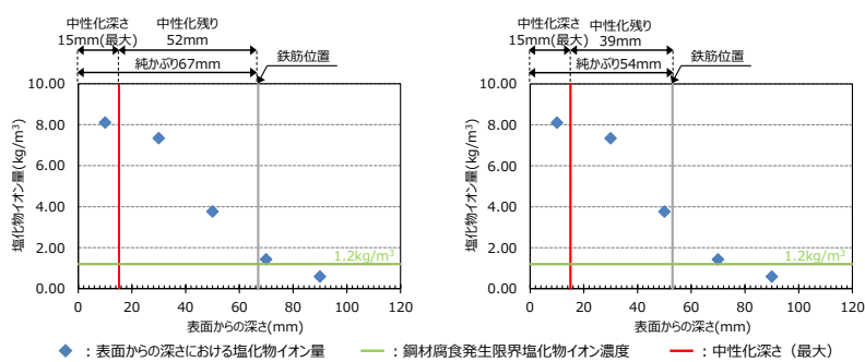
第5図 中性化試験及び塩化物イオン量試験の結果 (左図：縦筋，右図：横筋)
