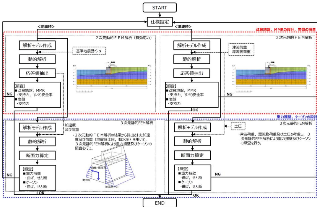
第1-105 図(1) 防波壁（波返重力擁壁）の解析概要
