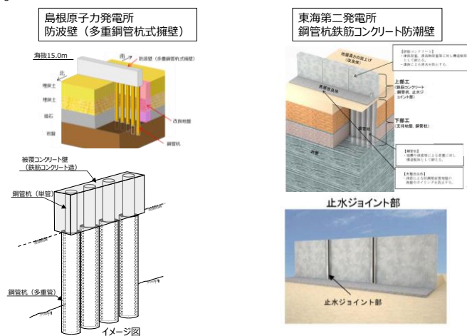
第1図 構造イメージ（島根原子力発電所 防波壁（多重鋼管杭式擁壁）及び東海第二発電所 鋼管杭鉄筋コンクリート防潮壁）
