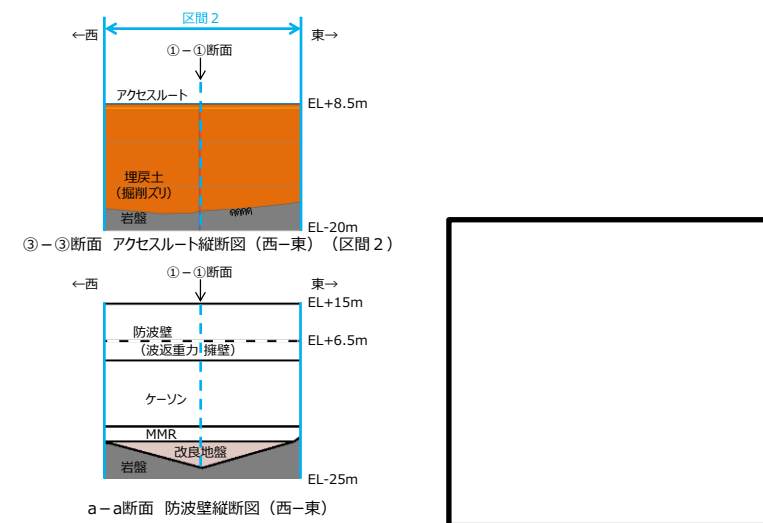
第4-24図 防波壁 (波返重力擁壁) (縦断面図)
