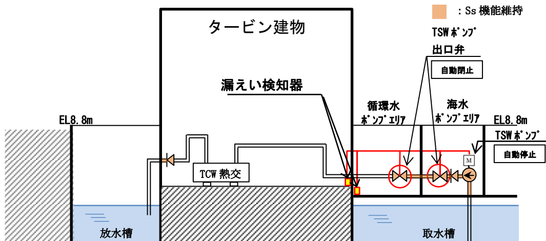
図 9-10 タービン補機海水系の対策概要図
