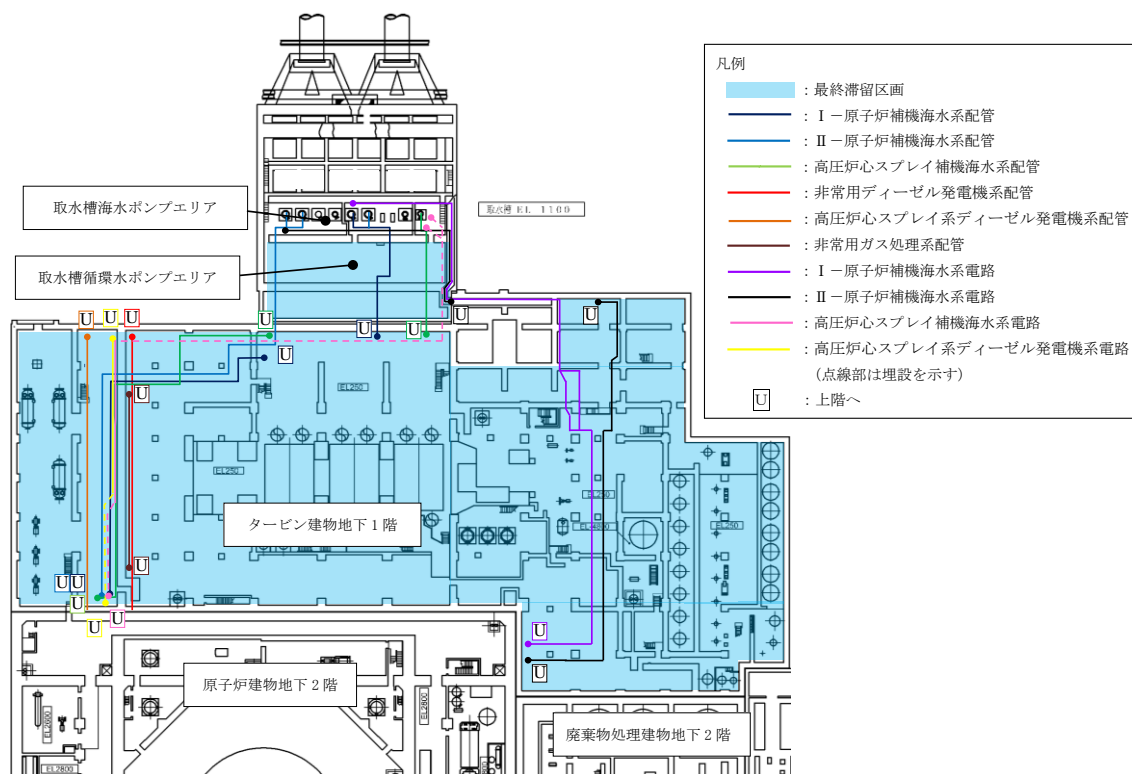
図 9-11 防護対象設備配置図
