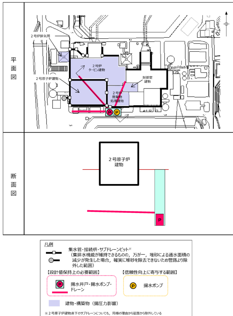
図10-4 地下水位低下設備の構成例
