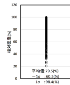
第4図 Ag2 層 (砂礫層) の相対密度
