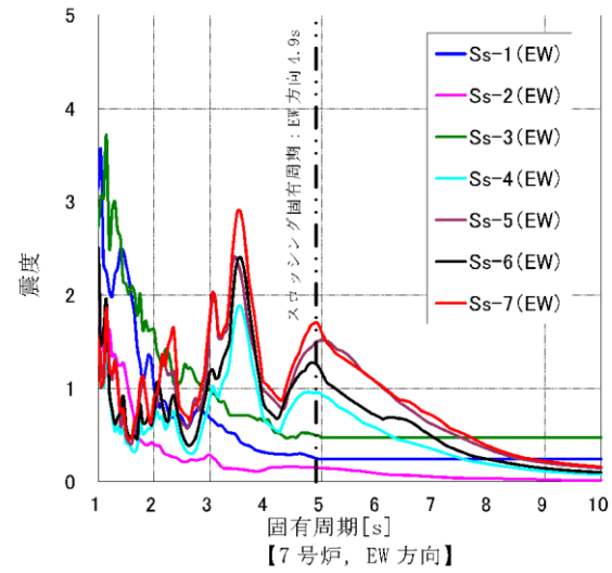
第8.1-1(2) 図 7号炉使用済燃料プールの水平方向床応答スペクトル トル (減衰定数0.5%)
