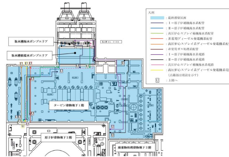
図 9-11 防護対象設備配置図
