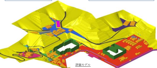
図 10-3-1 溢水伝播挙動の評価モデル
