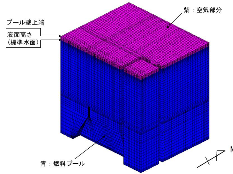
第9.1-4 図 解析モデルメッシュ概要
