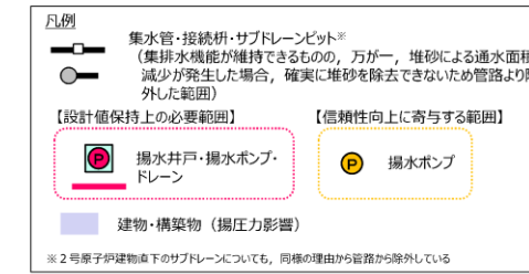
図10-4 地下水低下設備の構成例
