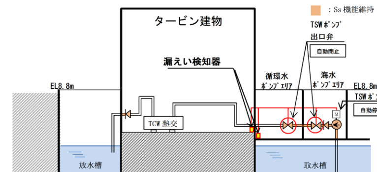
図 9-10 タービン補機海水系の対策概要図
