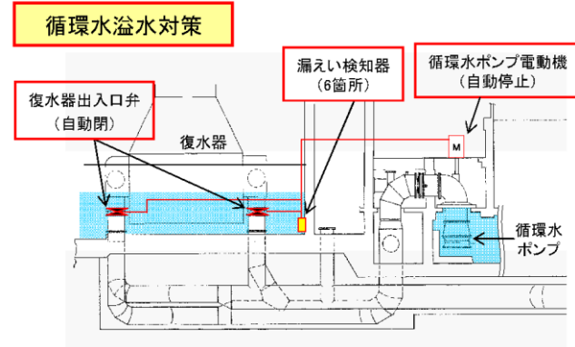
第11.2.1-1 図 循環水溢水対策イメージ
