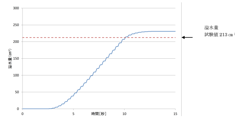
図3-5 溢水量の解析結果
