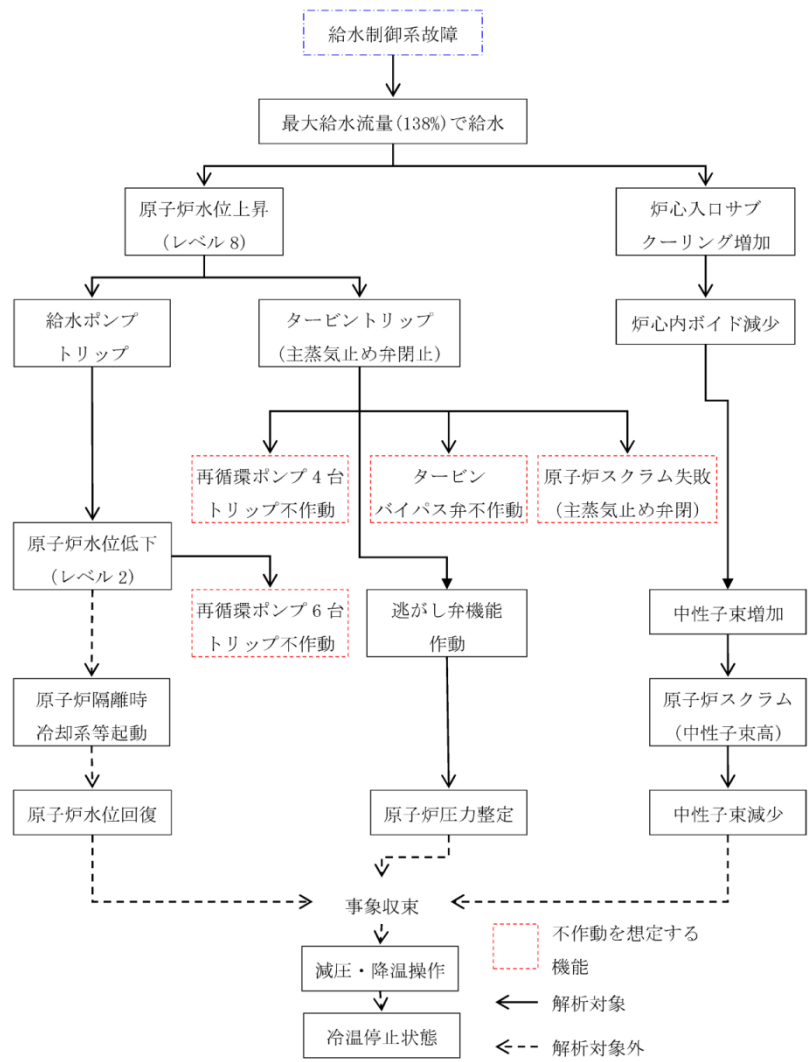
補足第 3. 6. 4. 2-2 図 給水制御系の故障事象進展フロー (タービン建屋起因)
