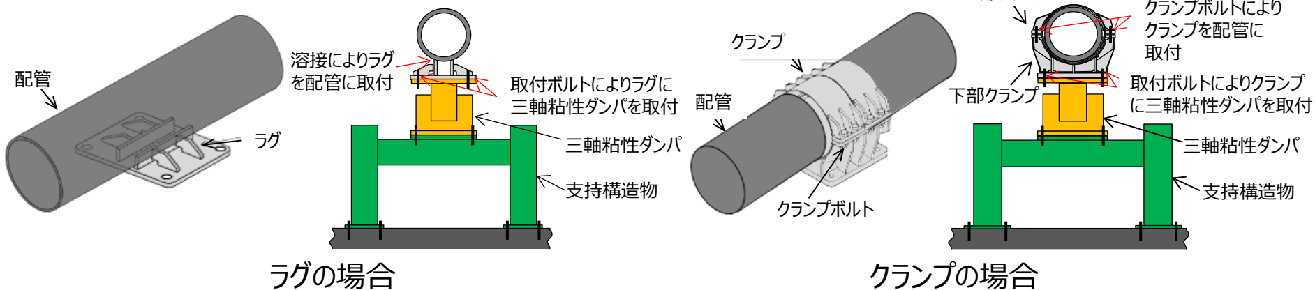
三軸粘性ダンパの配管への取付部の構造
