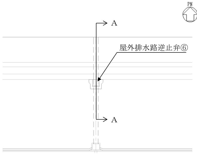
平面图
