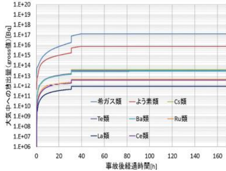
図 2-4-5 格納容器ベント実施時のベントライン経由の放出トレンド
