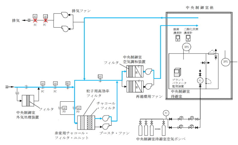
図3 中央制御室換気系の概要図
