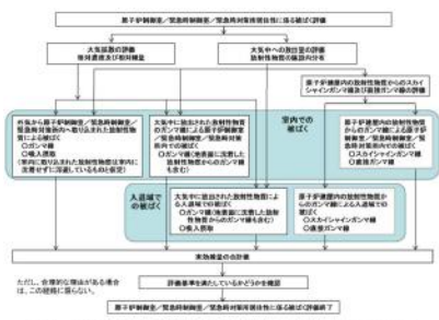
図3 原子炉制御室/緊急時対策室/緊急時対策所の居住性に係る被ばく評価手順
