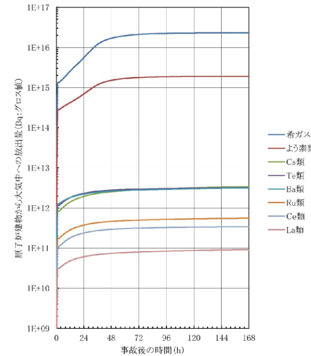
図 4-6 格納容器ベント実施時の原子炉建屋経由の放出トレンド
