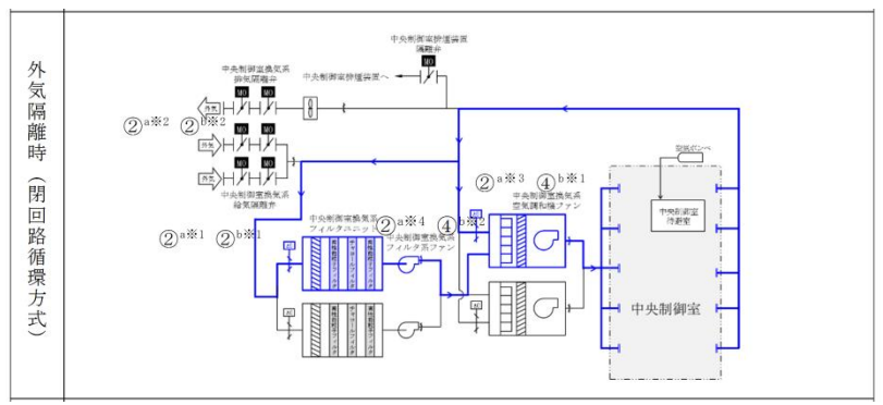
第5.1.3-2図 中央制御室換気系統構成
