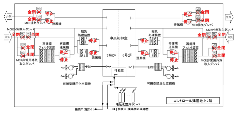
図3 6号及び7号炉中央制御室換気空調設備の概要図
