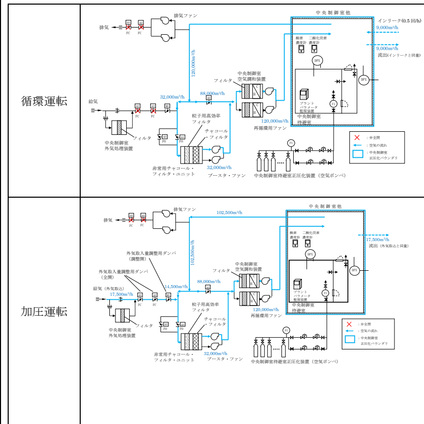
図1 中央制御室換気系 系統概要
