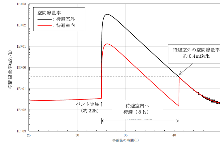
図 23-1 待避室内外の空間線量率
