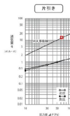
第3.7-7図 気密等級線図(A4等級)
