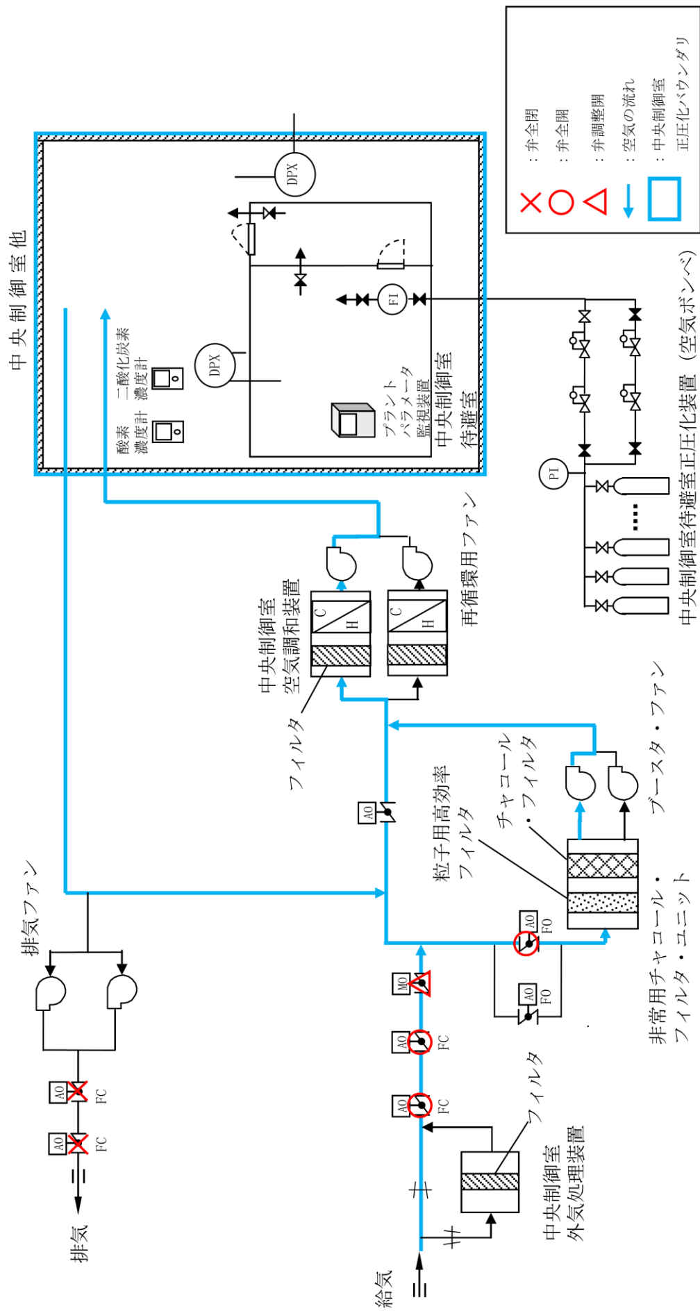
図 59-4-4 中央制御室換気系及び中央制御室待避室正圧化装置 (空気ボンベ) 概略系統図 (非常時運転モード (加圧運転 (プルーム通過前及びプルーム通過後)))
