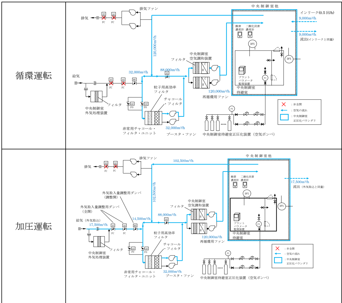
図1 中央制御室換気系 系統概要
