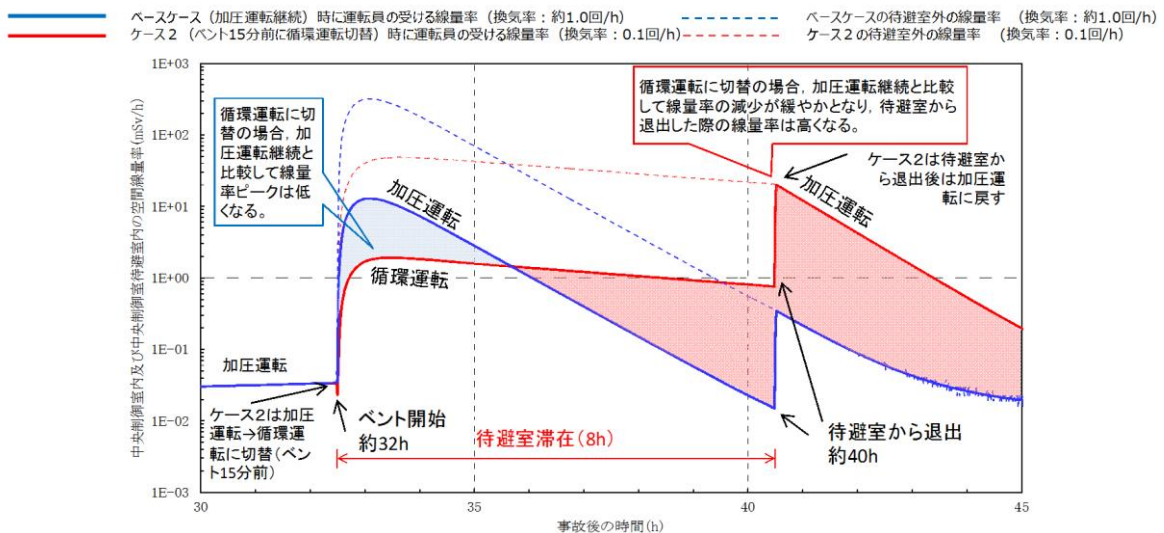
図 24-1 中央制御室内の空間線量率の推移
