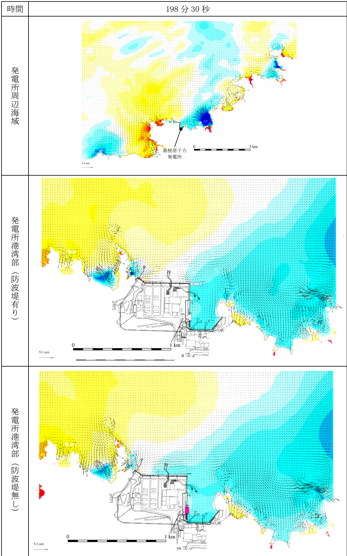
第 1 図 (198) 基準津波 1 の水位変動・流向ベクトル
