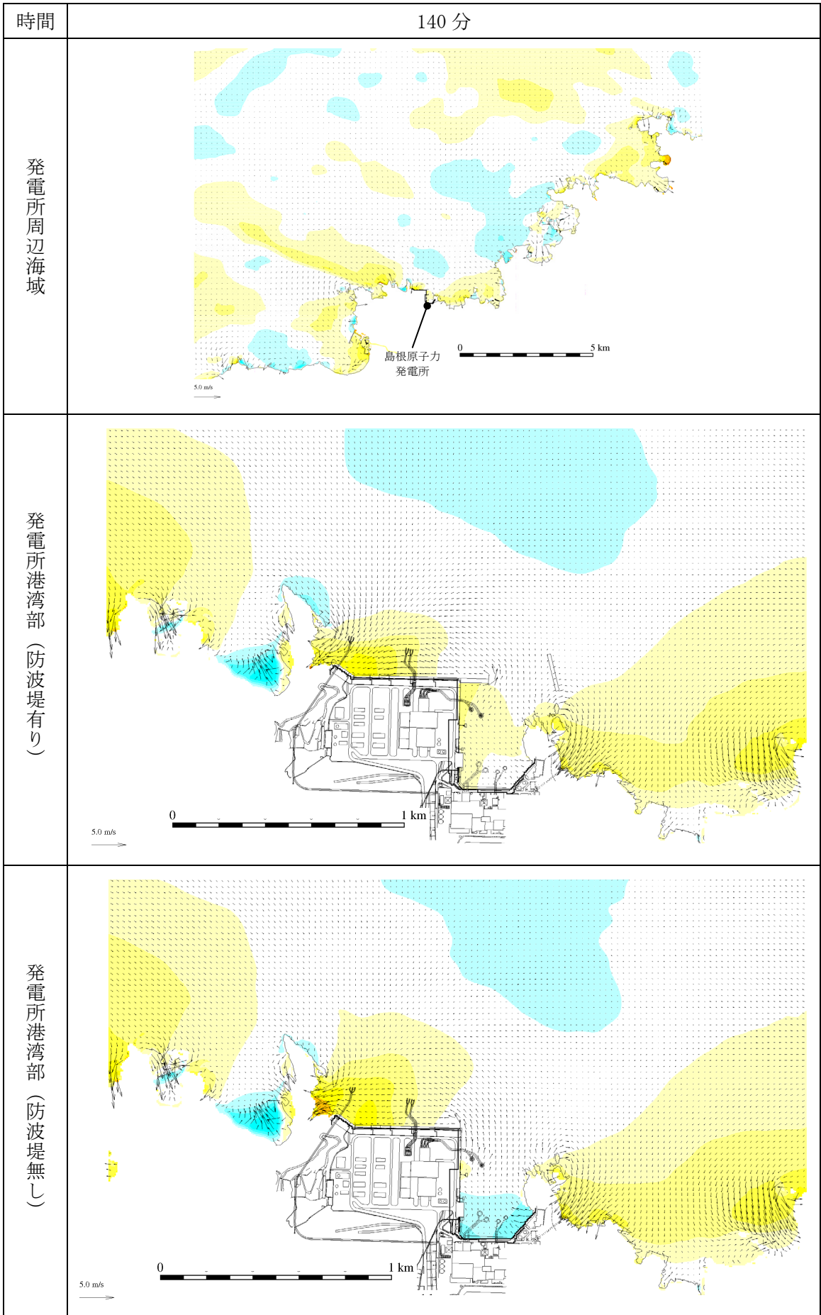
第 1 図(81) 基準津波 1 の水位変動・流向ベクトル
