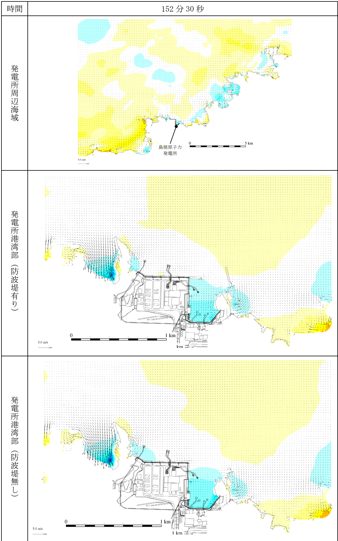
第 1 図 (106) 基準津波 1 の水位変動・流向ベクトル
