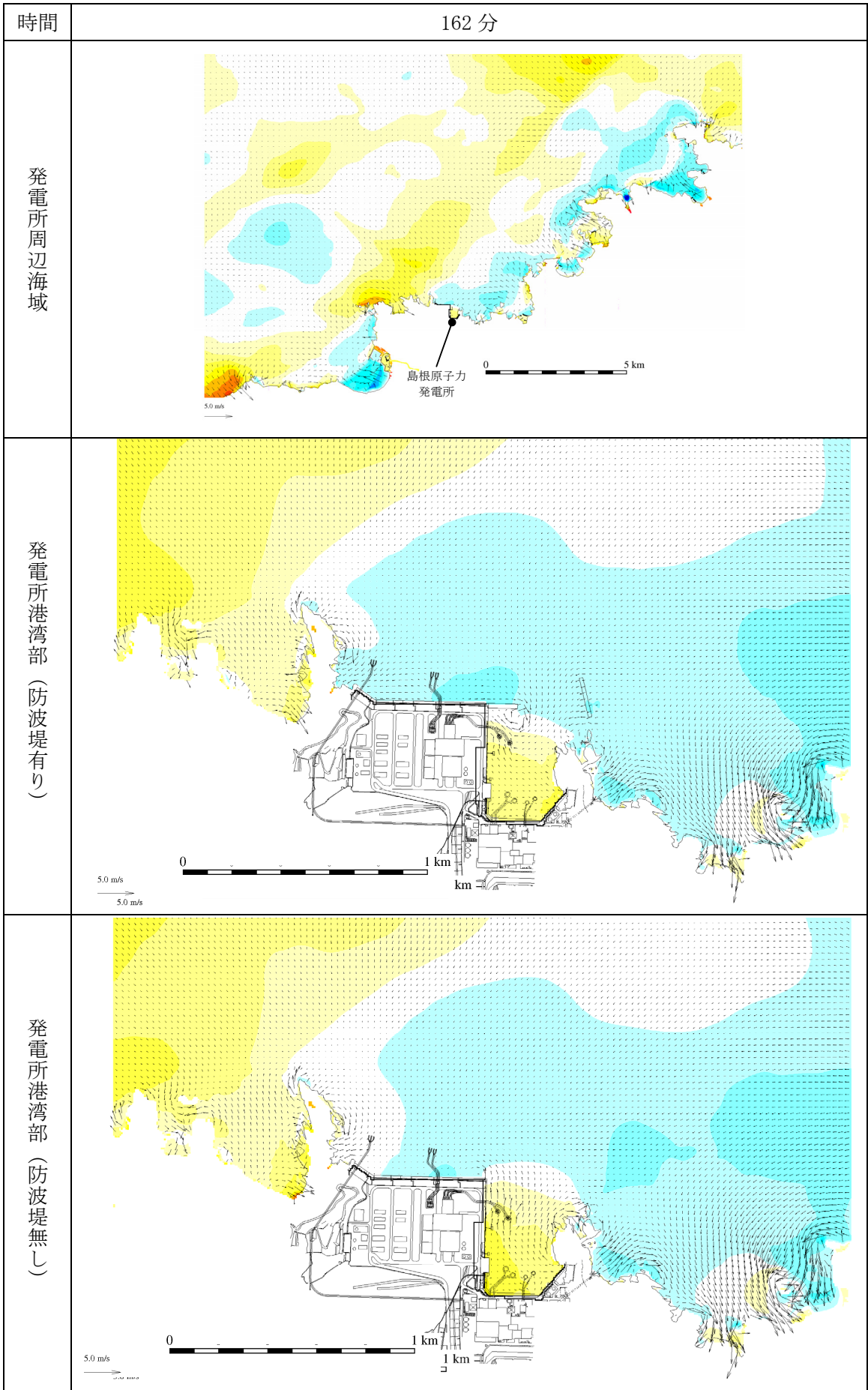
第 1 図 (125) 基準津波 1 の水位変動・流向ベクトル
