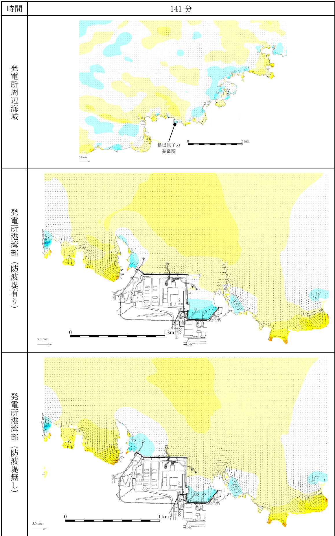
第 1 図(83) 基準津波 1 の水位変動・流向ベクトル
