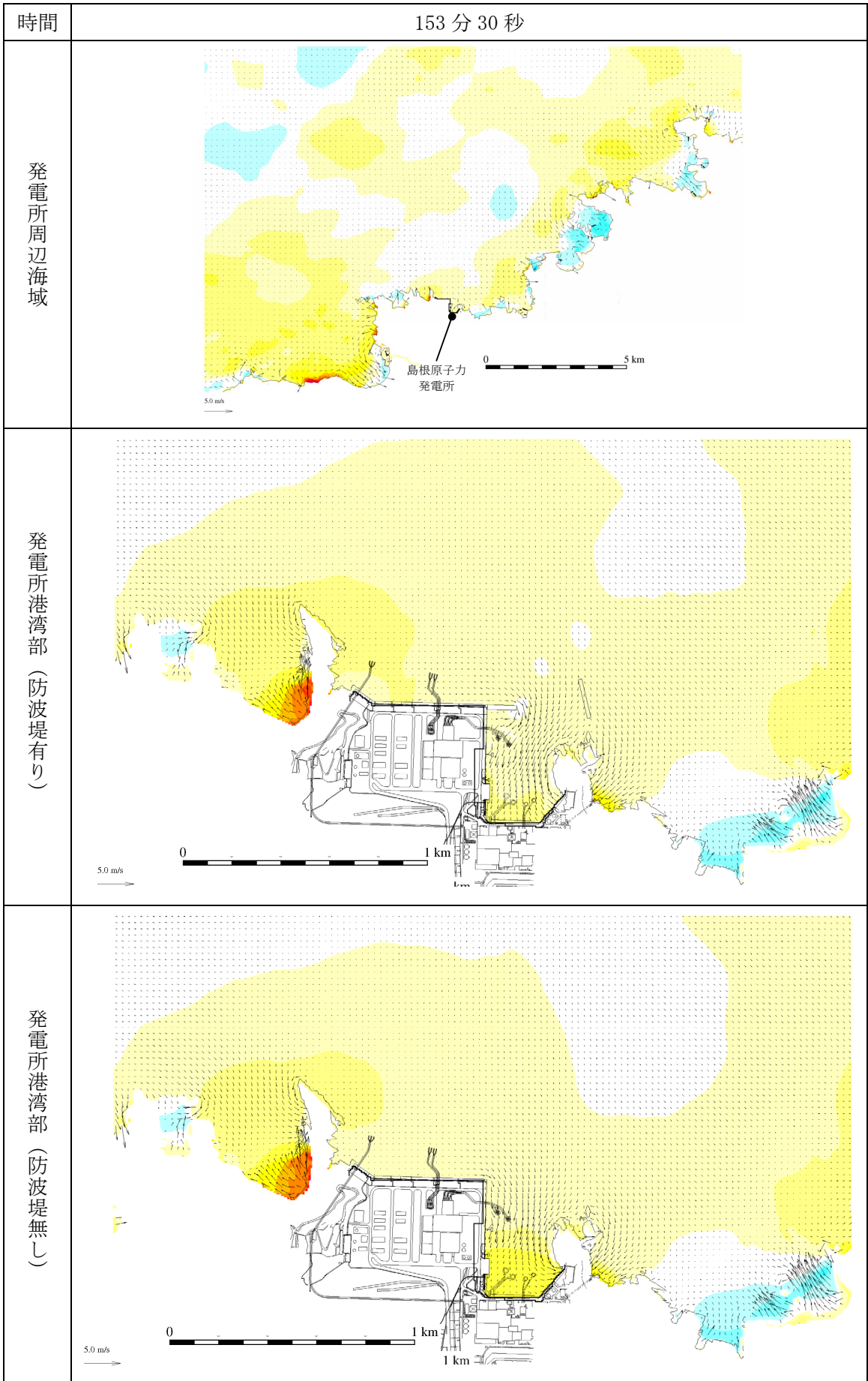
第 1 図 (108) 基準津波 1 の水位変動・流向ベクトル
