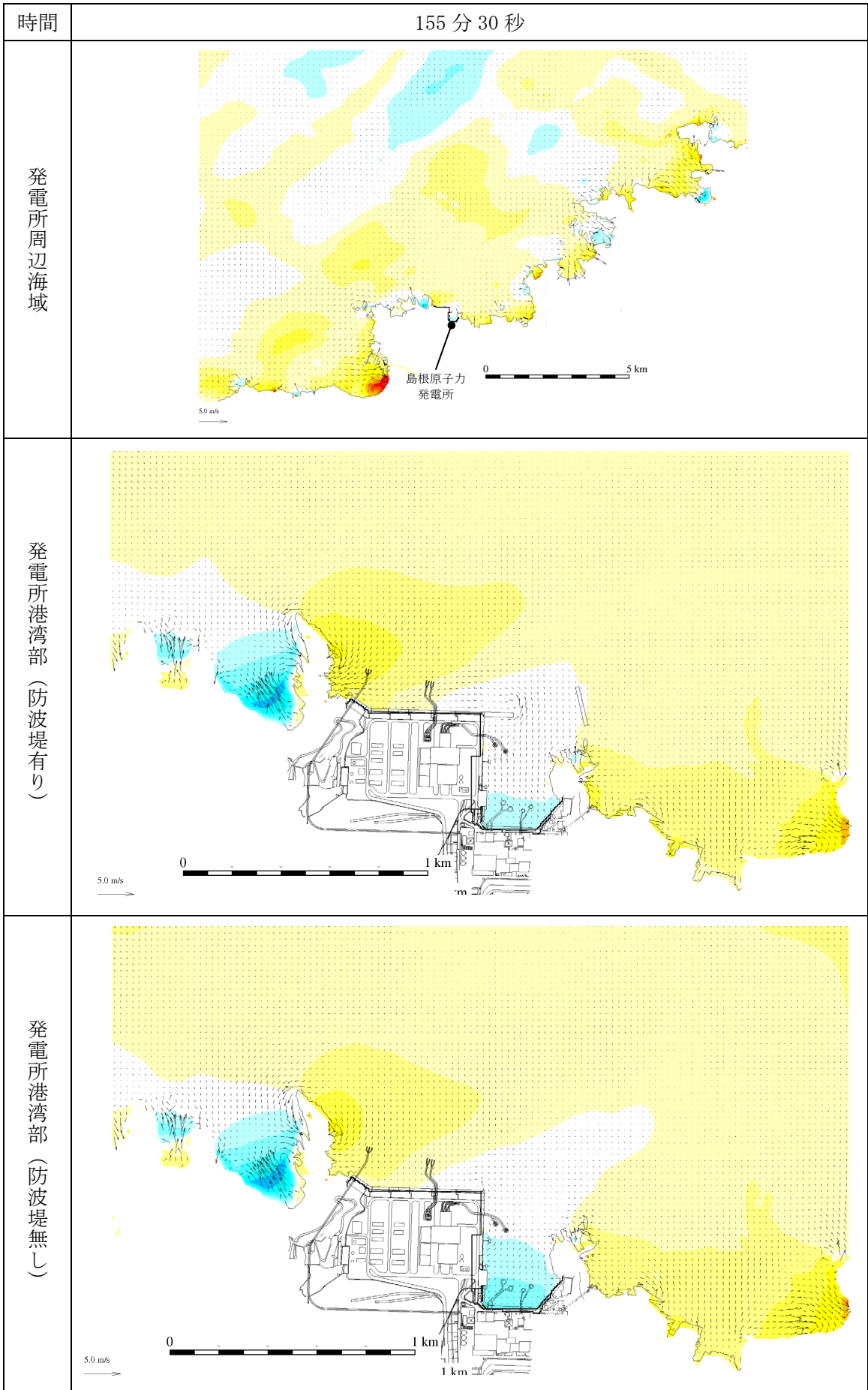
第 1 図 (112) 基準津波 1 の水位変動・流向ベクトル
