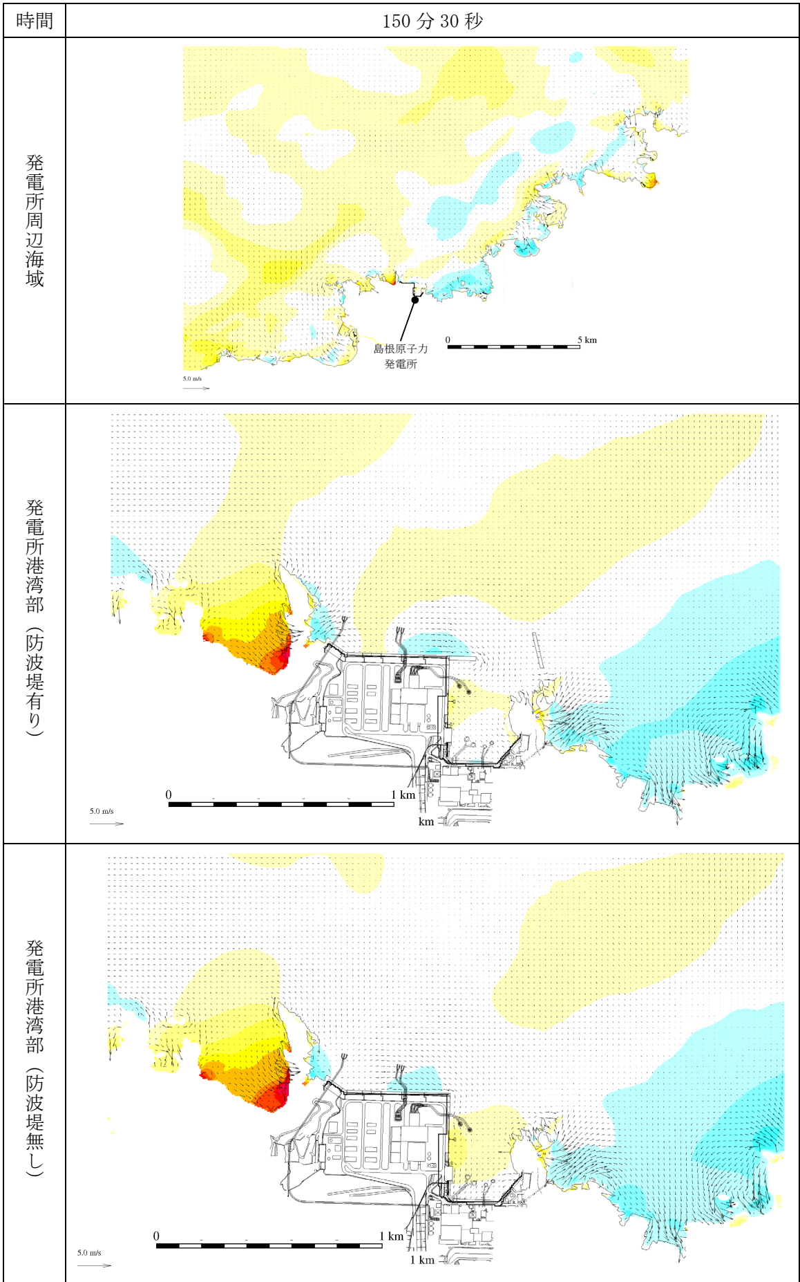
第 1 図 (102) 基準津波 1 の水位変動・流向ベクトル
