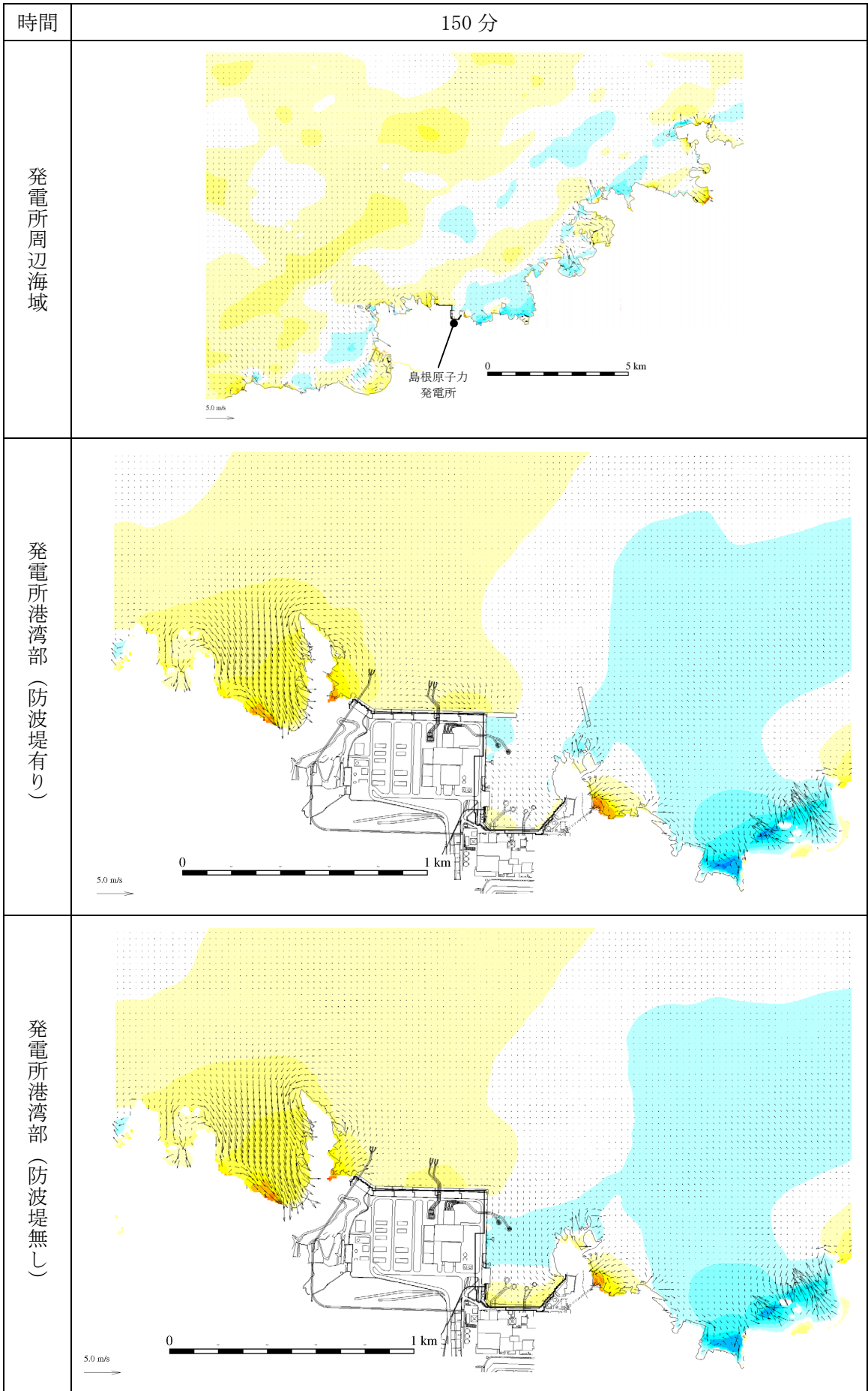
第 1 図 (101) 基準津波 1 の水位変動・流向ベクトル
