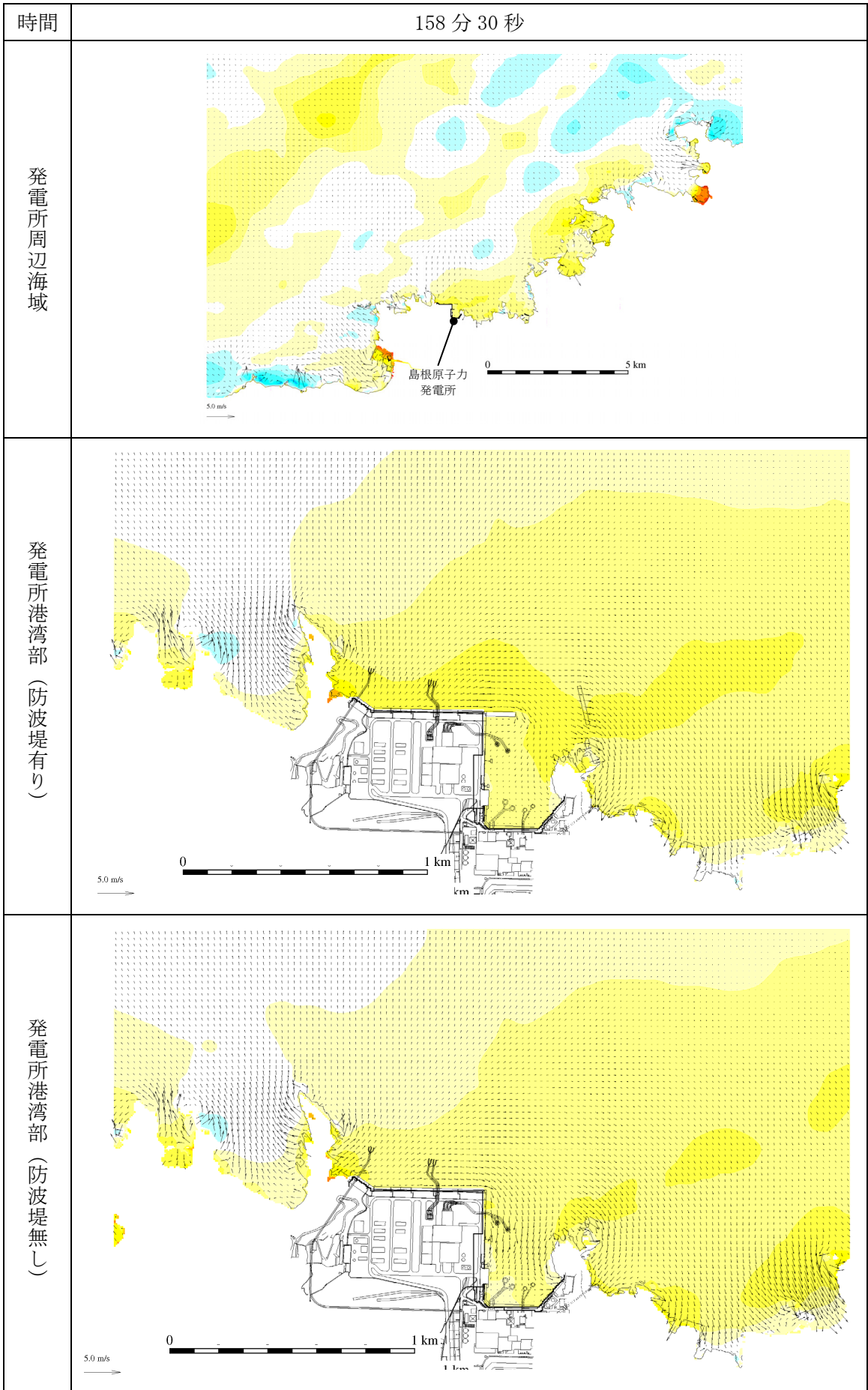
第 1 図 (118) 基準津波 1 の水位変動・流向ベクトル
