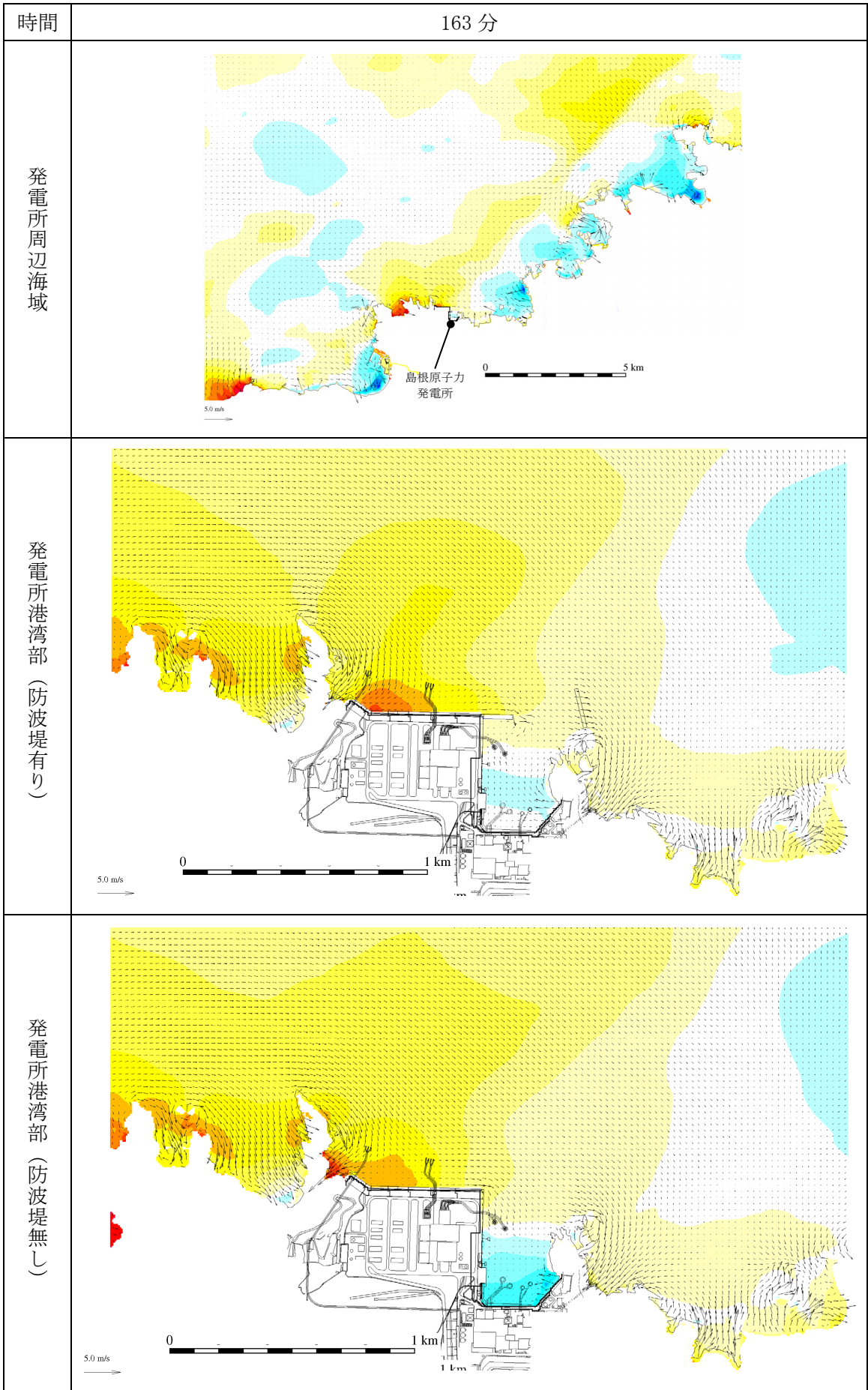
第 1 図 (127) 基準津波 1 の水位変動・流向ベクトル
