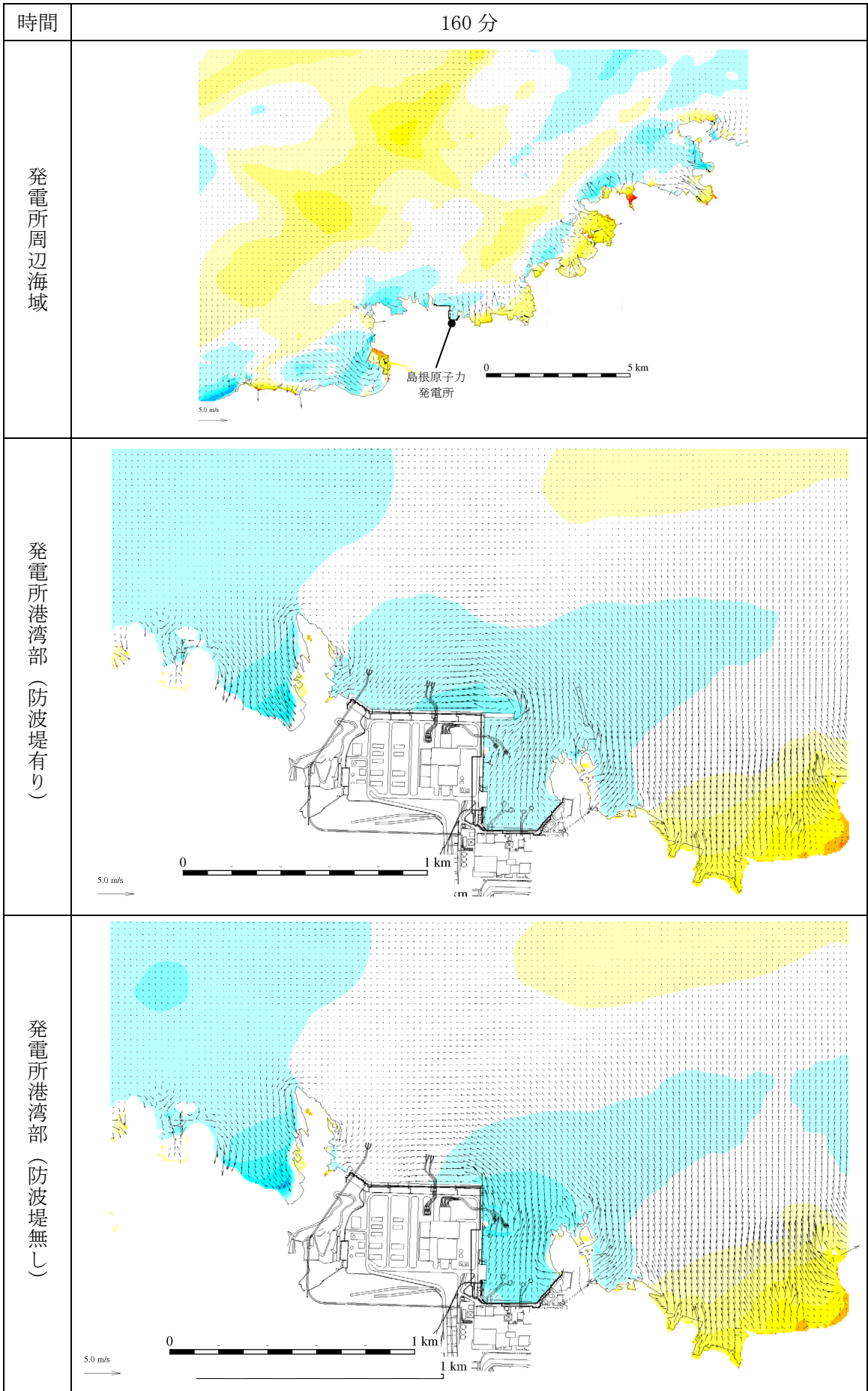
第 1 図 (121) 基準津波 1 の水位変動・流向ベクトル
