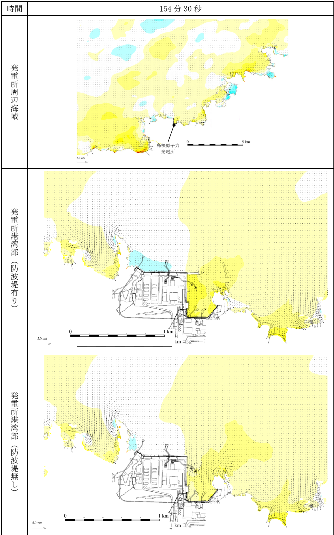
第 1 図 (110) 基準津波 1 の水位変動・流向ベクトル
