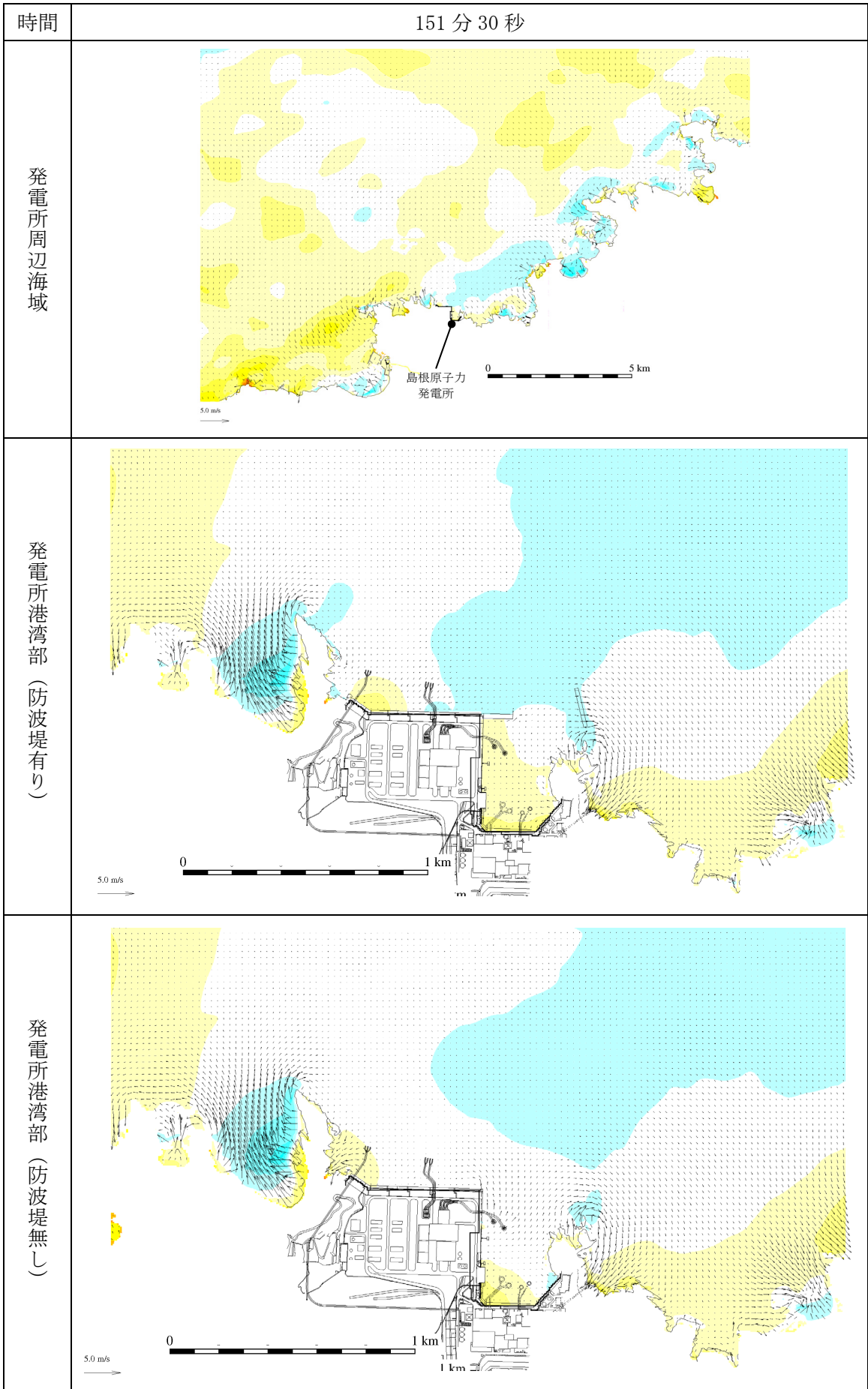
第 1 図 (104) 基準津波 1 の水位変動・流向ベクトル
