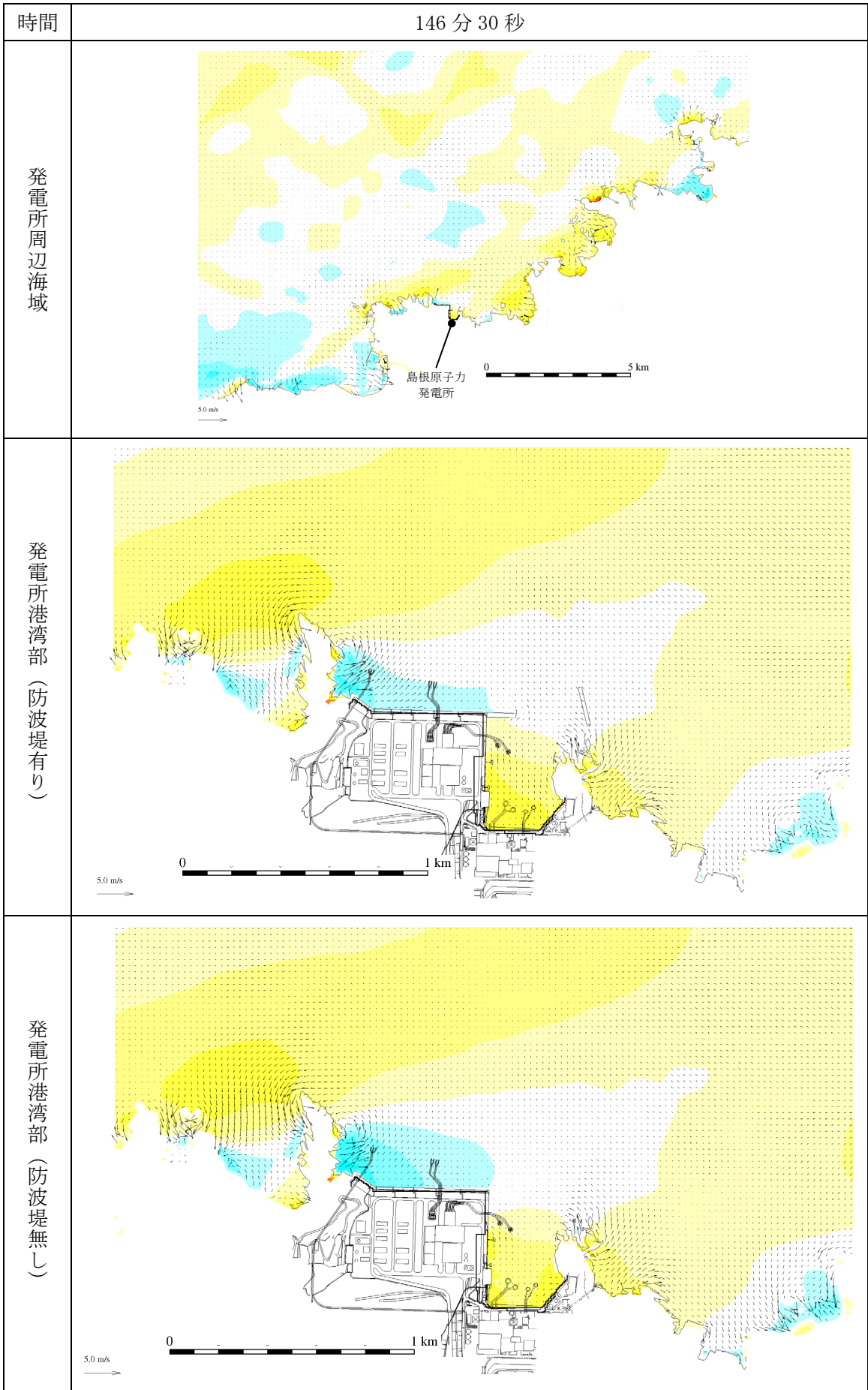
第 1 図(94) 基準津波 1 の水位変動・流向ベクトル
