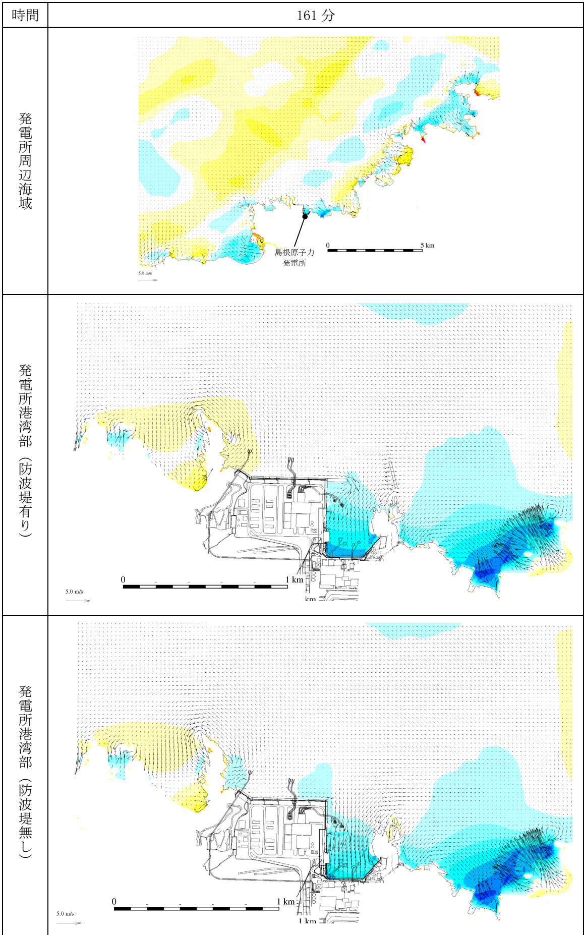
第 1 図 (123) 基準津波 1 の水位変動・流向ベクトル
