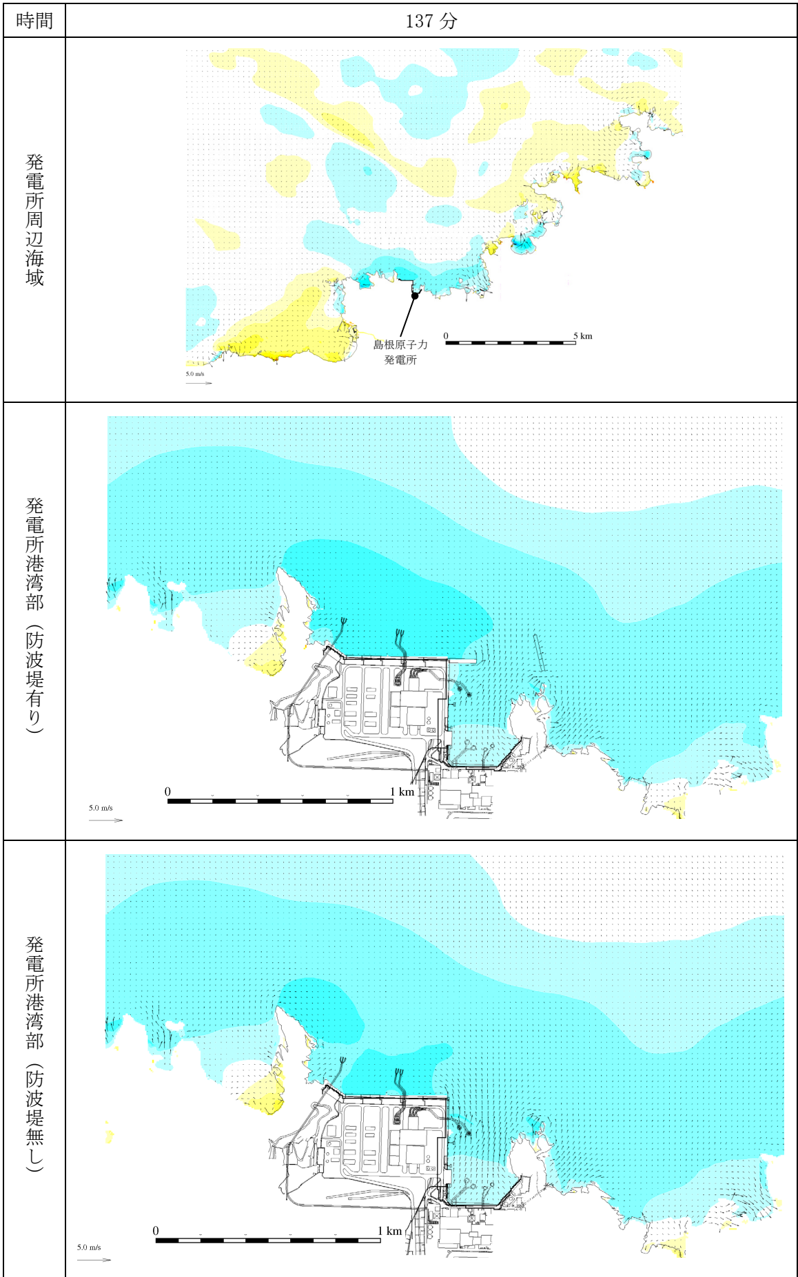
第 1 図(75) 基準津波 1 の水位変動・流向ベクトル
