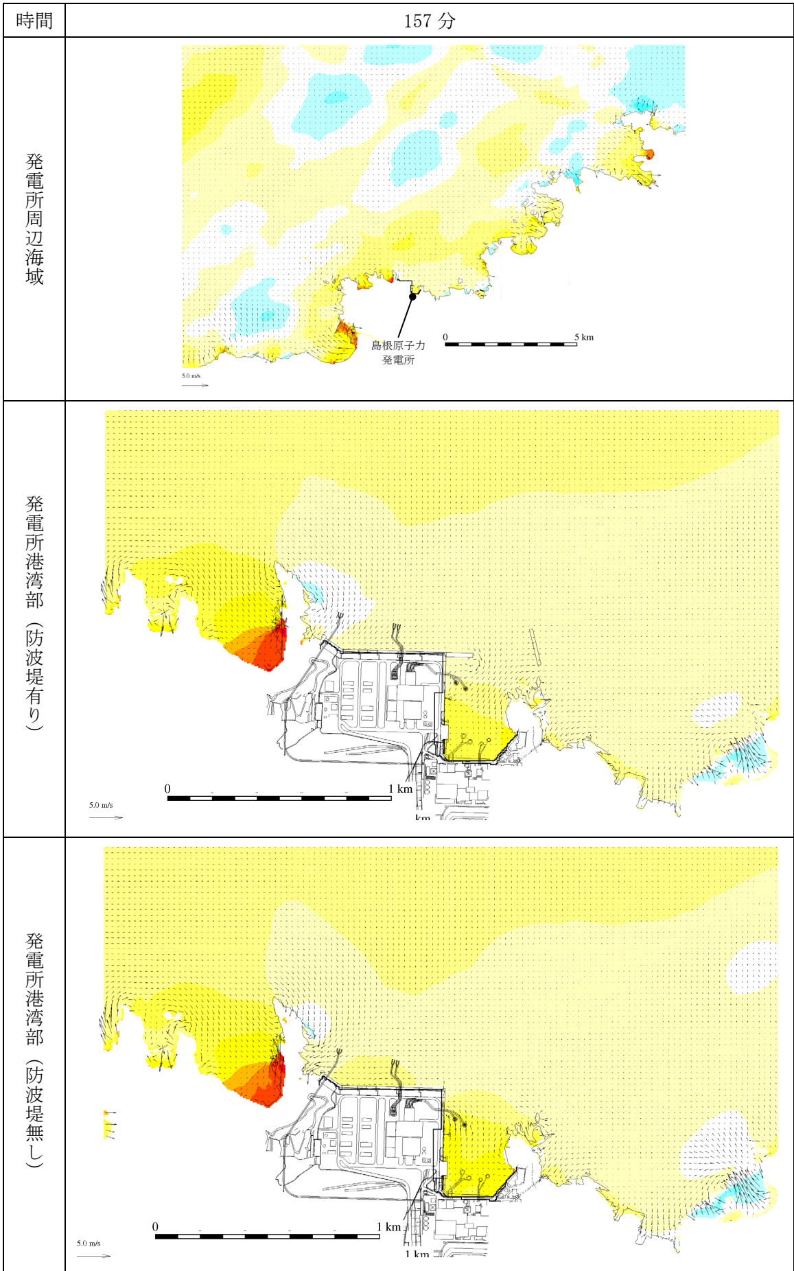
第 1 図 (115) 基準津波 1 の水位変動・流向ベクトル
