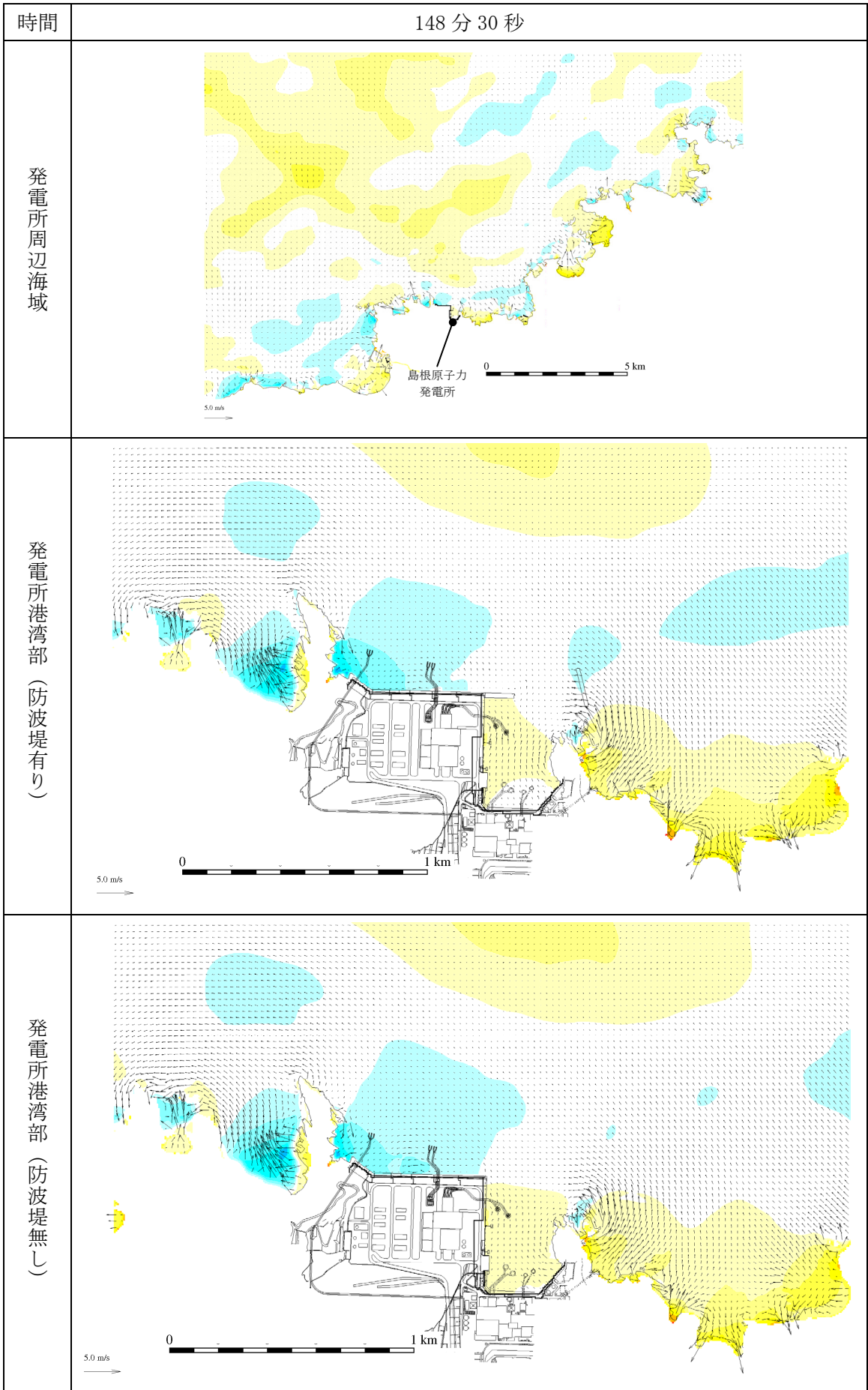
第 1 図(98) 基準津波 1 の水位変動・流向ベクトル
