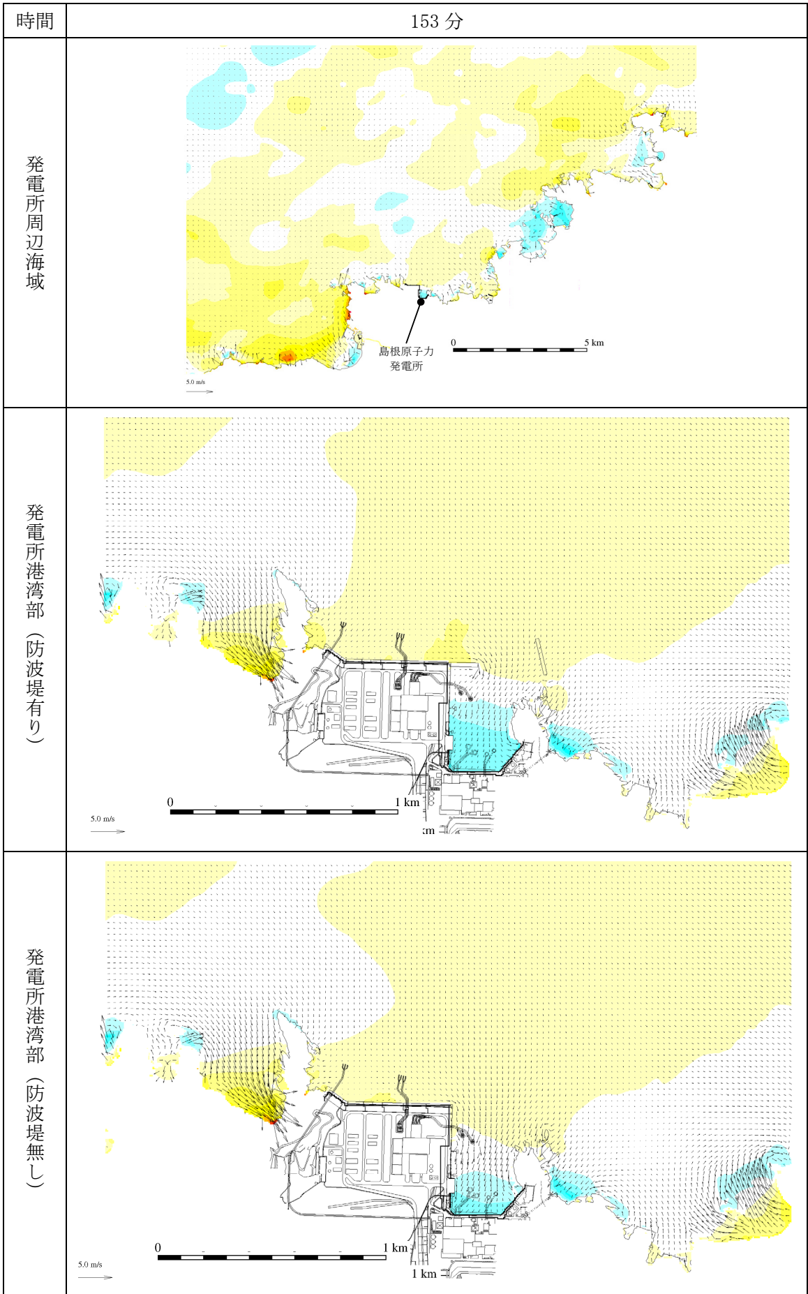
第 1 図 (107) 基準津波 1 の水位変動・流向ベクトル
