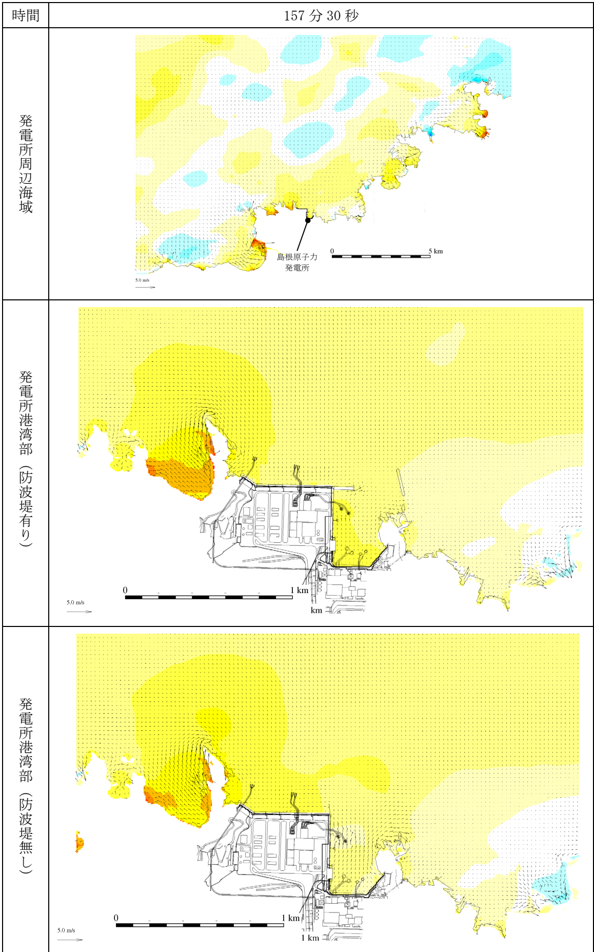
第 1 図 (116) 基準津波 1 の水位変動・流向ベクトル
