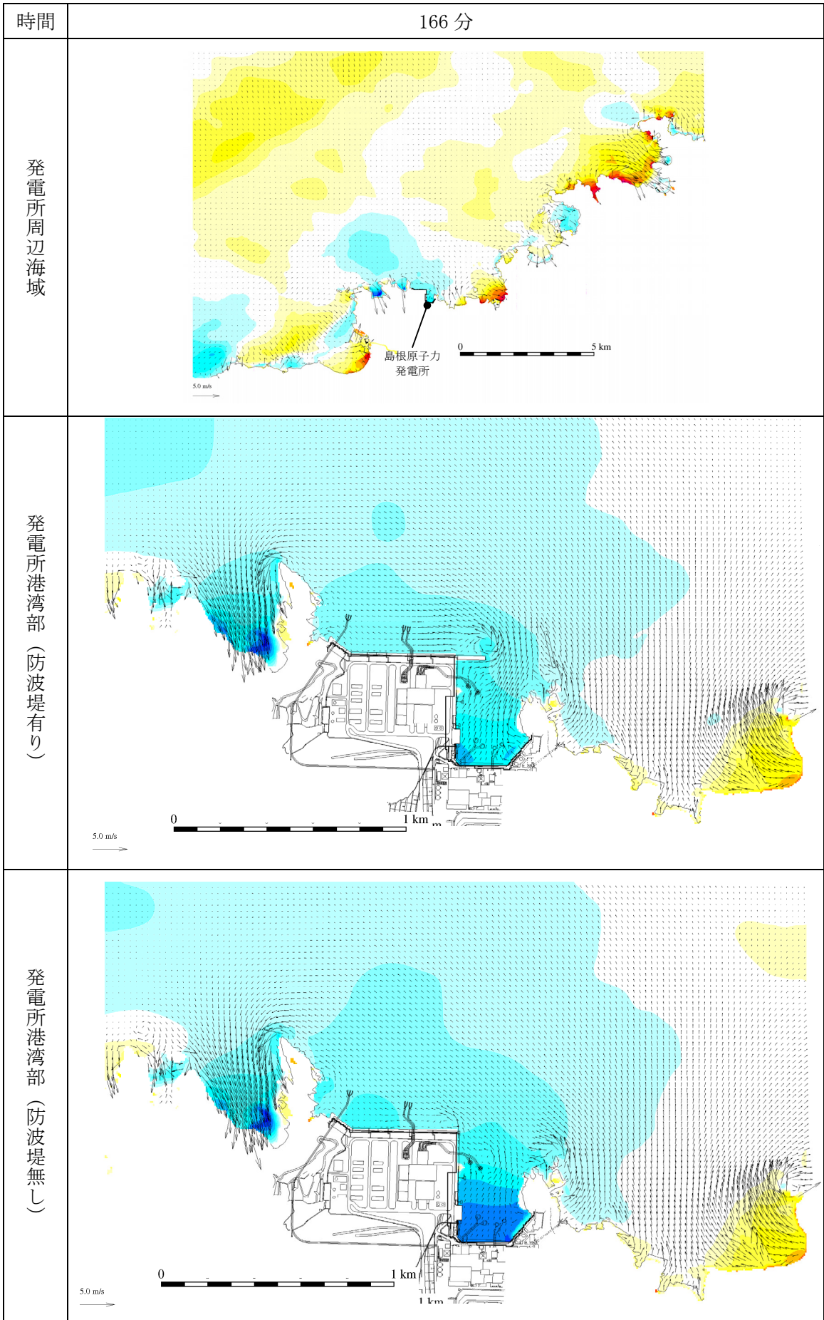
第 1 図 (133) 基準津波 1 の水位変動・流向ベクトル
