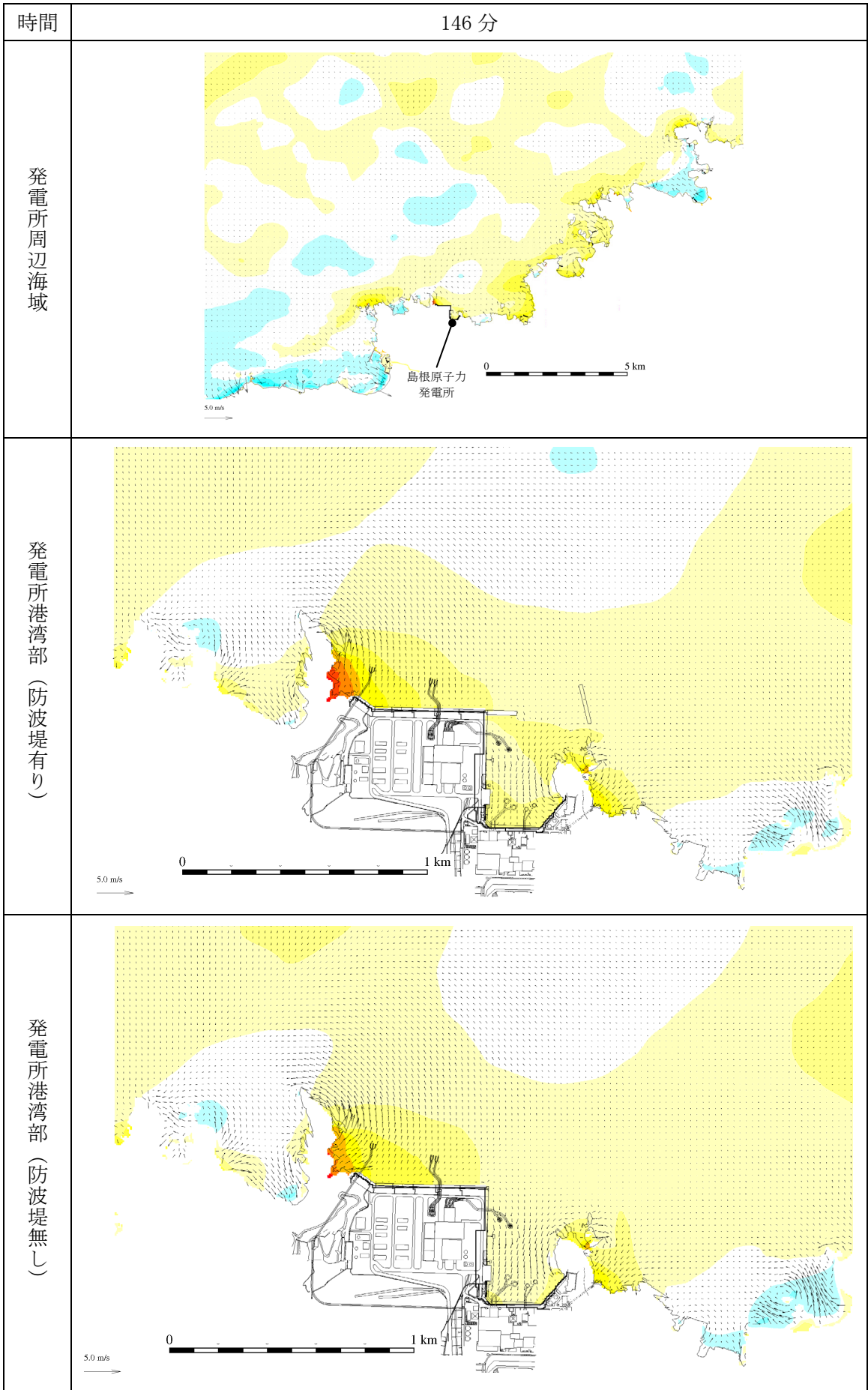
第 1 図(93) 基準津波 1 の水位変動・流向ベクトル
