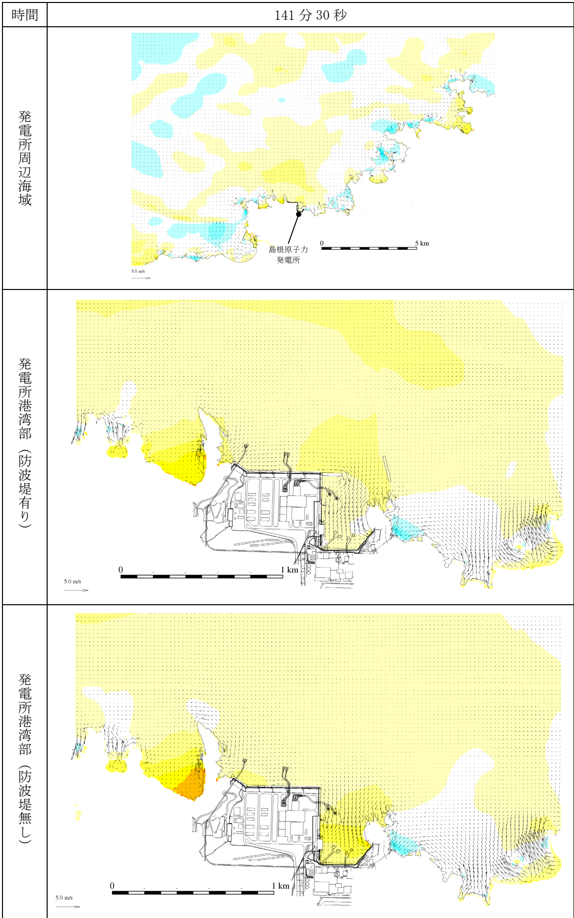
第 1 図(84) 基準津波 1 の水位変動・流向ベクトル
