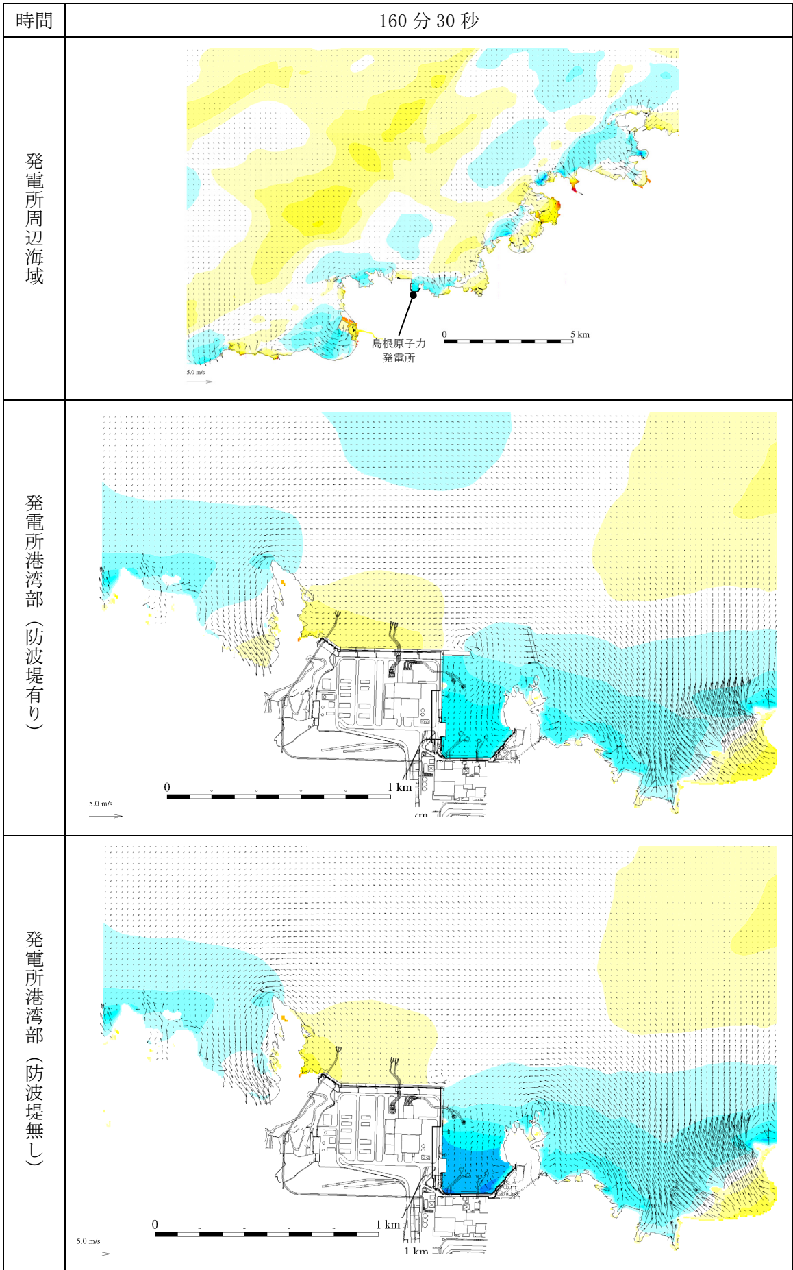
第 1 図 (122) 基準津波 1 の水位変動・流向ベクトル
