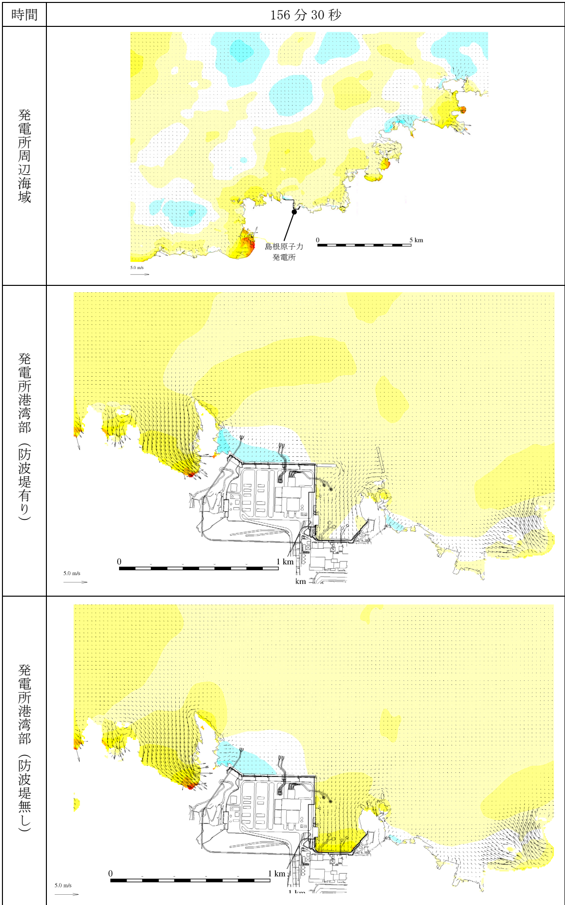
第 1 図 (114) 基準津波 1 の水位変動・流向ベクトル
