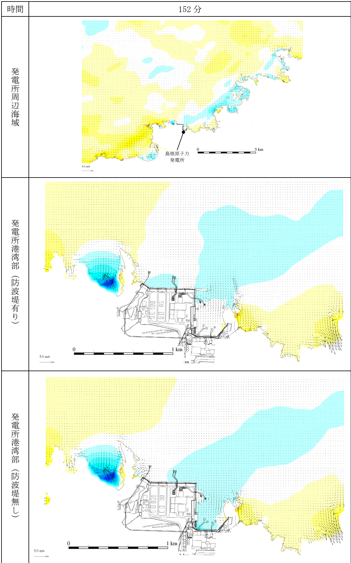
第 1 図 (105) 基準津波 1 の水位変動・流向ベクトル
