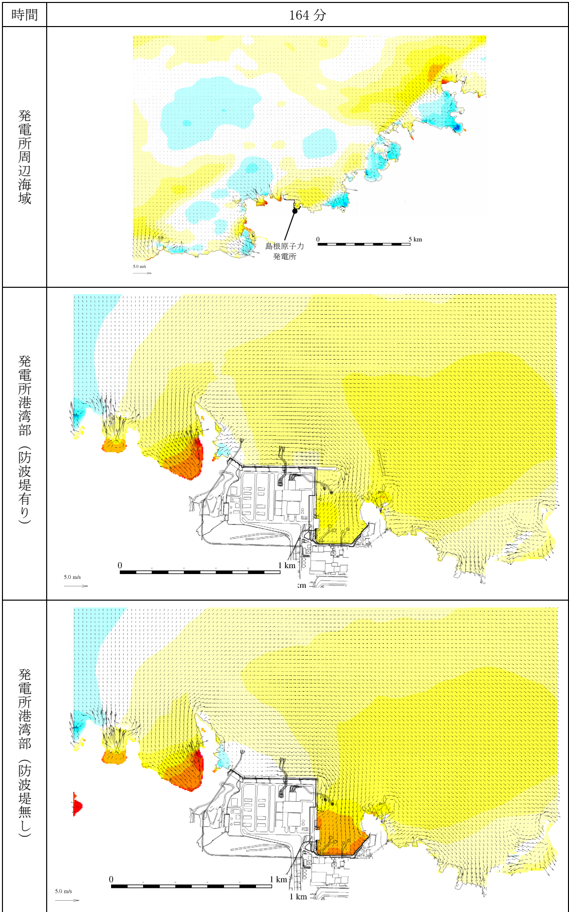
第 1 図 (129) 基準津波 1 の水位変動・流向ベクトル
