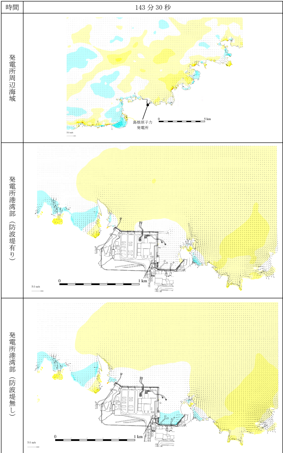
第 1 図(88) 基準津波 1 の水位変動・流向ベクトル
