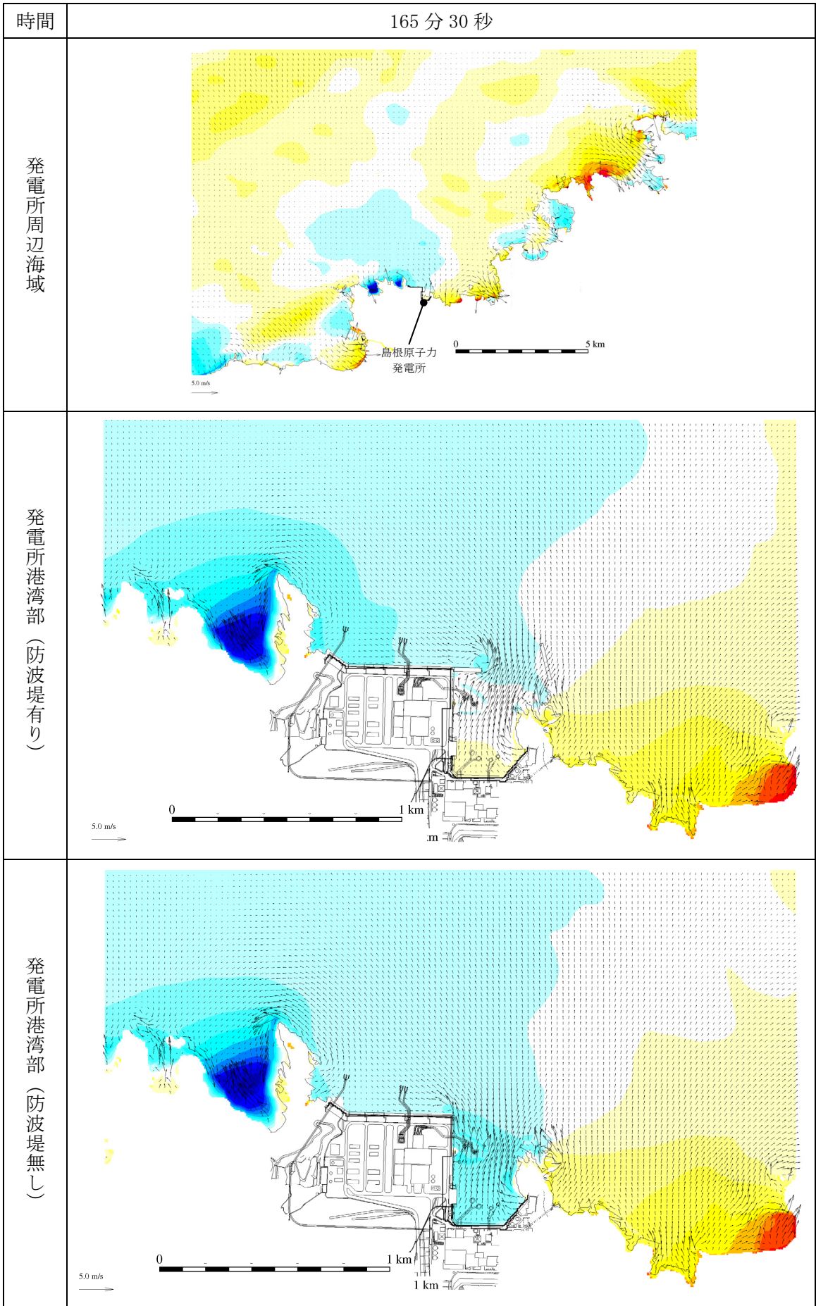
第 1 図 (132) 基準津波 1 の水位変動・流向ベクトル
