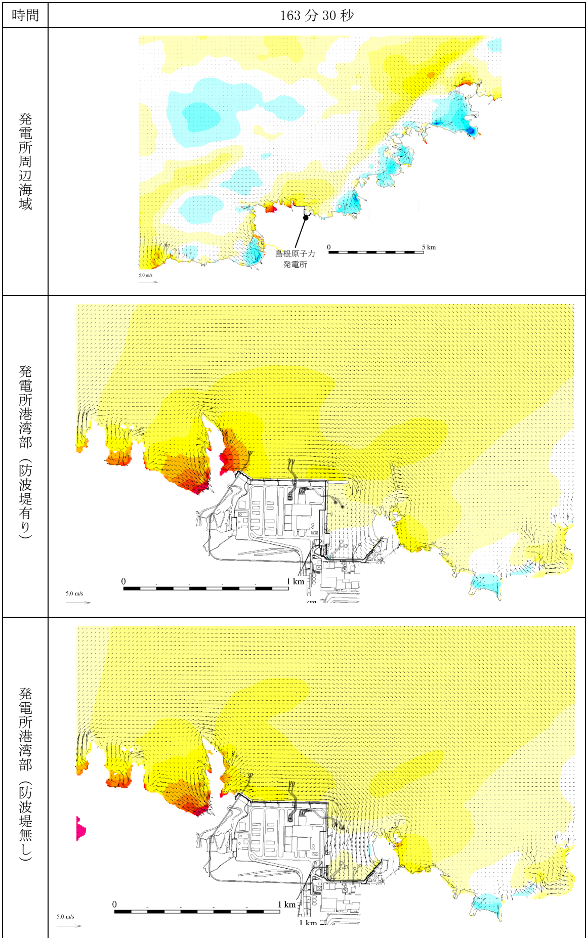
第 1 図 (128) 基準津波 1 の水位変動・流向ベクトル
