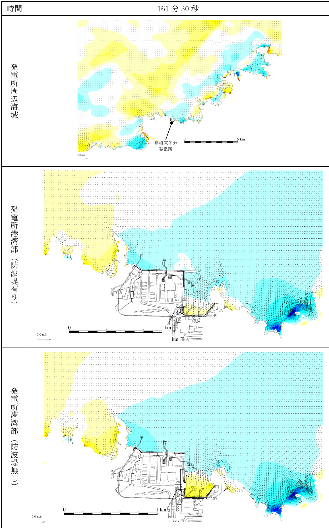
第 1 図 (124) 基準津波 1 の水位変動・流向ベクトル
