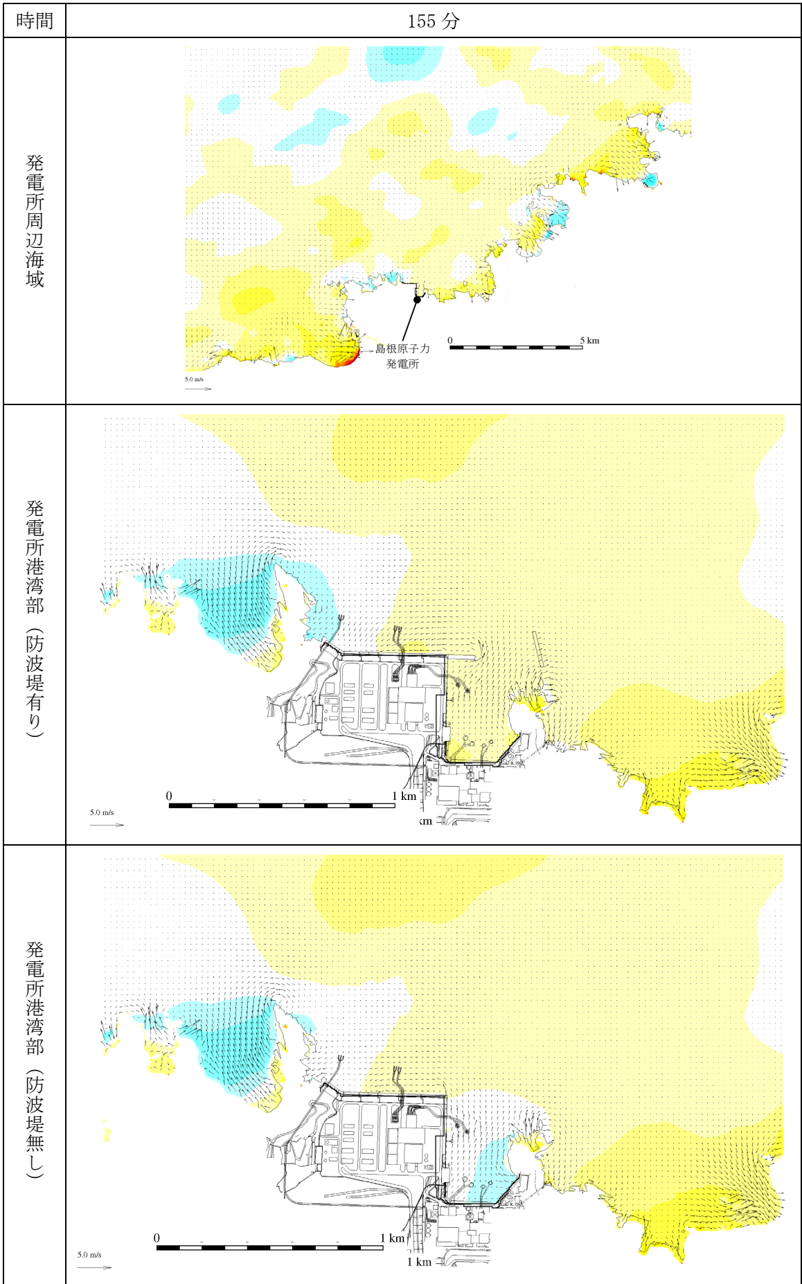
第 1 図 (111) 基準津波 1 の水位変動・流向ベクトル
