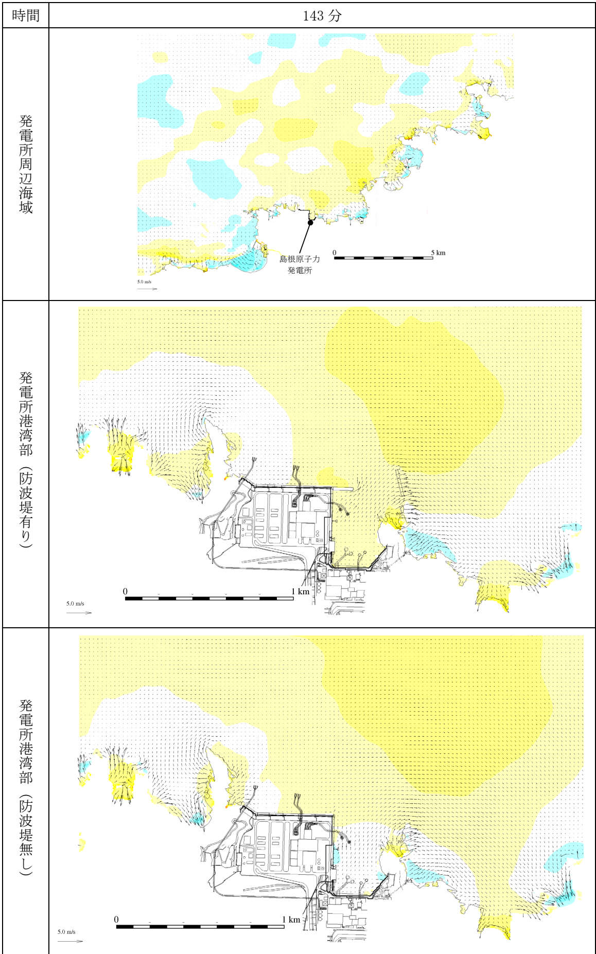
第 1 図(87) 基準津波 1 の水位変動・流向ベクトル
