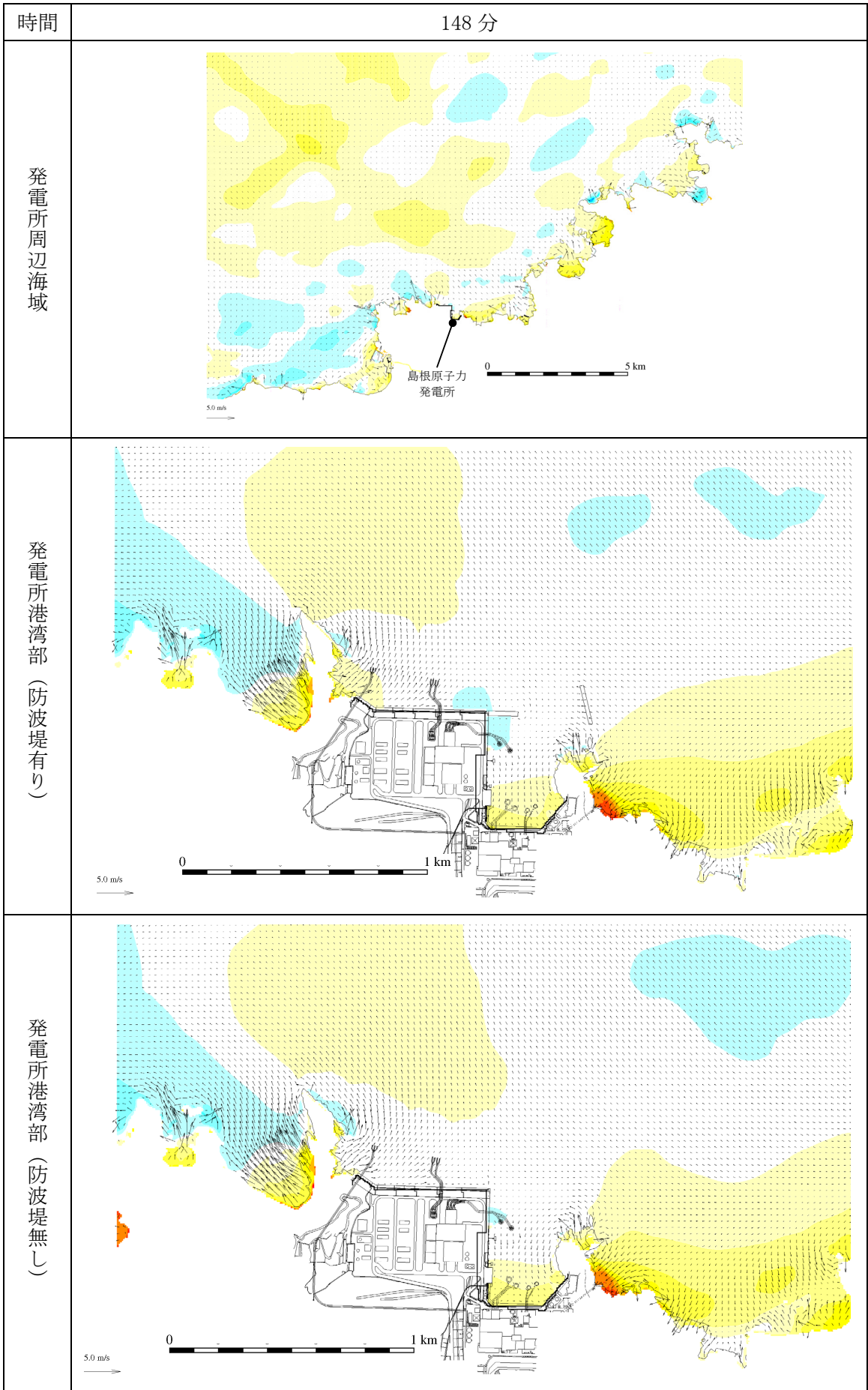
第 1 図(97) 基準津波 1 の水位変動・流向ベクトル
