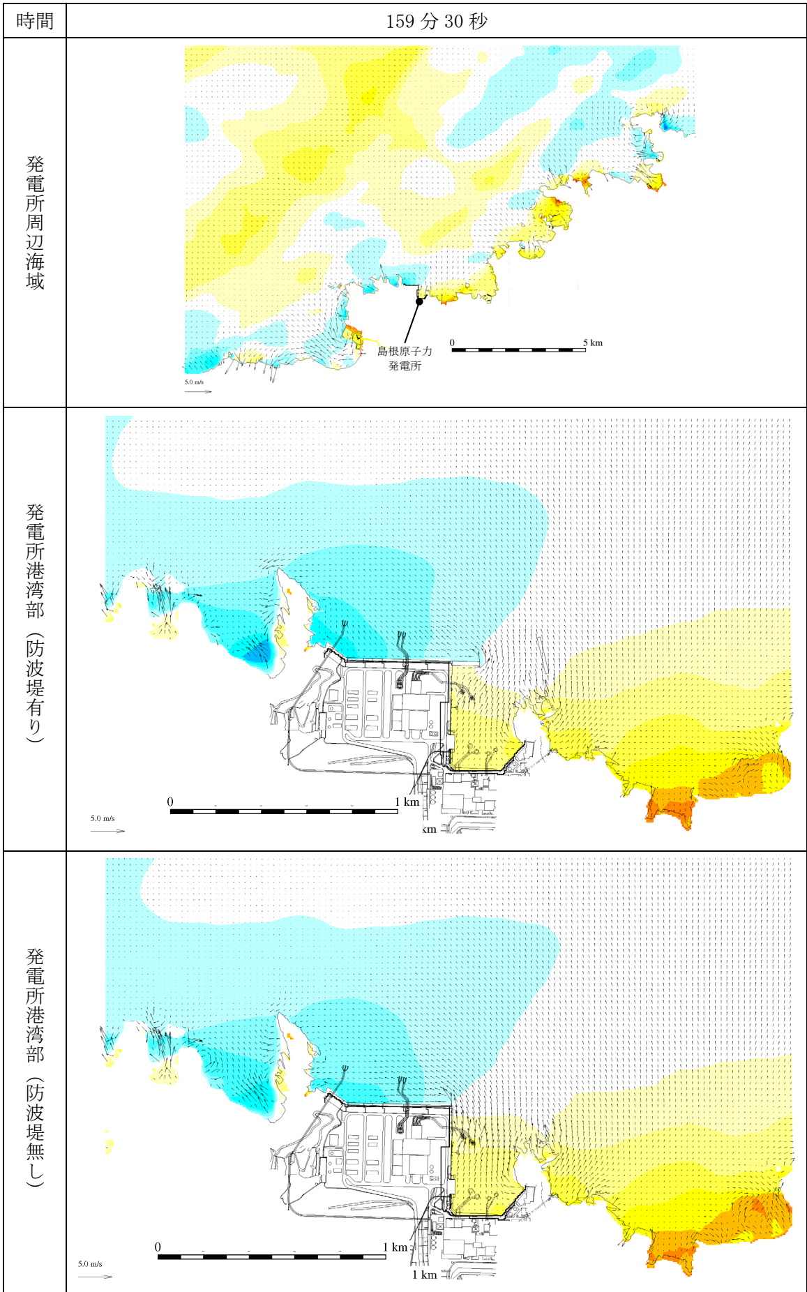
第 1 図 (120) 基準津波 1 の水位変動・流向ベクトル
