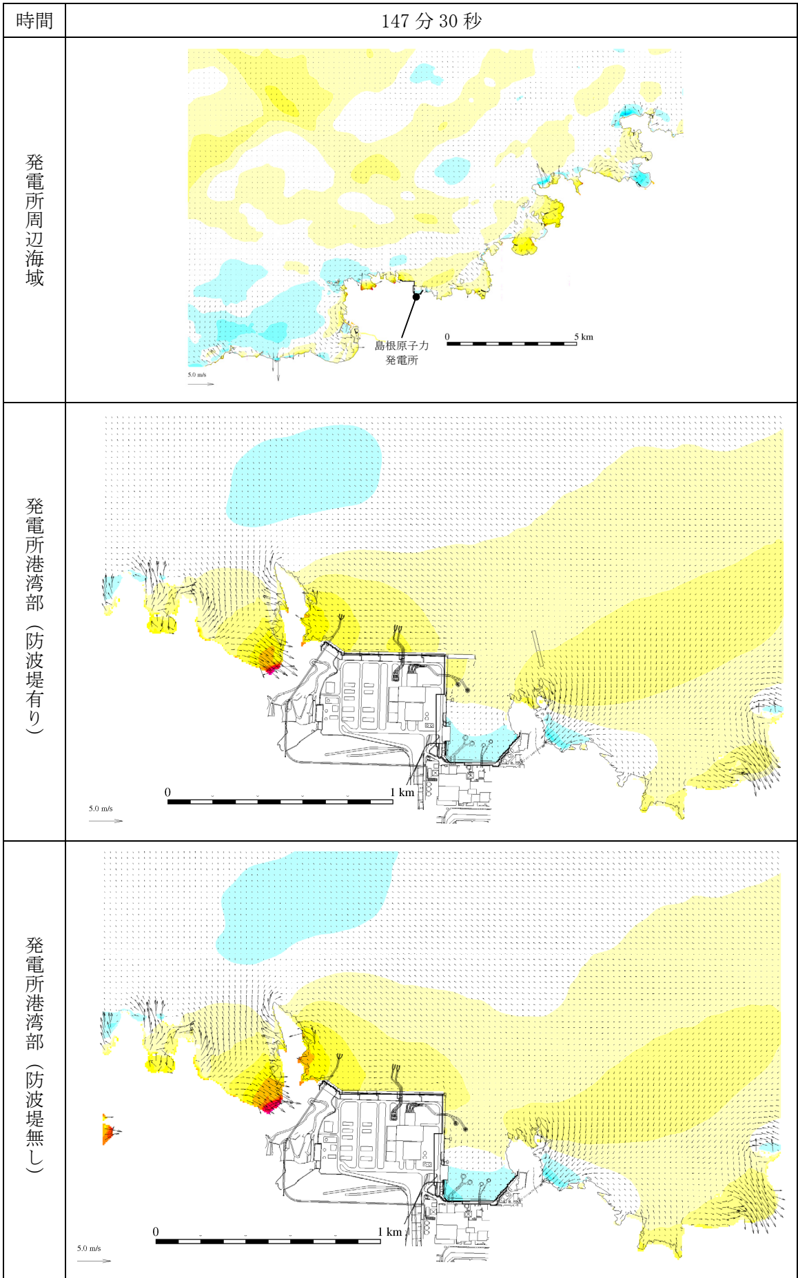
第 1 図(96) 基準津波 1 の水位変動・流向ベクトル
