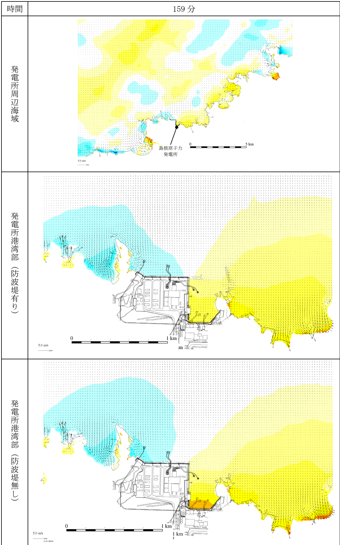
第 1 図 (119) 基準津波 1 の水位変動・流向ベクトル
