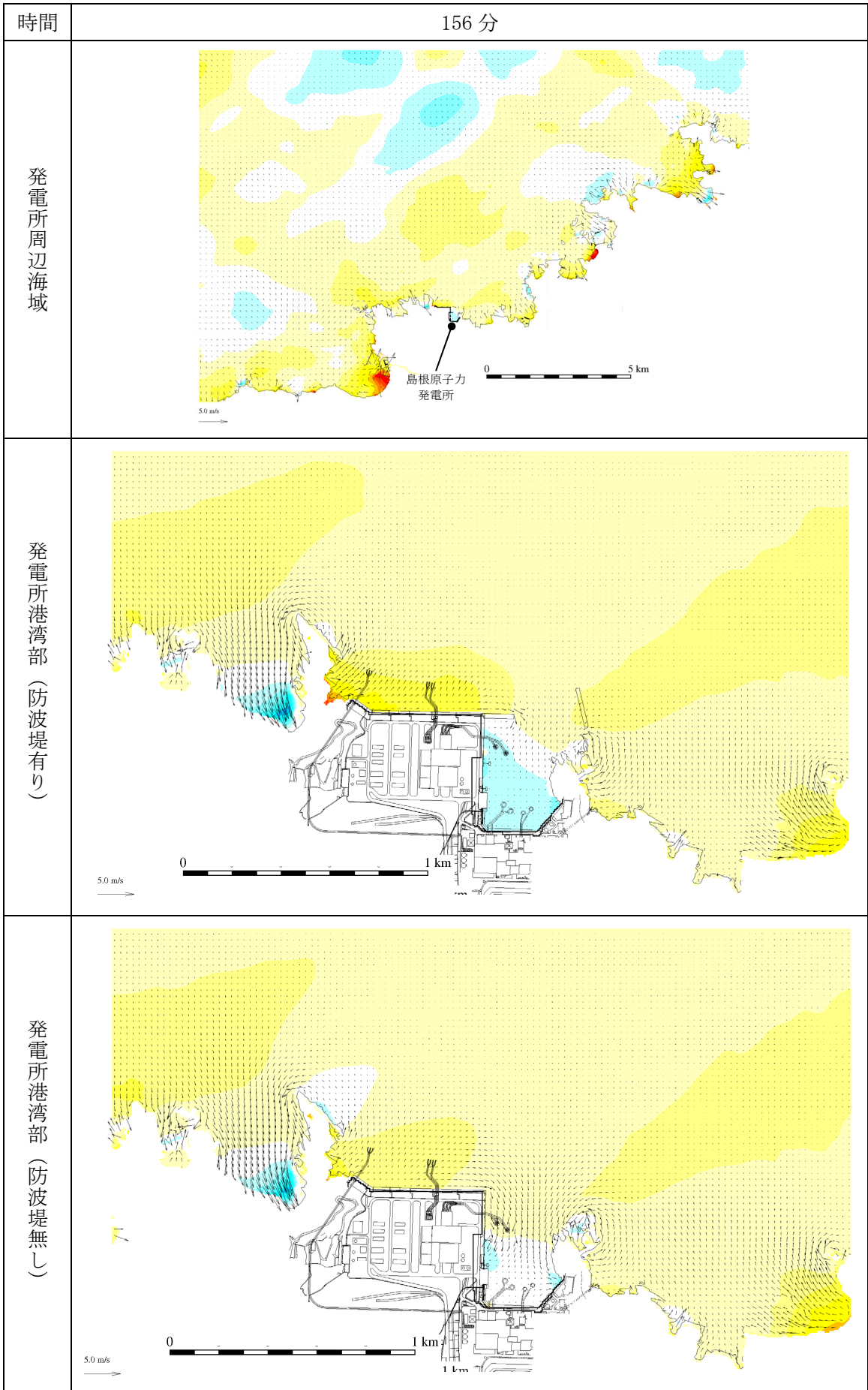
第 1 図 (113) 基準津波 1 の水位変動・流向ベクトル
