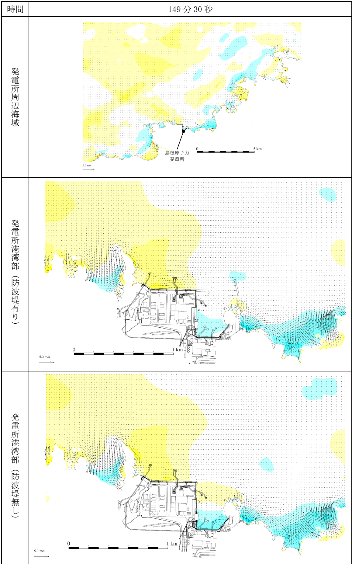
第 1 図 (100) 基準津波 1 の水位変動・流向ベクトル
