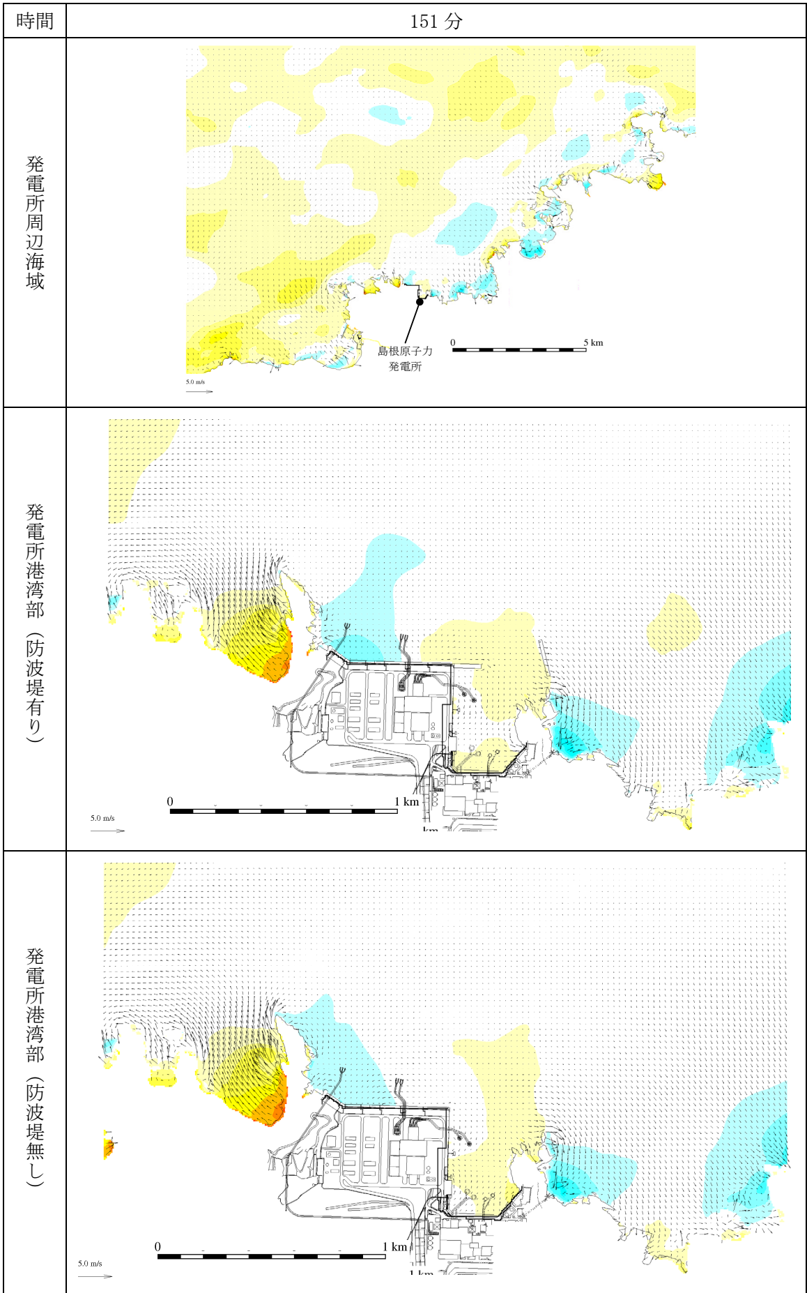
第 1 図 (103) 基準津波 1 の水位変動・流向ベクトル
