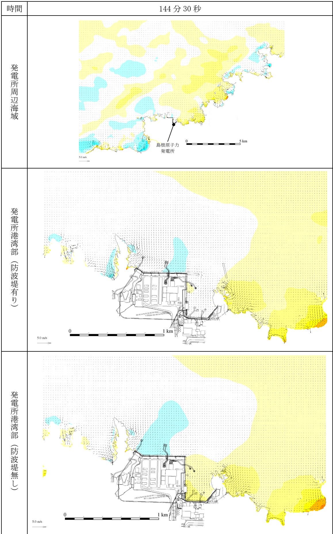
第 1 図(90) 基準津波 1 の水位変動・流向ベクトル
