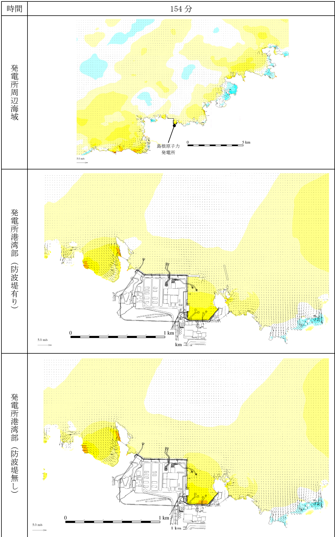
第 1 図 (109) 基準津波 1 の水位変動・流向ベクトル
