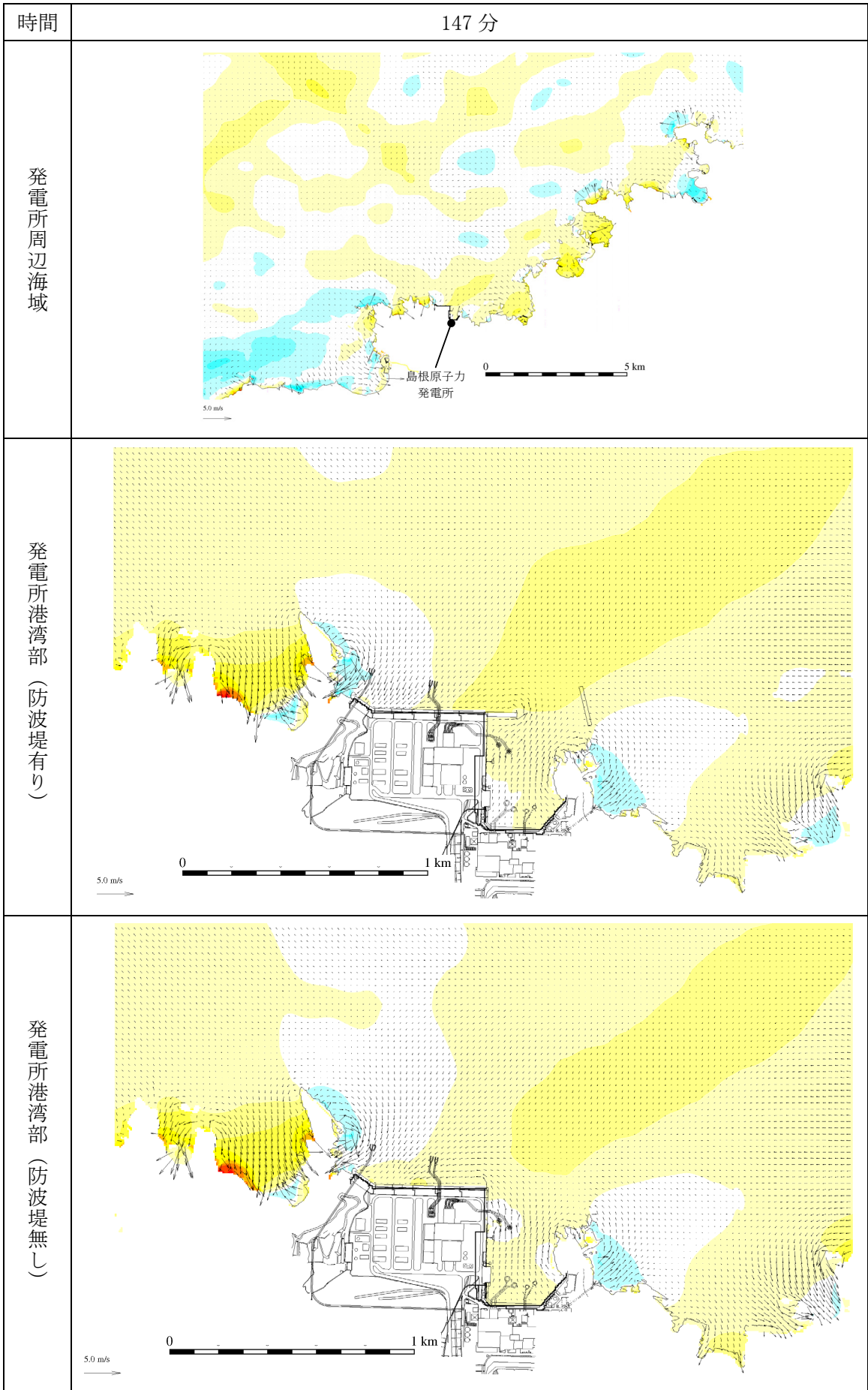
第 1 図(95) 基準津波 1 の水位変動・流向ベクトル
