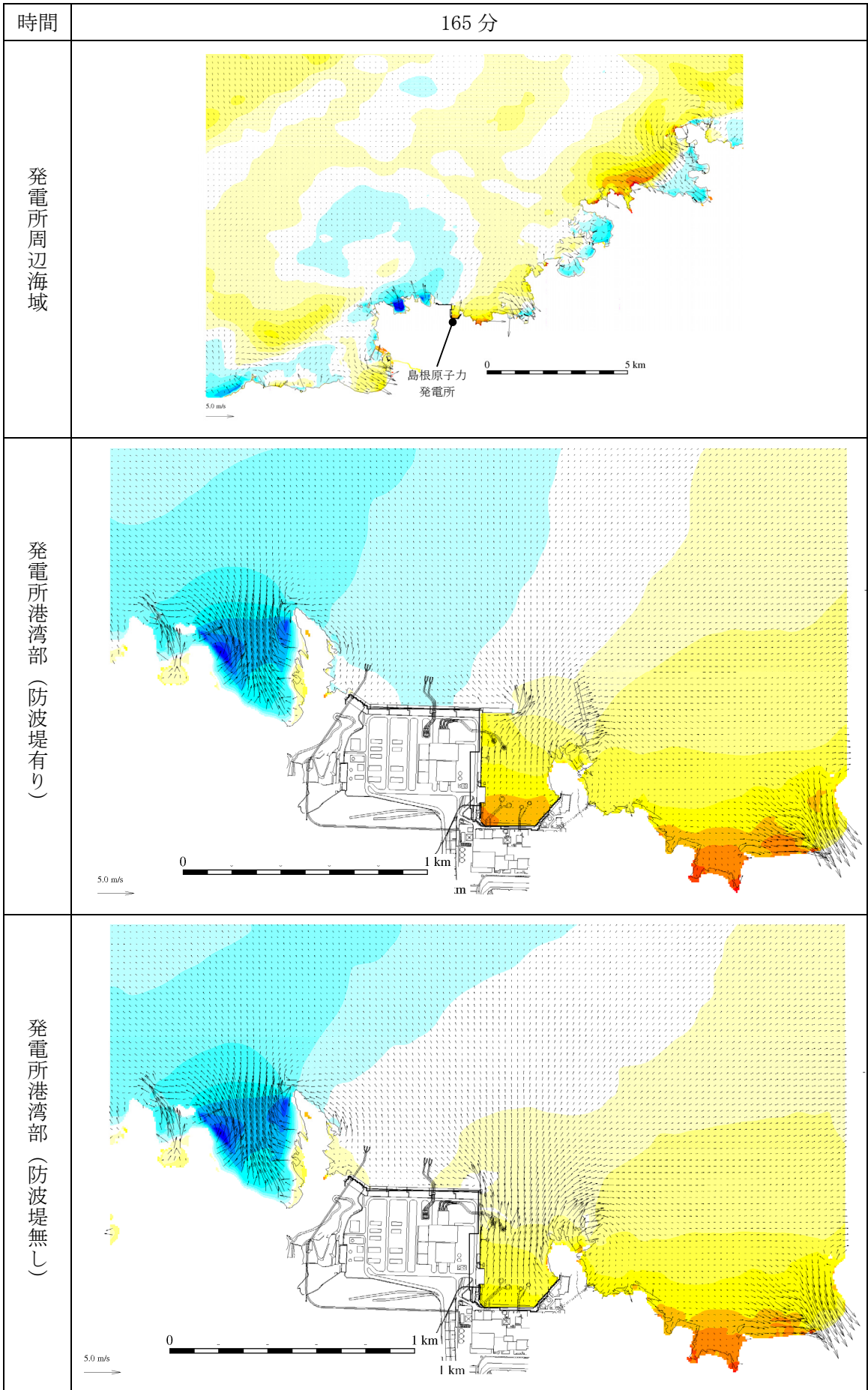
第 1 図 (131) 基準津波 1 の水位変動・流向ベクトル
