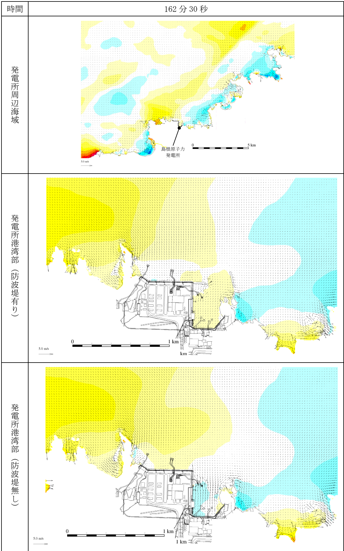
第 1 図 (126) 基準津波 1 の水位変動・流向ベクトル
