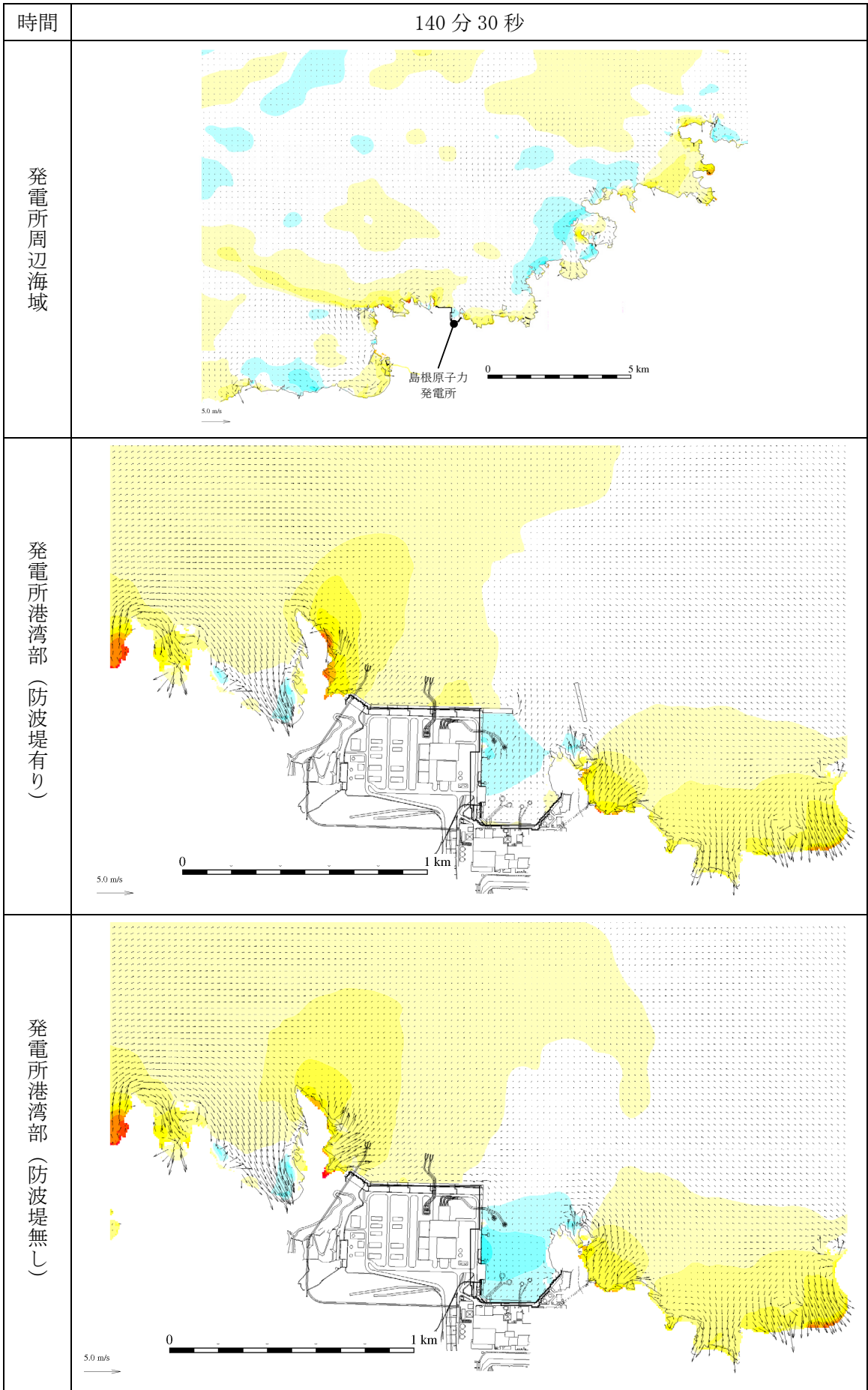
第 1 図(82) 基準津波 1 の水位変動・流向ベクトル
