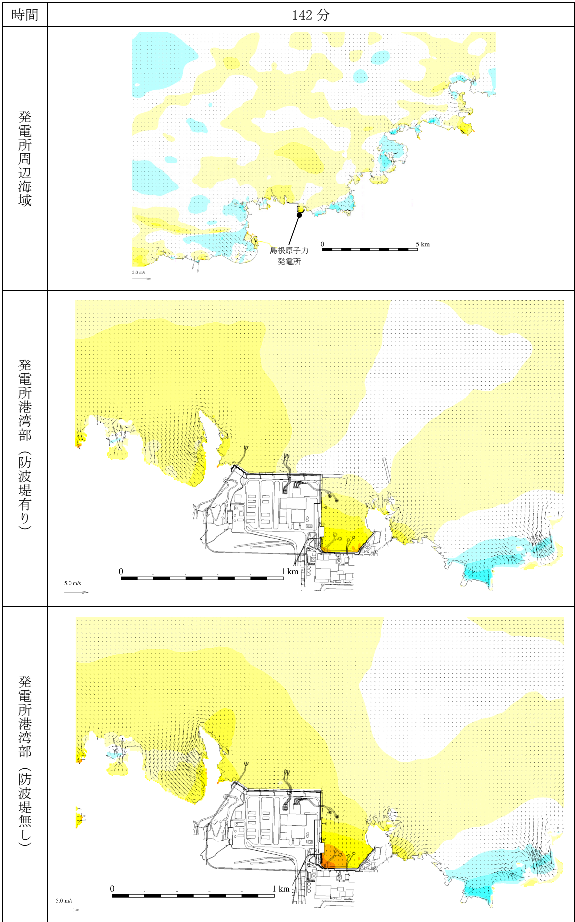
第 1 図(85) 基準津波 1 の水位変動・流向ベクトル
