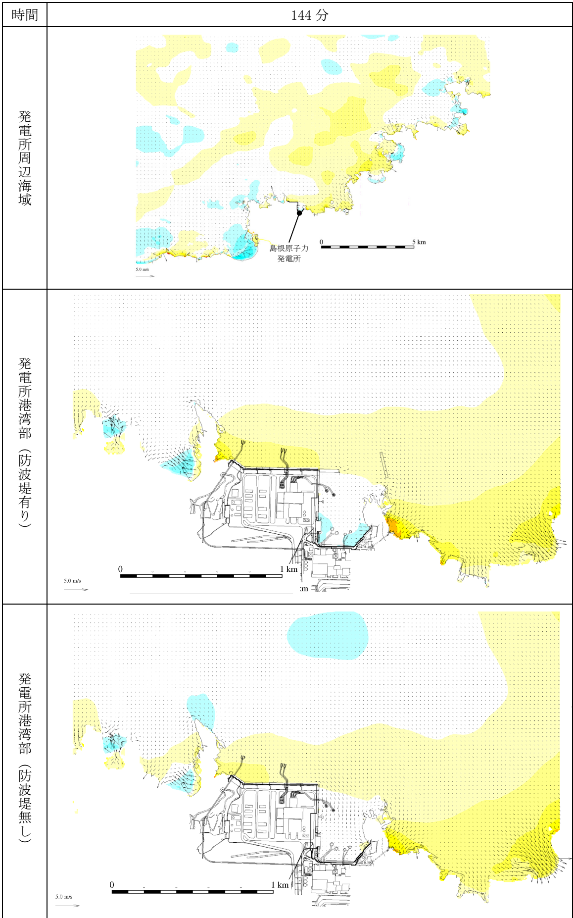
第 1 図(89) 基準津波 1 の水位変動・流向ベクトル
