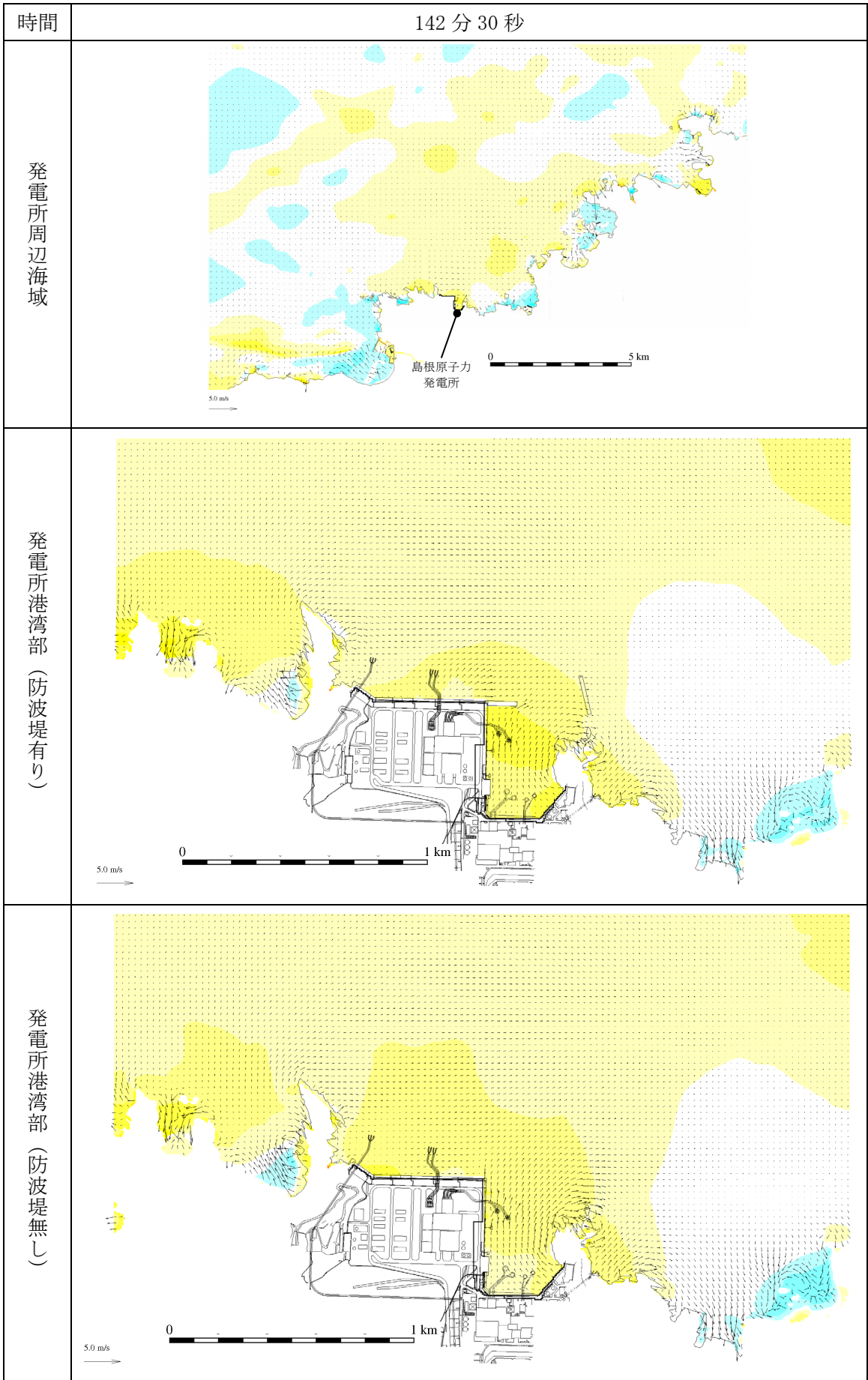
第 1 図(86) 基準津波 1 の水位変動・流向ベクトル
