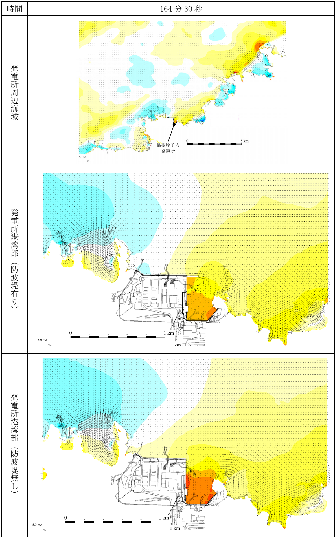
第 1 図 (130) 基準津波 1 の水位変動・流向ベクトル
