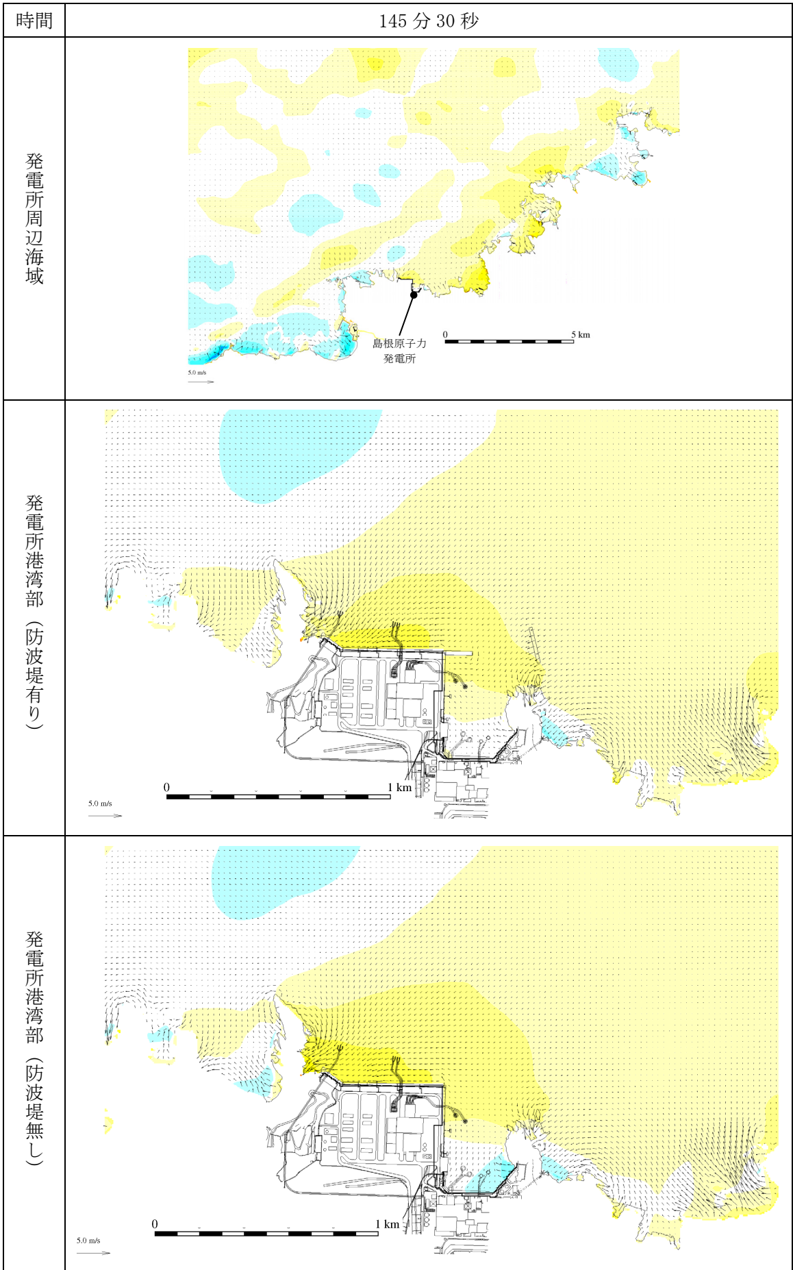
第 1 図(92) 基準津波 1 の水位変動・流向ベクトル
