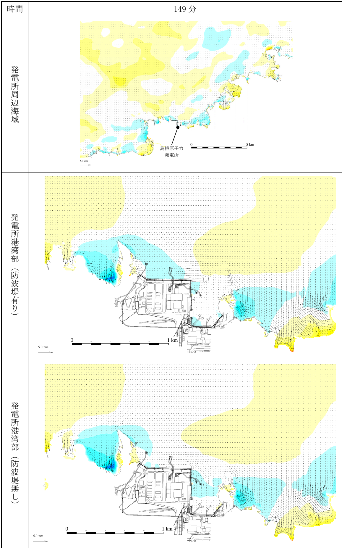
第 1 図(99) 基準津波 1 の水位変動・流向ベクトル
