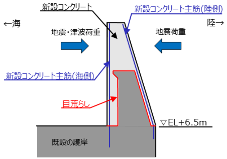
重力擁壁の構造
