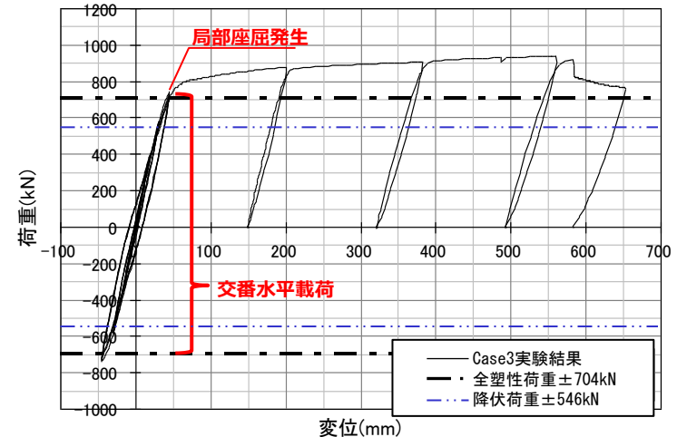
水平荷重と変形の関係
