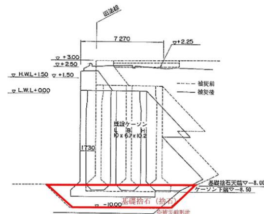
検討対象断面（釧路港北埠頭岸壁）
