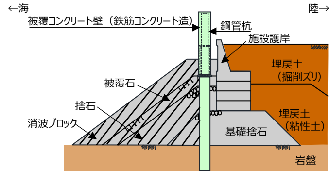
施設護岸前出し部（③－③断面）
