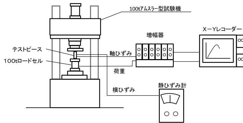
一軸圧縮試験装置図
