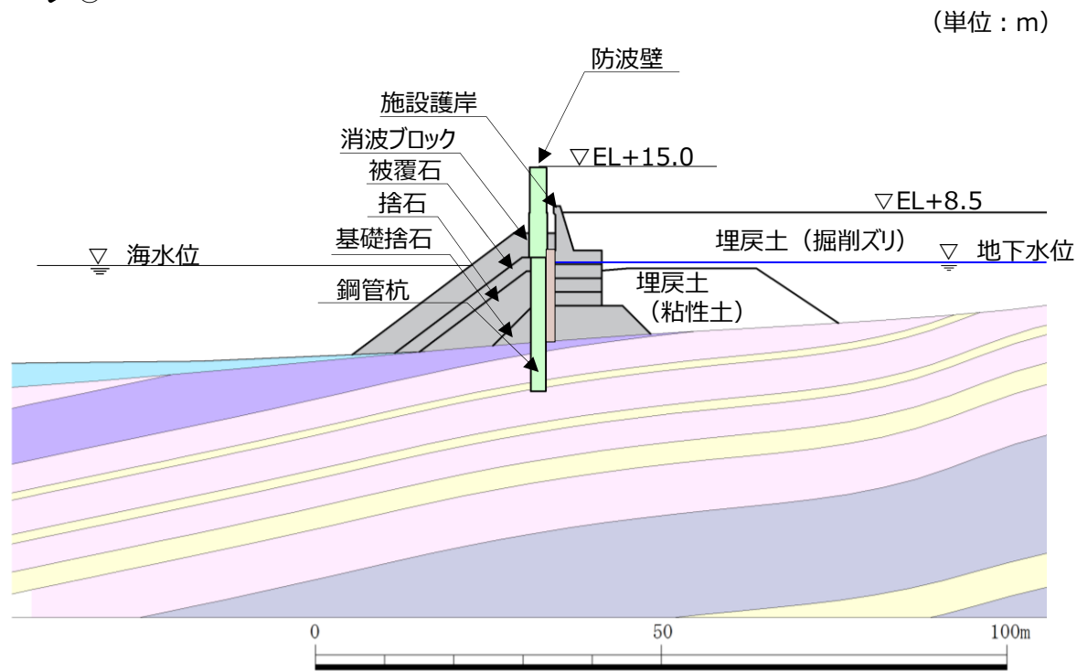
防波壁（多重鋼管杭式擁壁）施設護岸前出し部（③-③断面） 地質断面図
