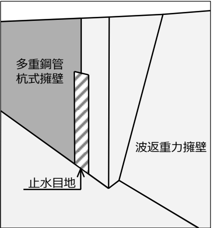
③多重鋼管杭式擁壁/波返重力擁壁 境界
