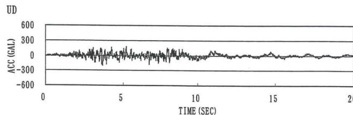
検討用地震動_ポートアイランド鉛直アレー地震観測網のGL-32mに設置の加速度計による1995兵庫県南部地震の際の観測記録
