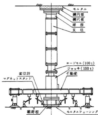
平板载荷試験装置
