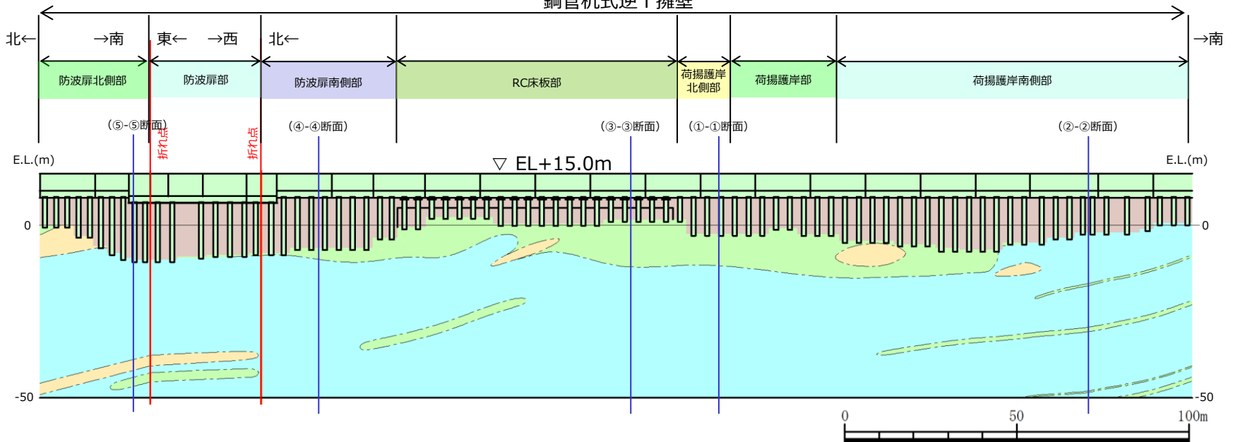
防波壁（鋼管杭式逆T擁壁） 岩級縦断図
