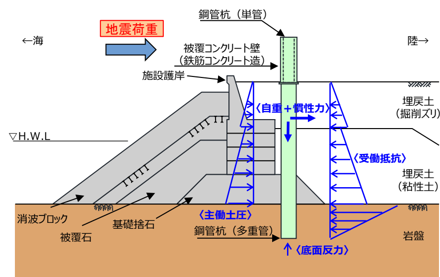
荷重図
