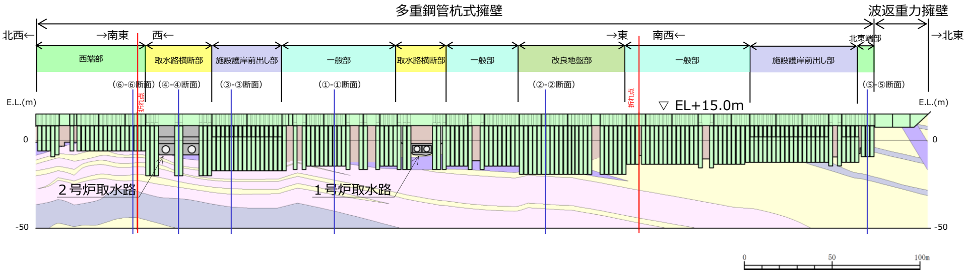
防波壁 (多重鋼管杭式擁壁) 岩相縦断面図
