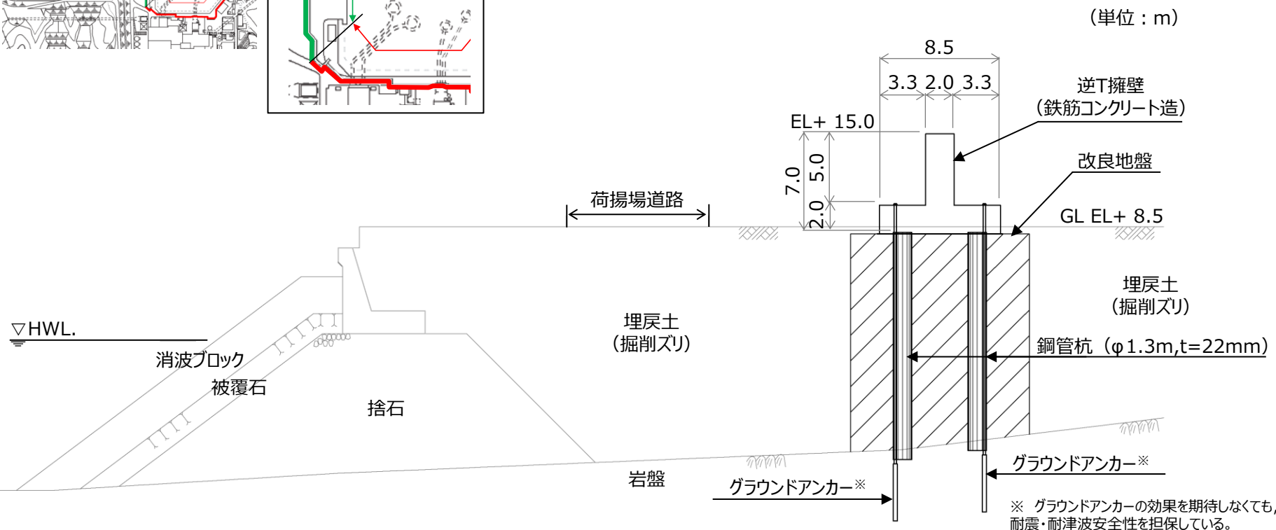
防波壁（鋼管杭式逆T擁壁）防波扉南側部（④－④断面） 断面図
