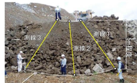
押し崩し試験の安息角計測イメージ
