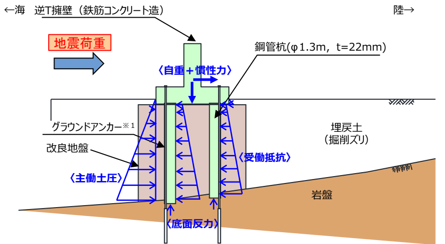
荷重図
