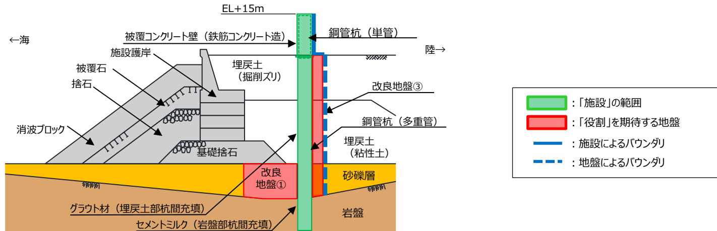
防波壁（多重鋼管杭式擁壁）（改良地盤部）における構造上のバウンダリ
