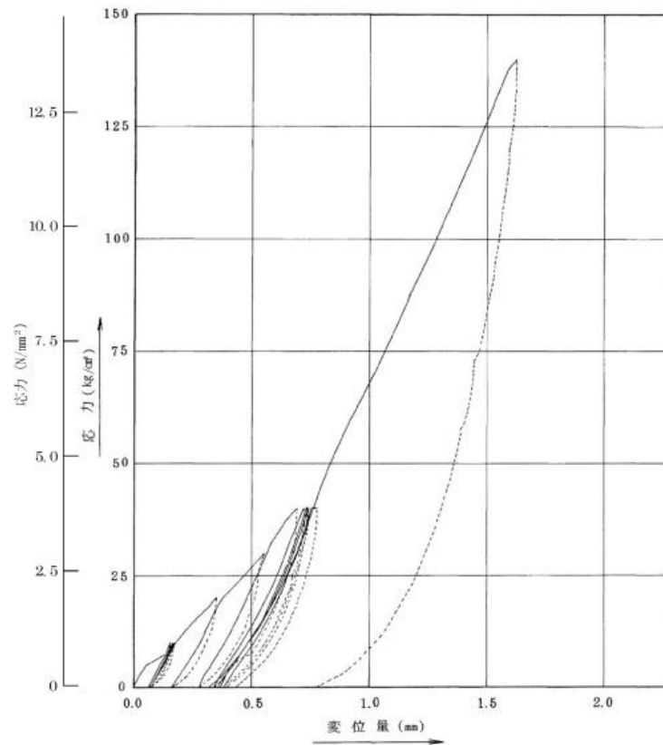
CM級の平板载荷試験結果
