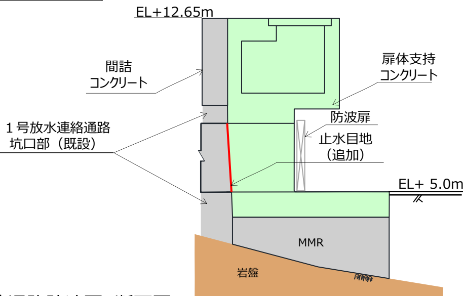
C-C 断面
