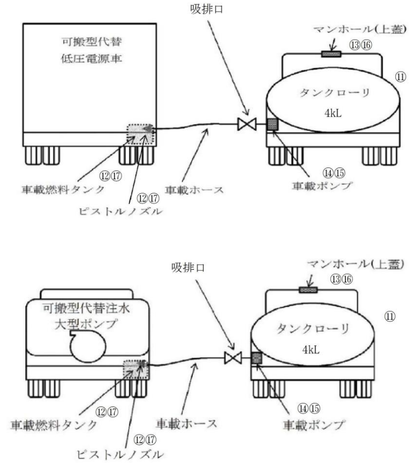
第 1.14.55 図 タンクローリから各機器への給油 概要図
