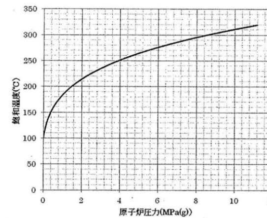
第58-8-3図 飽和温度/圧力の関係を利用した圧力の推定
