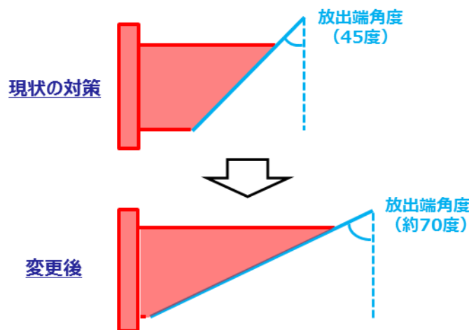
図2 放出端の雨水侵入防止対策
