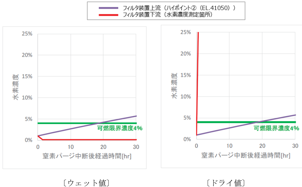
図 6 水素濃度の窒素パージ中断後の時間経過（ウェット値，ドライ値）
