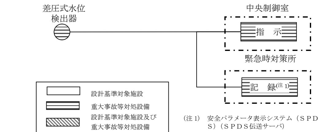
図2 スクラバ容器水位の概略構成図
