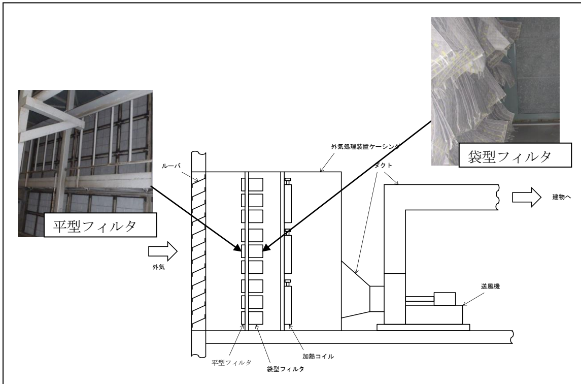
第3.2-2図 中央制御室換気系外気取入状況
