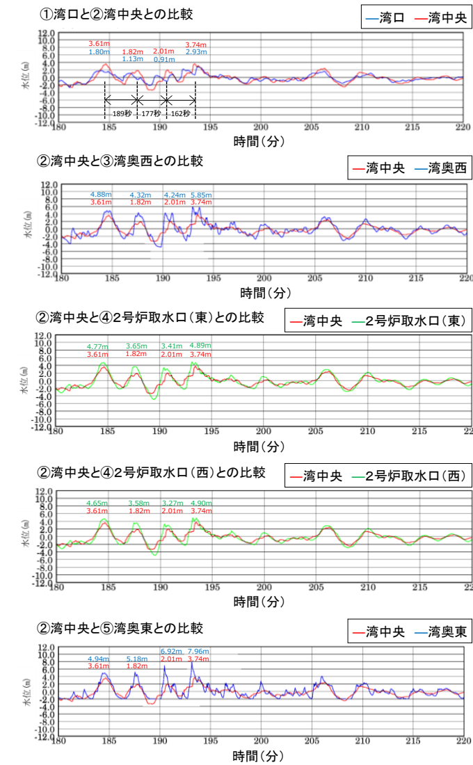
図3 水位の時刻歴波形 (輪谷湾)
