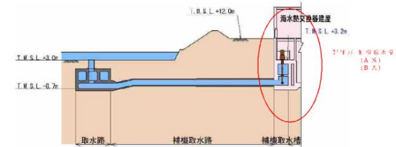
添付第6-2図(7) 5号炉取水路 (F-F断面)
