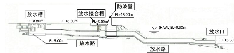
図2-12 3号炉放水施設断面図
