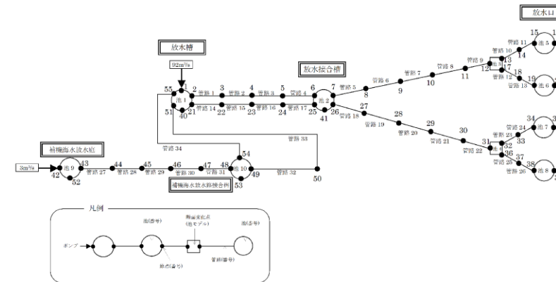
図3-6 3号炉放水施設の管路計算モデル図
