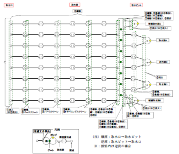
第1-2図 取水路の管路解析モデル
