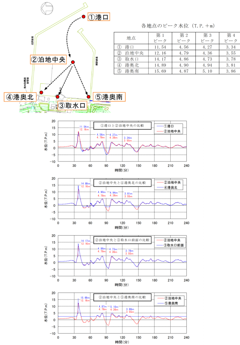
第2図 港湾内における時刻歴波形の地点別比較
