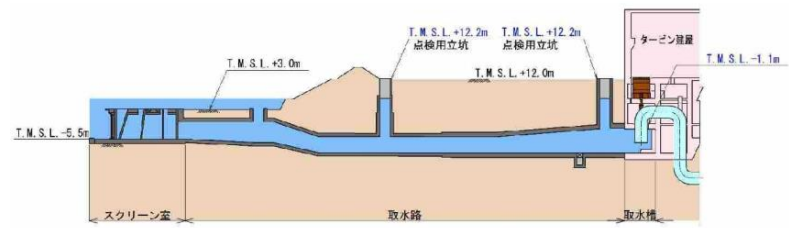
添付第6-2図(4) 7号炉取水路 (C-C断面)
