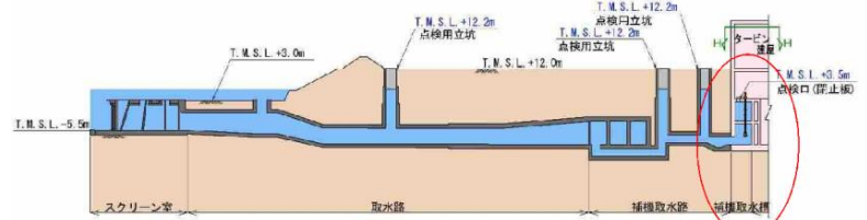
添付第6-2図(5) 7号炉取水路 (D-D断面)
