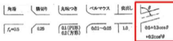
第2-3図 入口形状と損失係数 f_a (土木学会水理公式集 (平成11年版) p.375)
