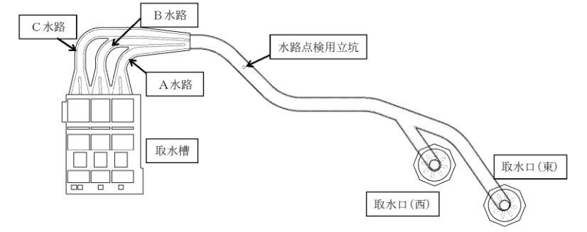
図2-5 3号炉取水施設平面図
