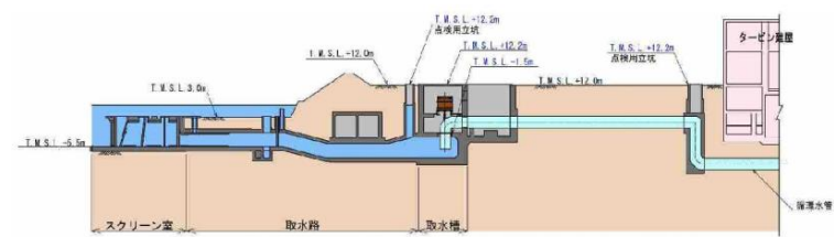
添付第6-2図(6) 5号炉取水路 (E-E断面)
