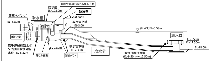
図2-4 2号炉取水施設断面図
