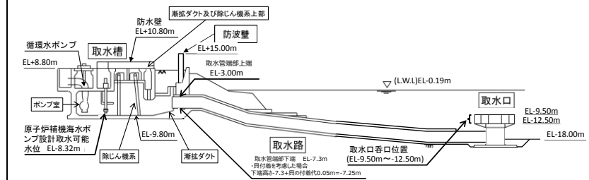
図15 2号炉取水施設断面図
