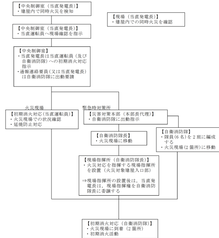
図2 建屋内同時火災の対応フロー
