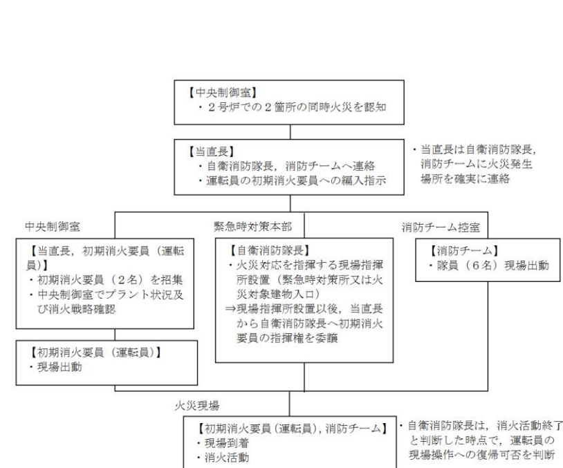
第1図 建物内部での同時火災に対する対応フロー
