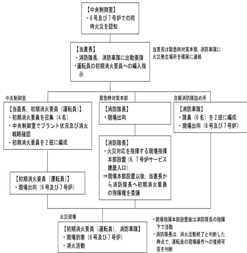
第1図 建屋内での同時火災に対する対応フロー
