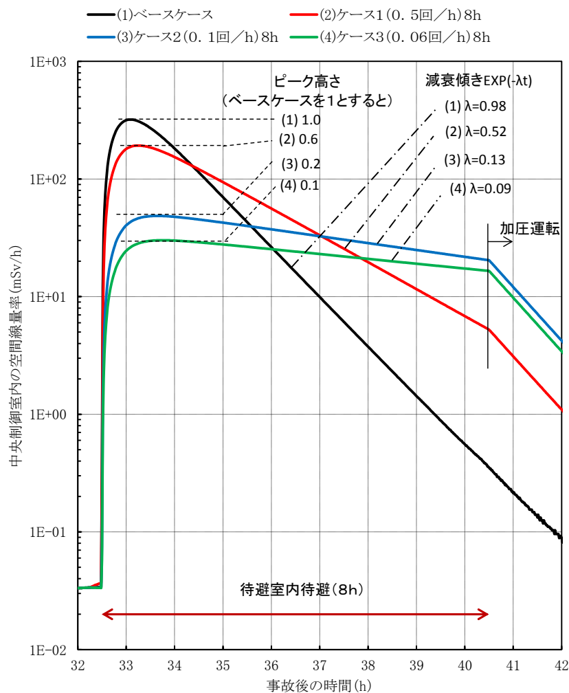
図 24-1 中央制御室内の空間線量率の推移
