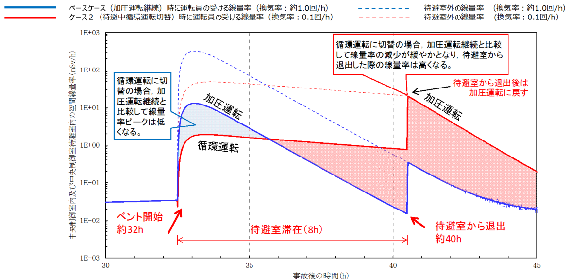
図 24-1 中央制御室内の空間線量率の推移
