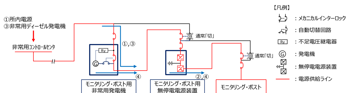
第 1 図 モニタリング・ポストの電源構成概要図
