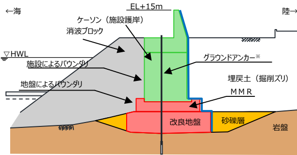
地盤改良部
