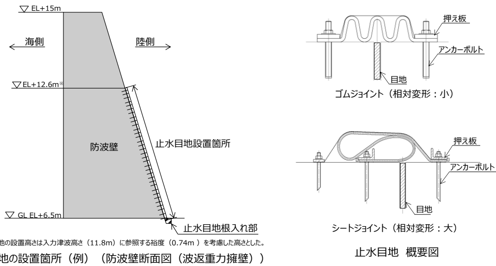
第 8-1 図 防波壁の止水目地の設置箇所及び概要図
