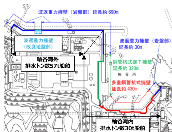
第 10-5-5 図 対象漂流物の設定
