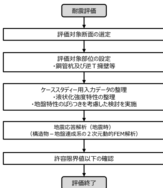
第 6-19 図 設計フロー
