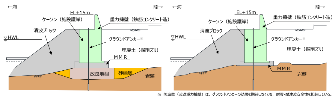
第 7-7 図 防波壁（波返重力擁壁）断面図
