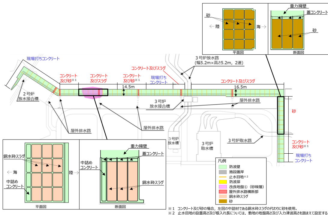
第7-4 図 防波壁（波返重力擁壁）におけるケーソン中詰材の施工状況
