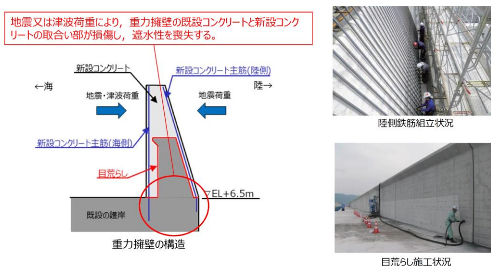
第 7-30 図 防波壁（波返重力擁壁）弱部②概要図
