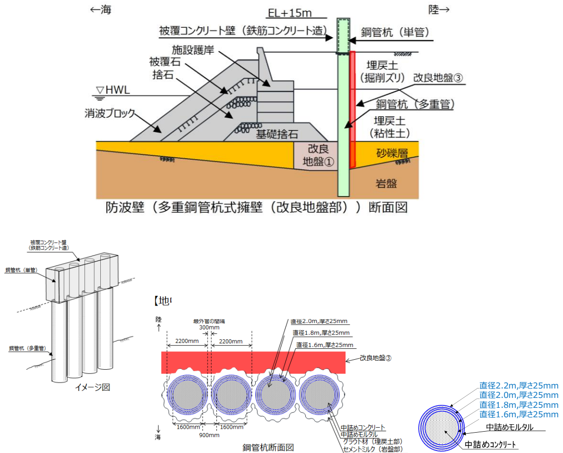
第5-6 図 防波壁（多重鋼管杭式擁壁）の各部位の仕様詳細図
