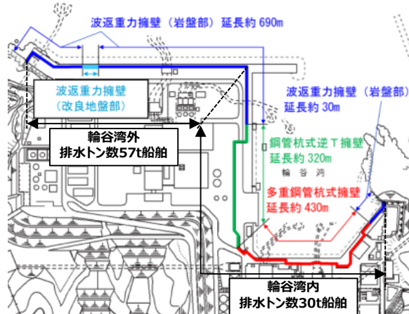
第 10-4-4 図 対象漂流物の設定
