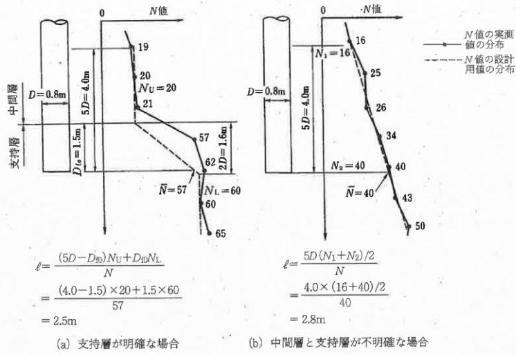
解説図 15.2.2.3-1 打込み杭工法による先端開放鋼管杭の支持層への換算根入れ深さ l
