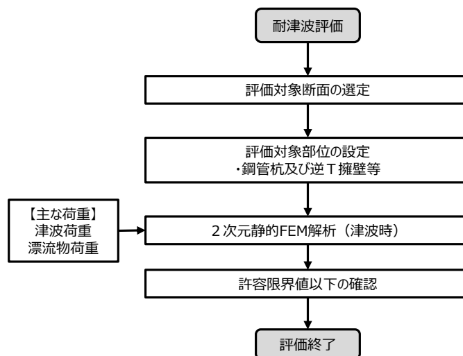
第 6-21 図 解析の概要
