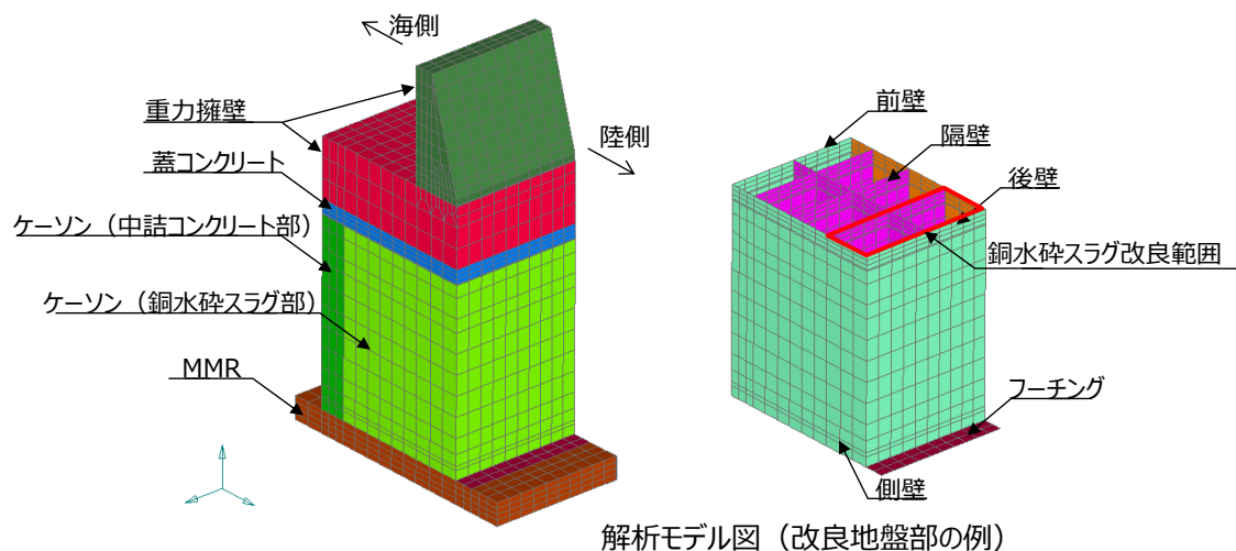
第10-5-3 図 3次元静的FEM解析の解析モデル図 (改良地盤部)
