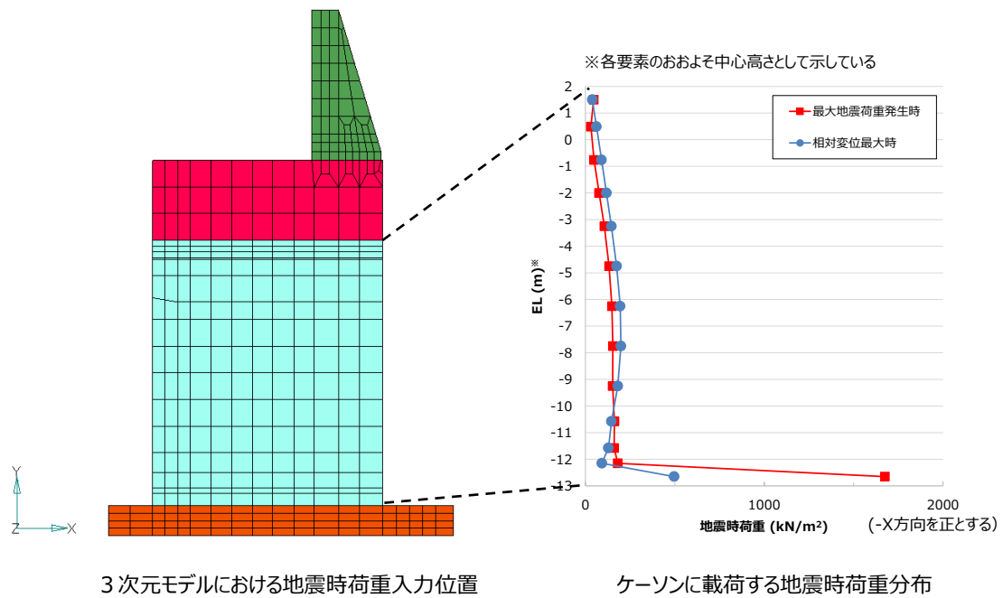
第 7-34 図 ケーソンの頂底版間の相対変形量が最大となる時刻における地震時荷重分布
