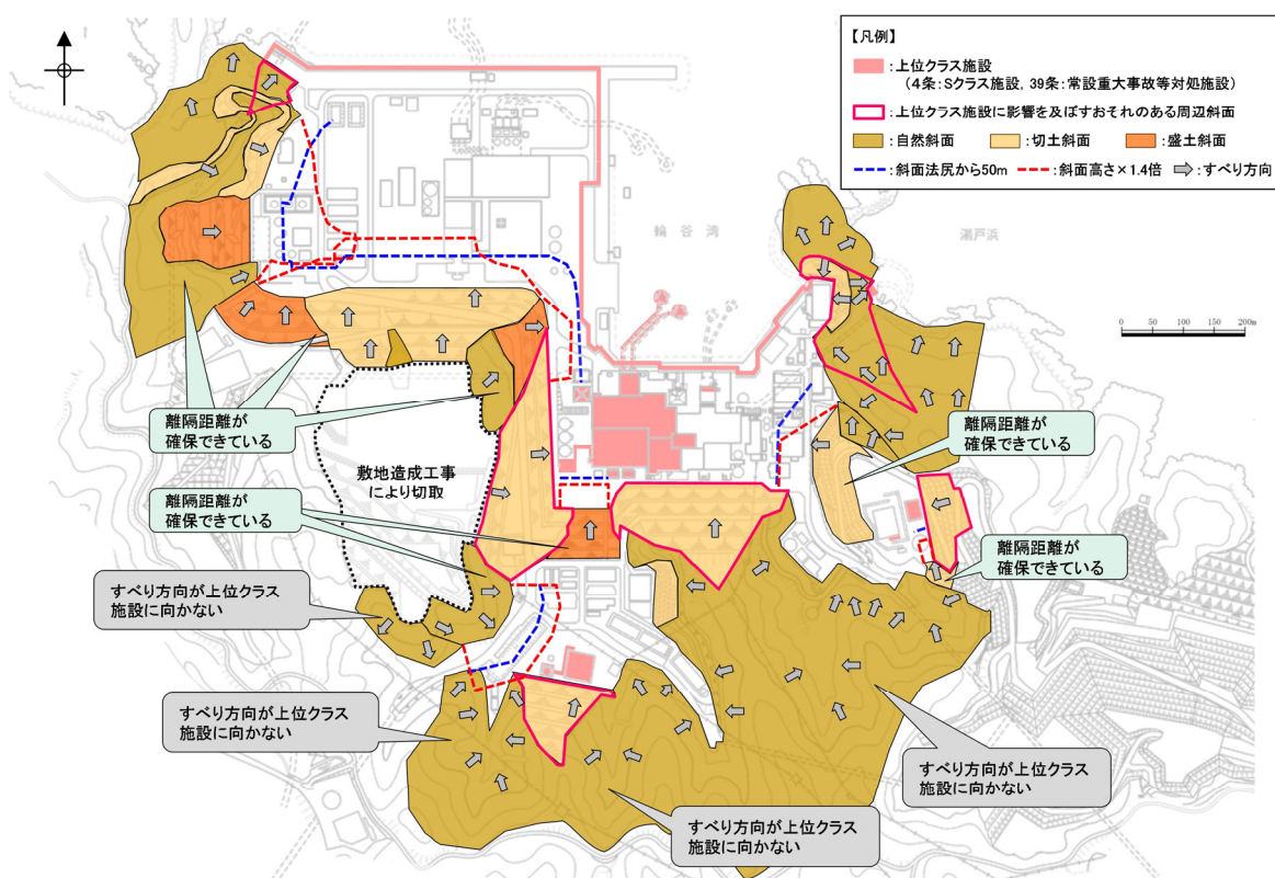
第2図 上位クラス施設に影響を及ぼすおそれのある斜面の平面位置図
