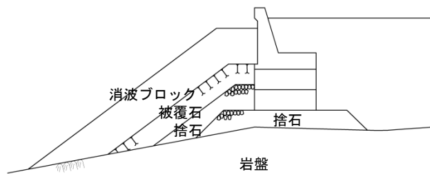
第5図 護岸の構造概要
