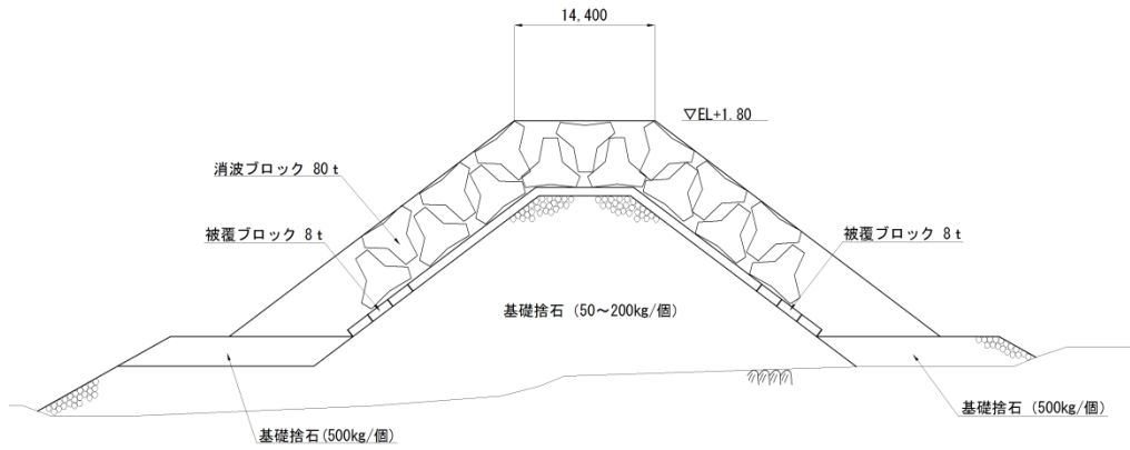
第4図 東防波堤の構造概要
