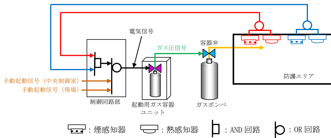
第6図 全域ガス消火設備（専用型）の系統構成
