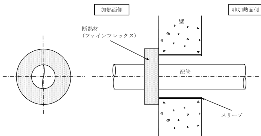
第8図 断熱材施工例
