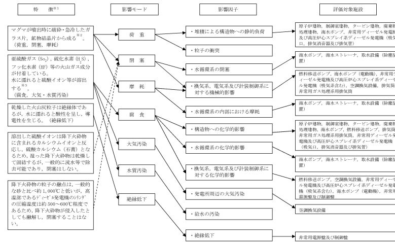
第2-1図 降下火砕物の特徴と影響因子
