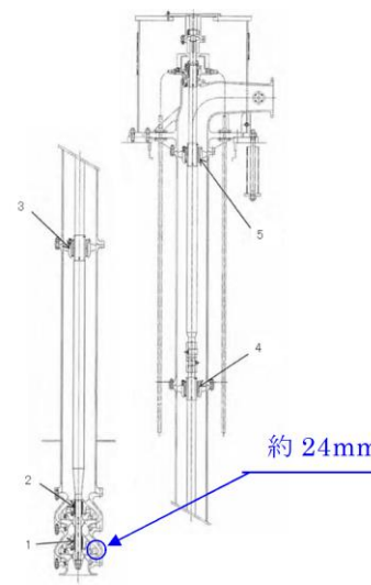
第6図 非常用ディーゼル発電機(高圧炉心スプレー系ディーゼル発電機を含む。)用海水ポンプ断面図
