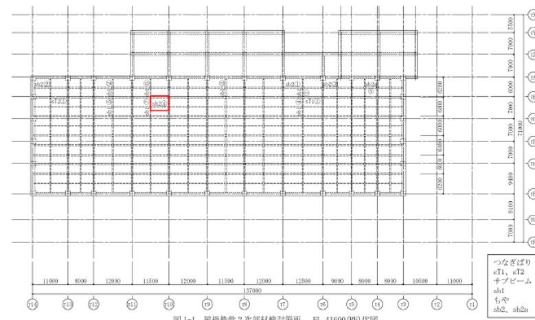
図 1-1 船橋鉄骨 2 次部材検討箇所 EL. 41600 (BF) 状態
