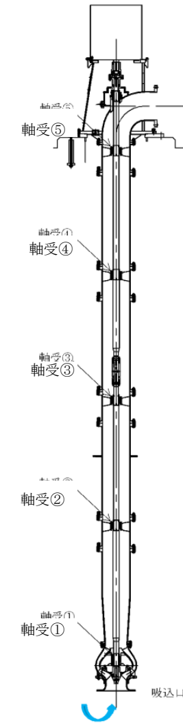
第2-2図 原子炉補機海水ポンプ軸受構造
