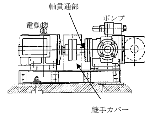
第 4-2 図 燃料移送ポンプ概略構造図
