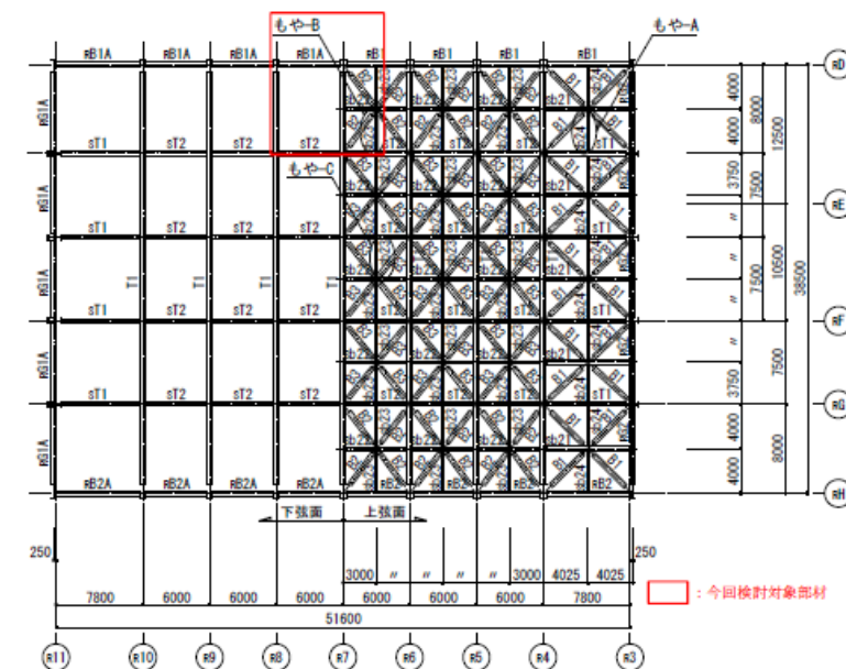
第3-3図 部材位置図 (トラス二次部材：母屋)
