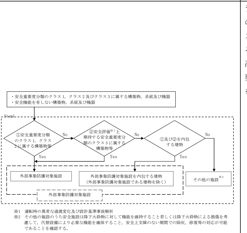
第 1.3-1 図 外部事象防護対象施設評価フロー
