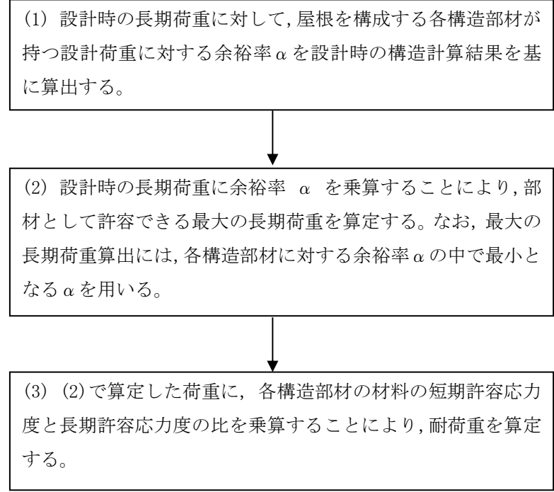
第1-1図 耐荷重算定フロー
