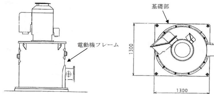
第2図 非常用ディーゼル発電機（高圧炉心スプレィ系ディーゼル発電機含む。）海水系ポンプ 評価部位概要図
