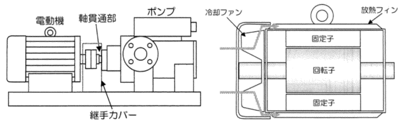
図 5-3 燃料移送ポンプ概略構造図
