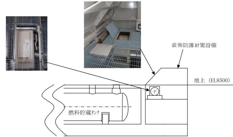
第 4-1 図 燃料移送ポンプ設置状況 (概略)
