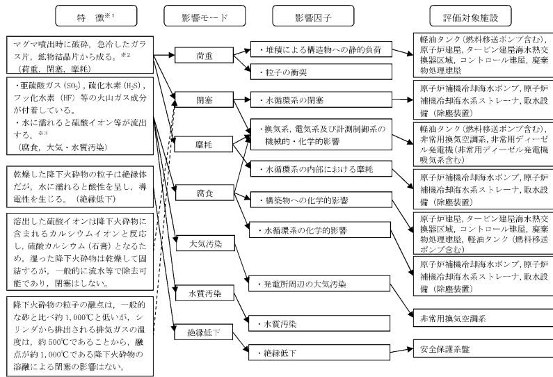
図2-1 降下火砕物の特徴と影響因子
