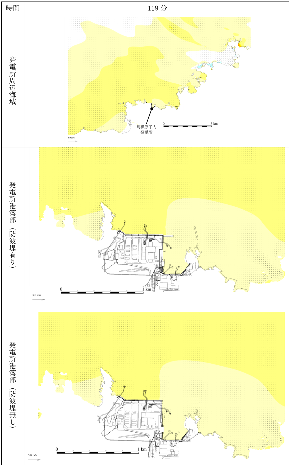
第 1 図 (39) 基準津波 1 の水位変動・流向ベクトル
