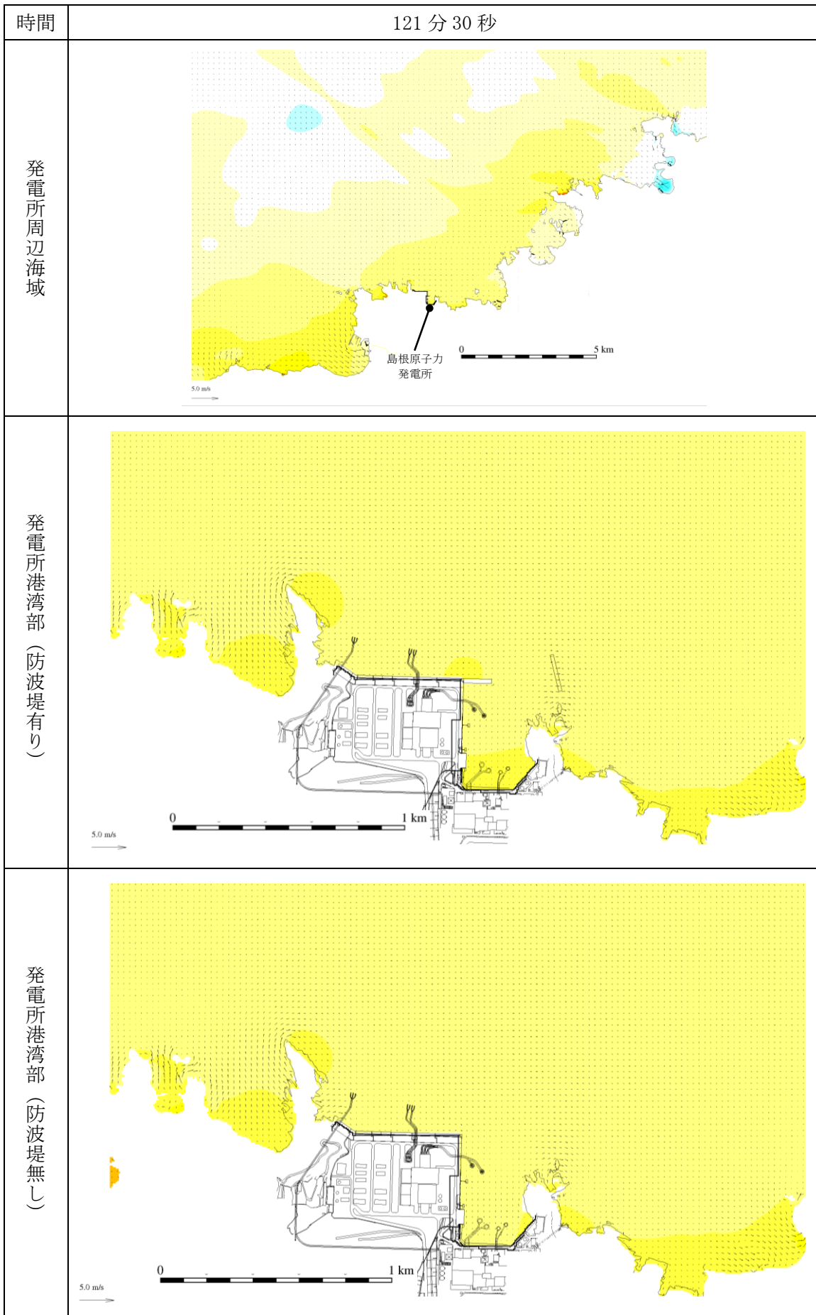
第 1 図(44) 基準津波 1 の水位変動・流向ベクトル
