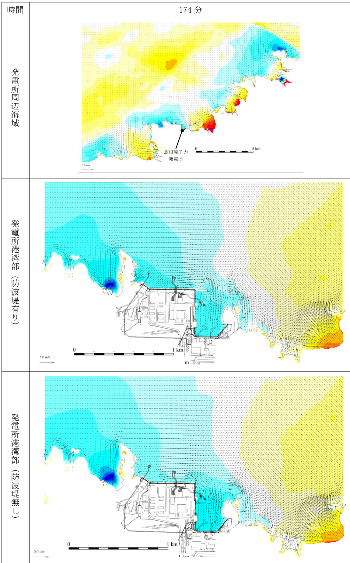
第 1 図(149) 基準津波 1 の水位変動・流向ベクトル
