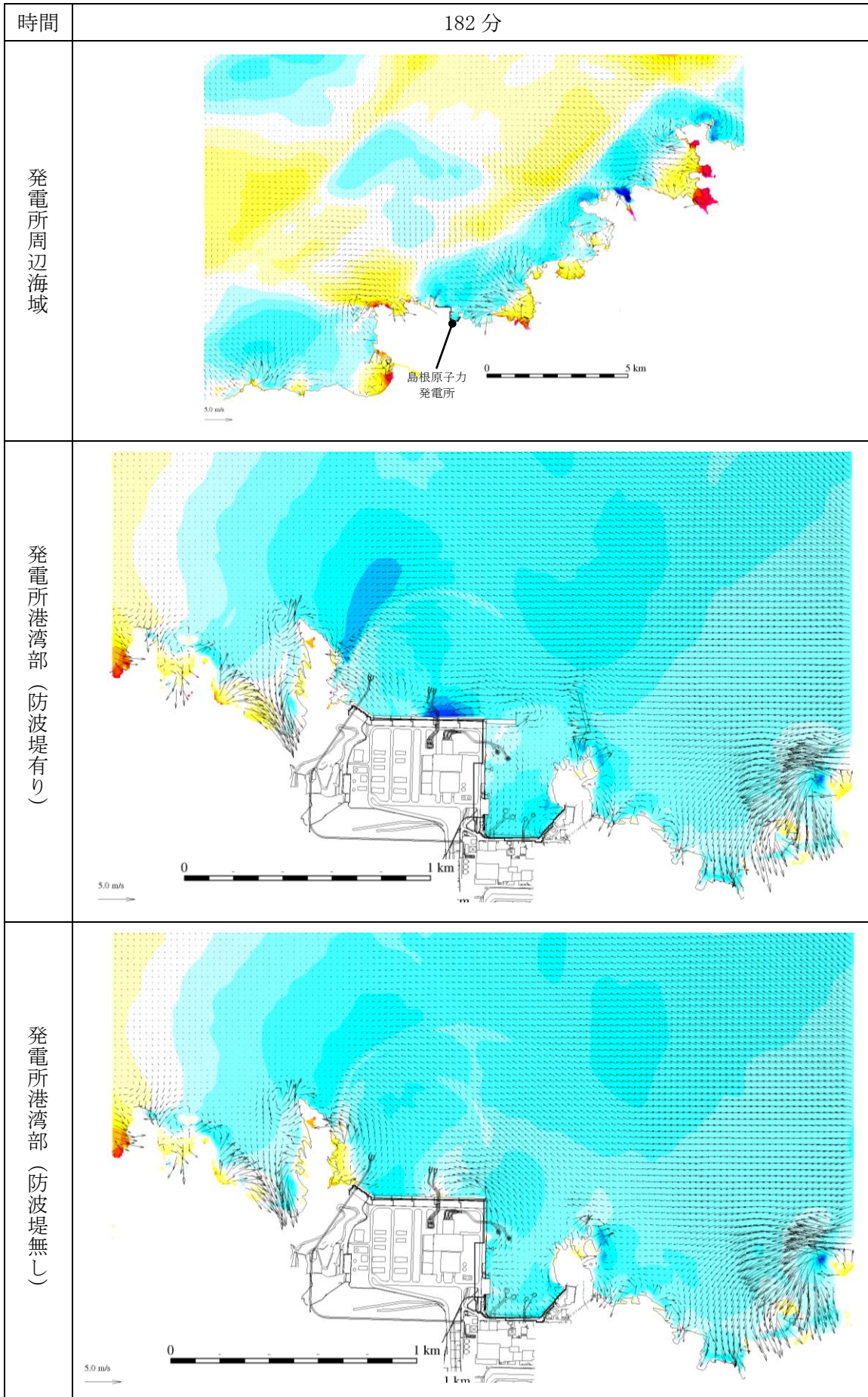
第 1 図(165) 基準津波 1 の水位変動・流向ベクトル
