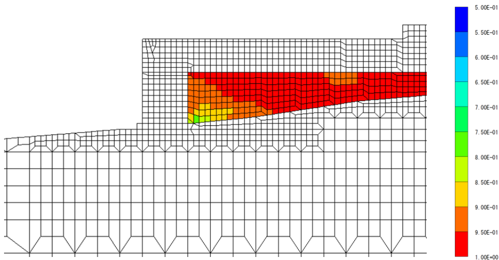
第 9 図 過剰間隙水圧比分布図
