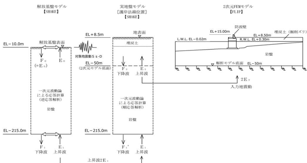
第5図 入力地震動算定の概念図
