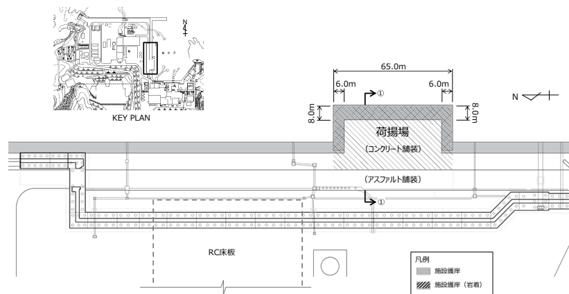
第1図 荷揚場平面図
