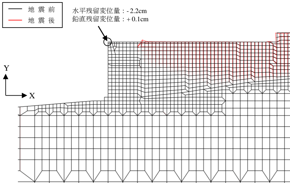
第 8 図 最終変形量図
