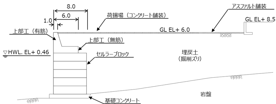
第2図 荷揚場断面 (①-①)
