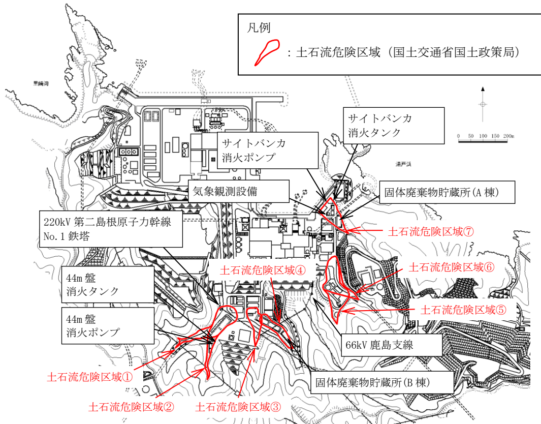
図1 島根原子力発電所周辺における土石流危険区域及び対象施設（安全施設等）位置図
