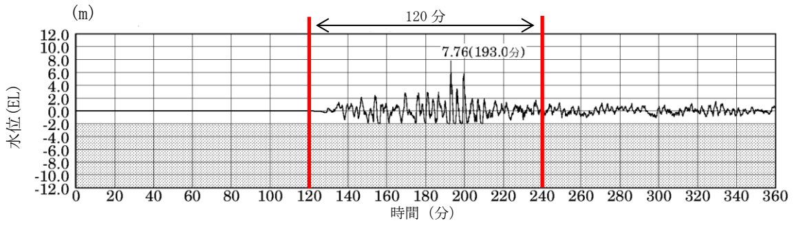
屋外排水路⑬ (入力津波 5, 防波堤無し)
