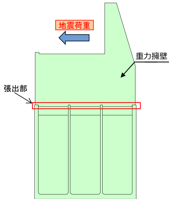
防波壁（波返重力擁壁）輪谷部 断面図
