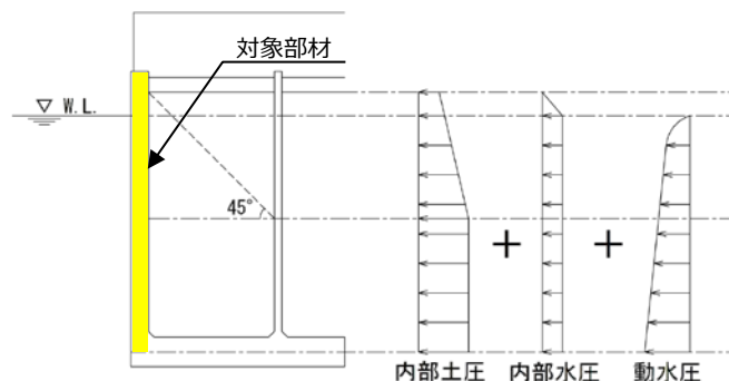
側壁（前壁）に生じる作用イメージ図 （地震時、海側への作用）
