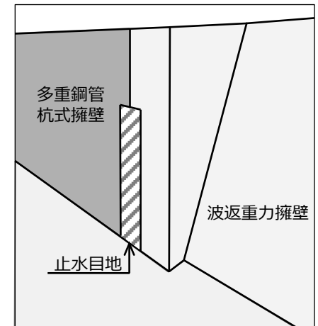
③ 多重鋼管杭式擁壁/波返重力擁壁 境界
