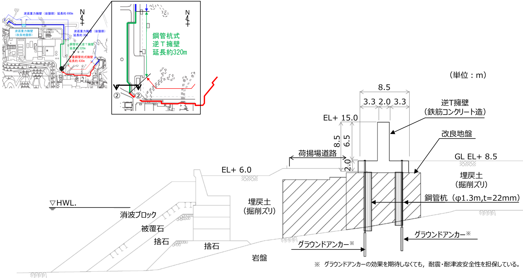
防波壁（鋼管杭式逆T擁壁）荷揚護岸南側部（②-②断面） 断面図
