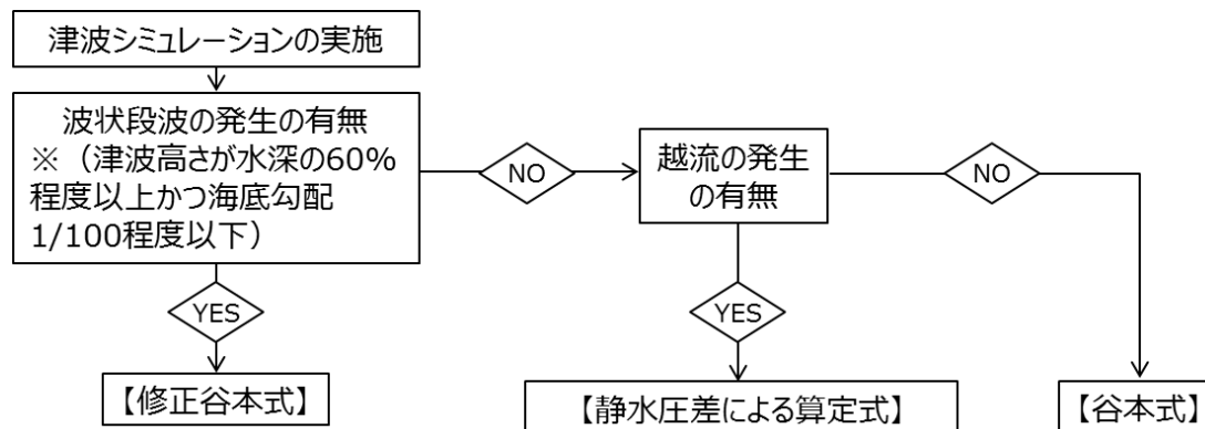
防波堤に対する津波波力算定手順 （港湾基準（H30）より抜粋）
