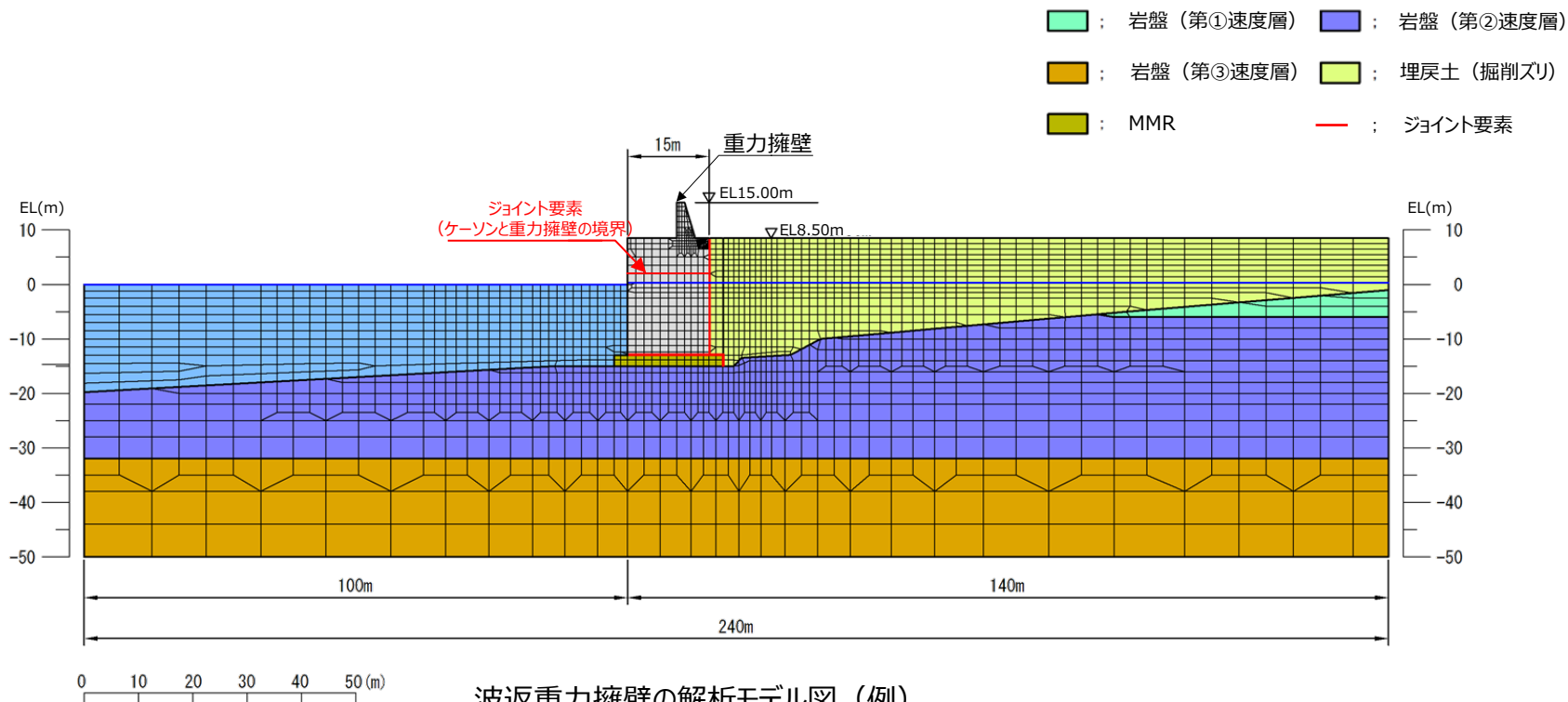
波返重力擁壁の解析モデル図（例）
