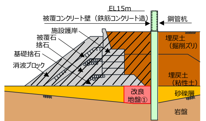
地盤改良部断面（②-②断面）
