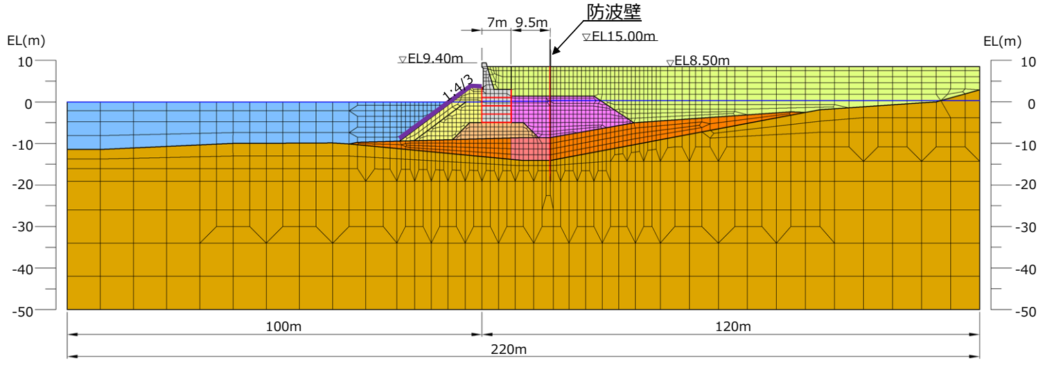
多重鋼管杭式擁壁の解析モデル図（例）
