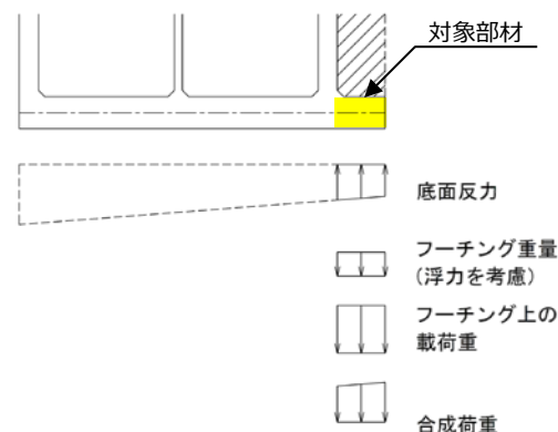
フーチングに生じる作用イメージ図
