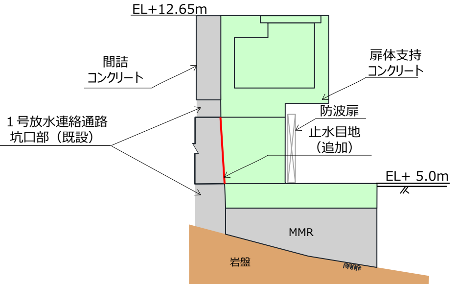
C-C 断面
