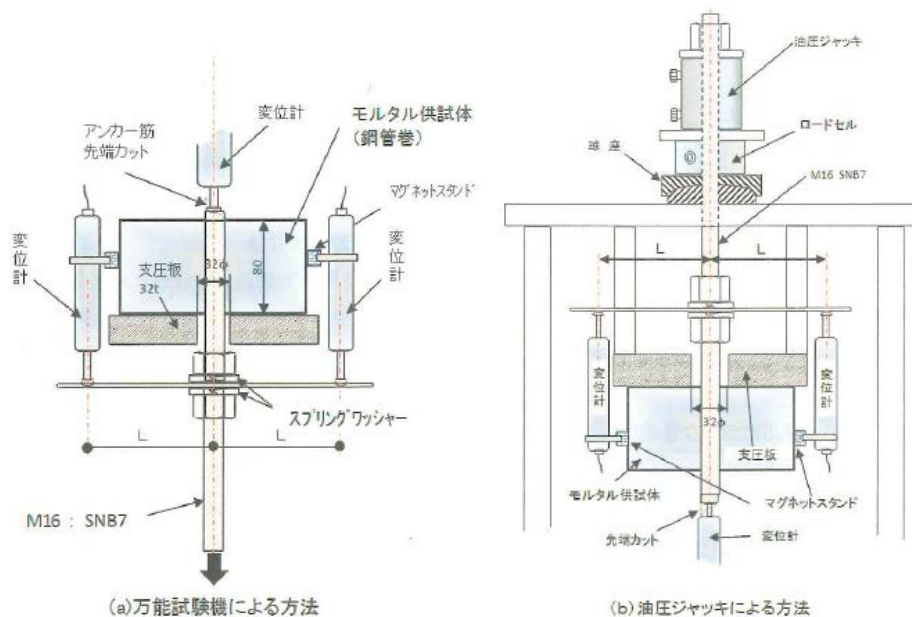
接着系アンカーのセット試験方法の一例
