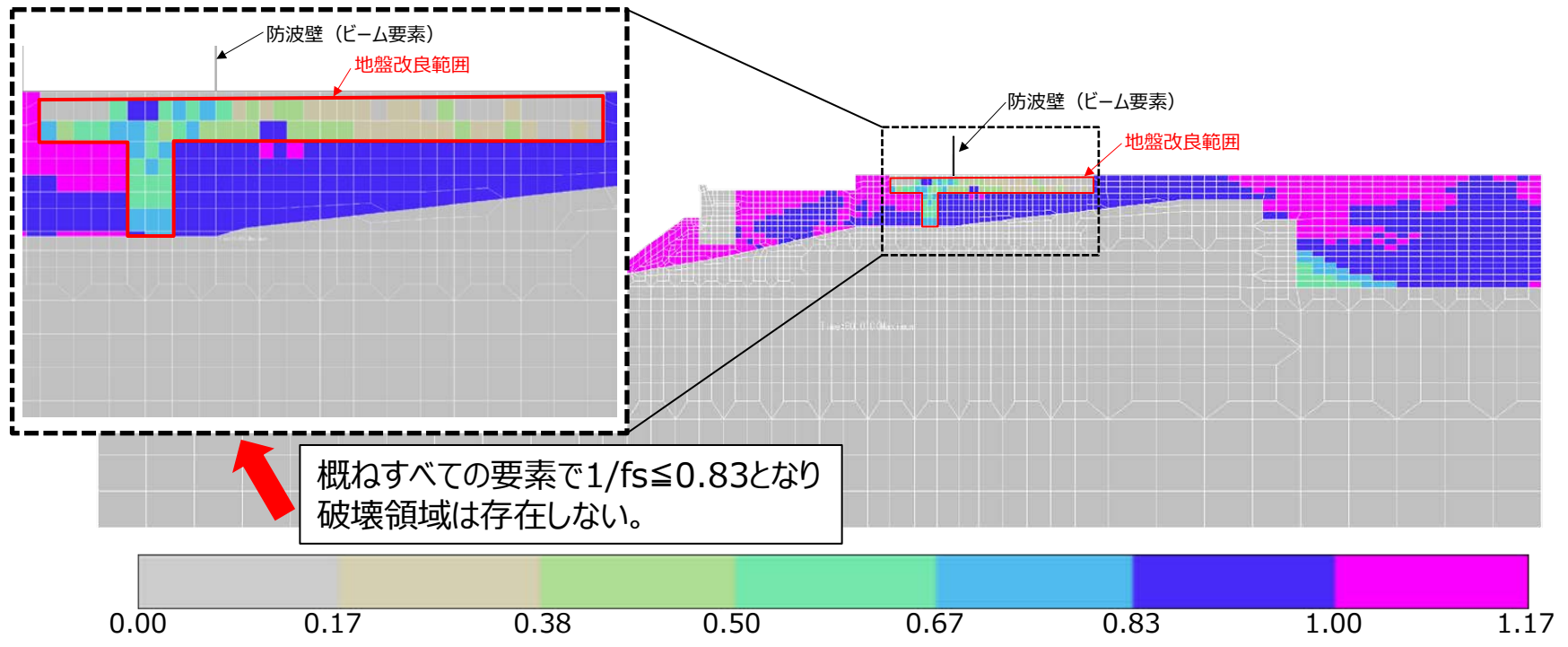
全時刻での局所安全率の逆数の分布
