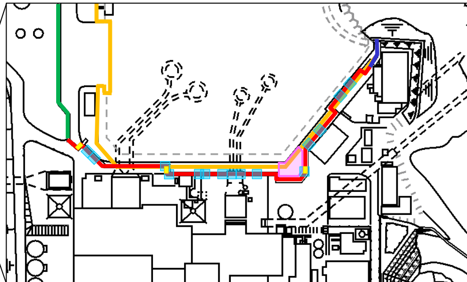
防波壁平面図（多重鋼管杭式擁壁）
