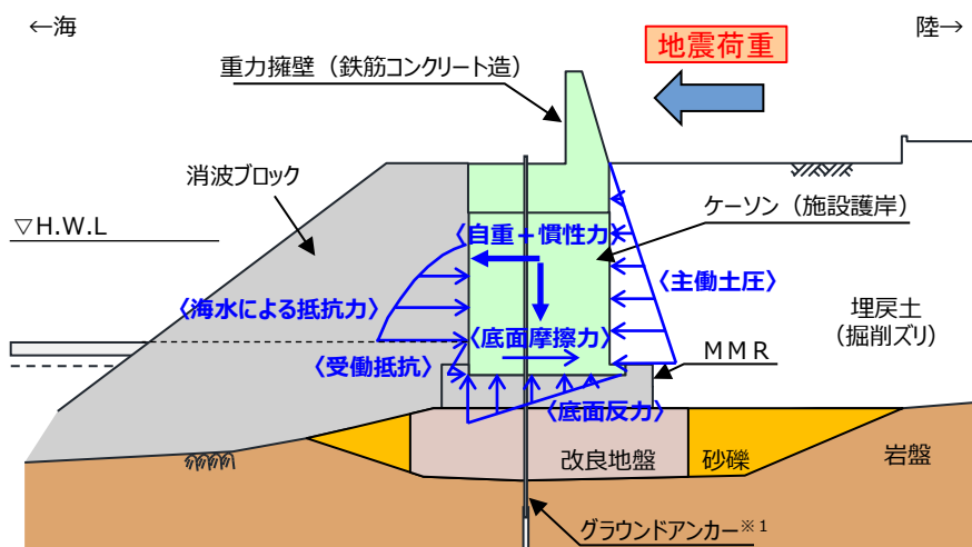
荷重図
