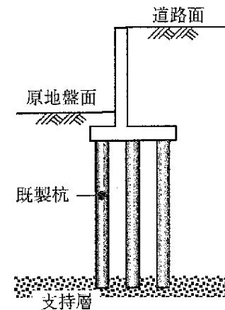
杭基礎形式の擁壁 (道路土工 擁壁工指針（平成24年7月）より引用)
