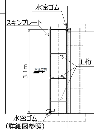
⑤ 1号放水連絡通路防波扉 断面図
