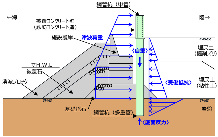
荷重図
