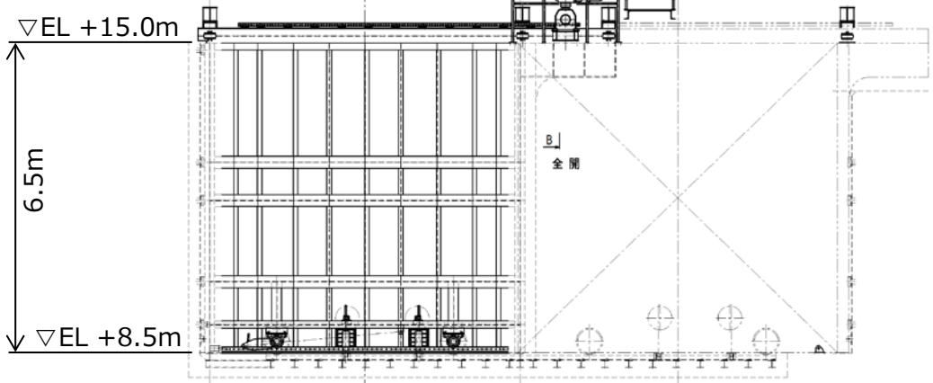
②防波壁通路防波扉（1, 2号炉北側） 正面図
