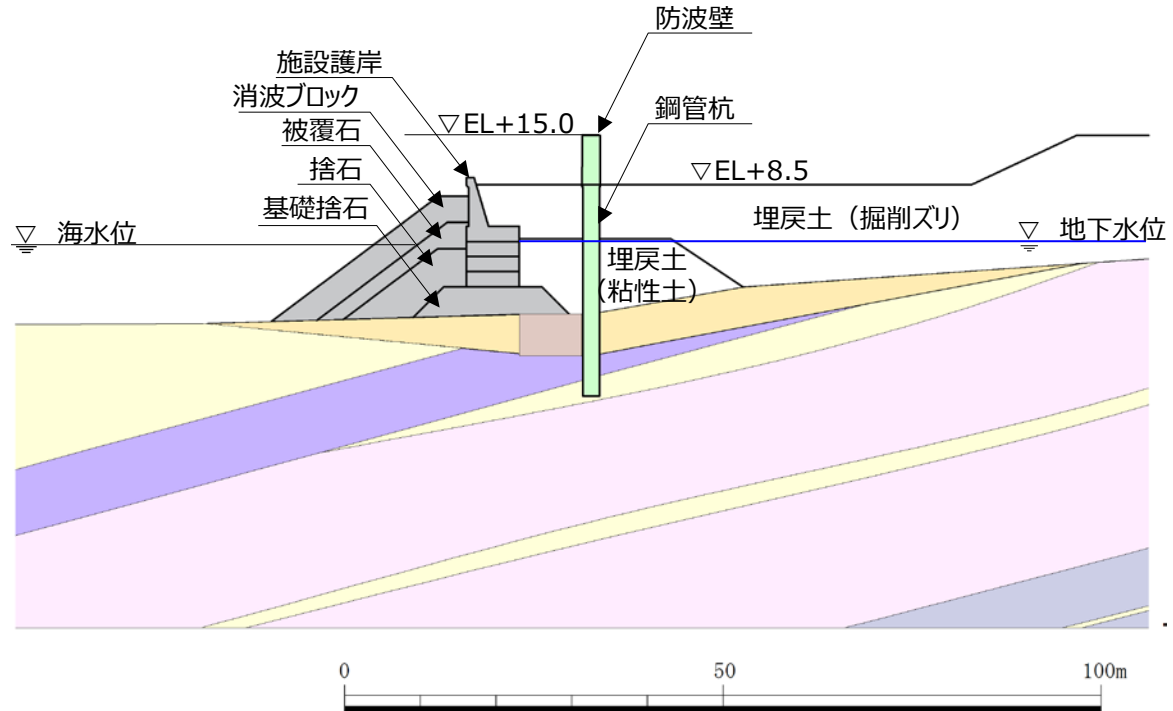
防波壁（多重鋼管杭式擁壁）改良地盤部（②-②断面） 地質断面図
