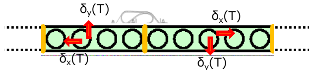
地震時の相対変形概念図 防波壁（多重鋼管杭式擁壁）の例
