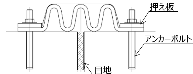
ゴムジョイント (相対変形: 小)
