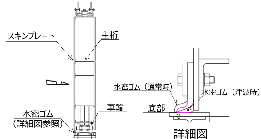
④防波壁通路防波扉（1, 2号炉北側） 断面図
