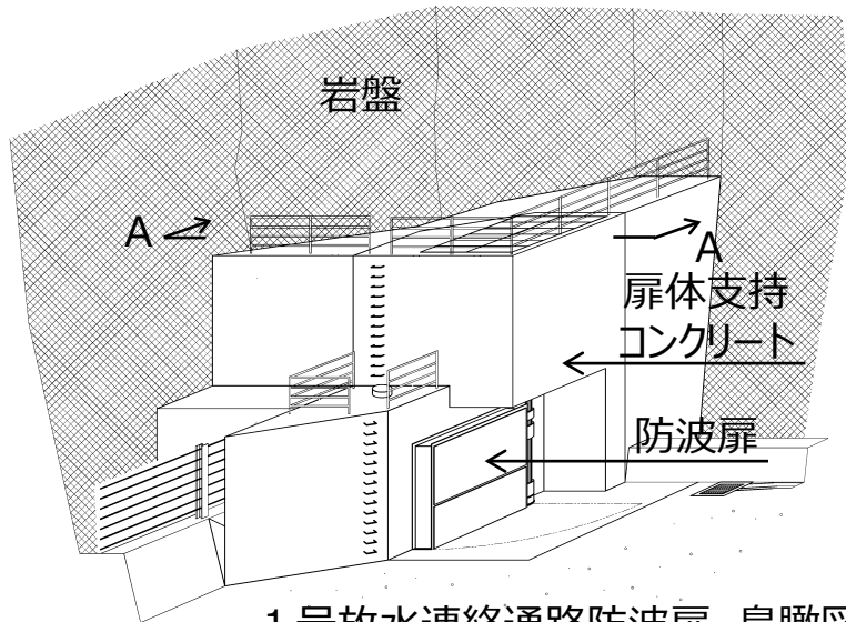
1号放水連絡通路防波扉 鳥瞰図
