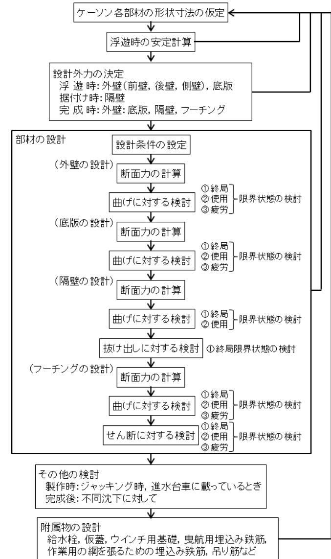
ケーソンの設計順序（港湾基準（H11）に基づき作成）
