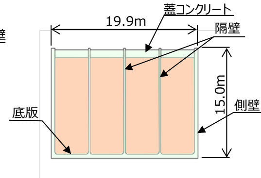
ケーソン構造図 (②-②断面)
