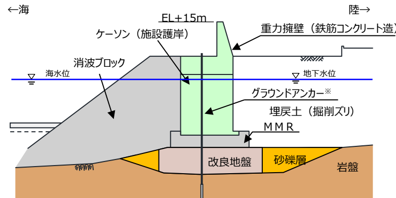
防波壁（波返重力擁壁）
