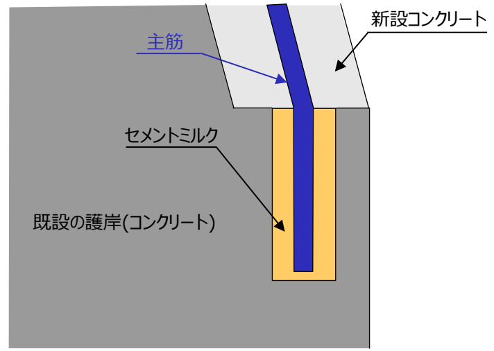
定着部の構造イメージ（陸側主筋）
