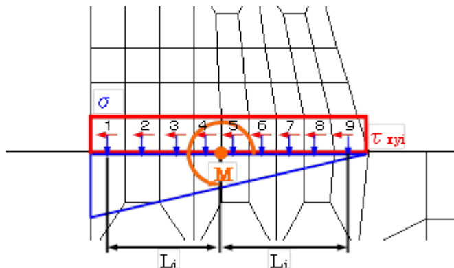
2次元動的FEM解析モデル図
