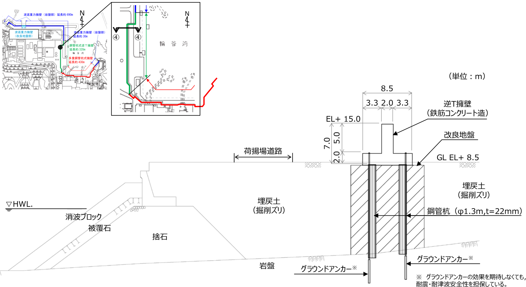
防波壁（鋼管杭式逆T擁壁）防波扉南側部（④－④断面） 断面図
