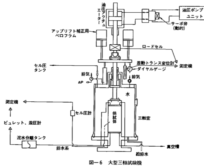
図-6 大型三軸圧縮試験機
