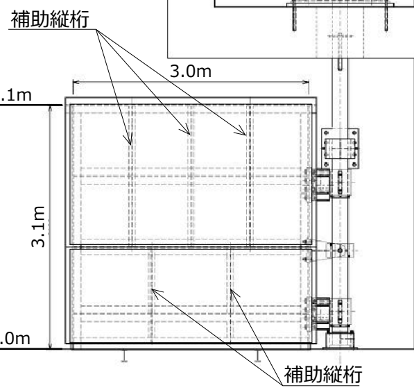
⑤ 1号放水連絡通路防波扉 正面図
