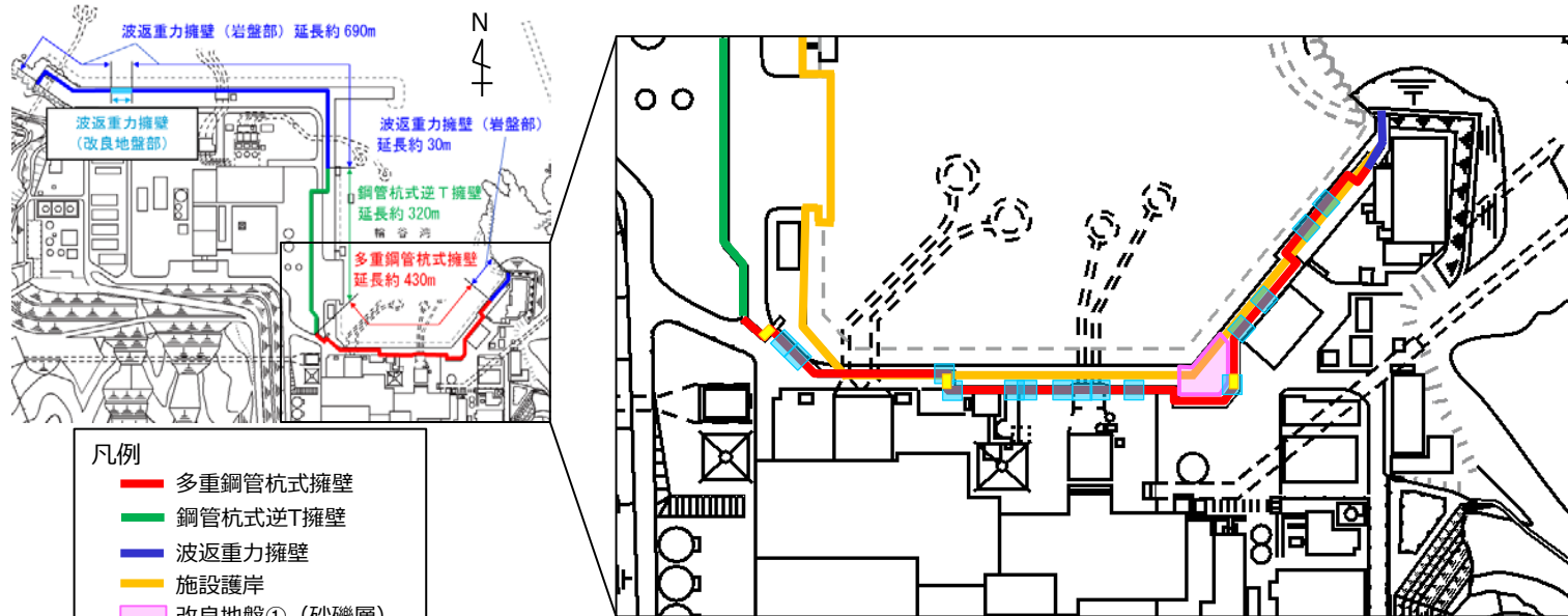
防波壁平面図 (多重鋼管杭式擁壁)
