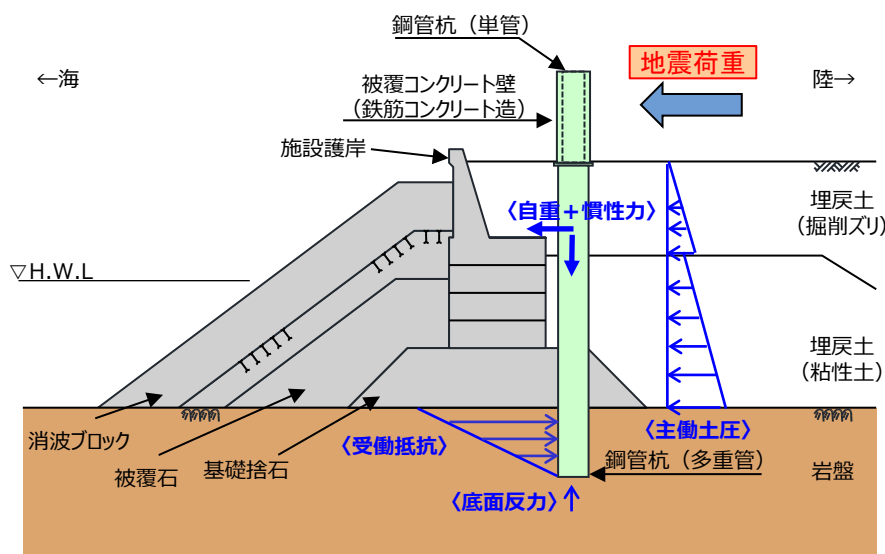
荷重図
