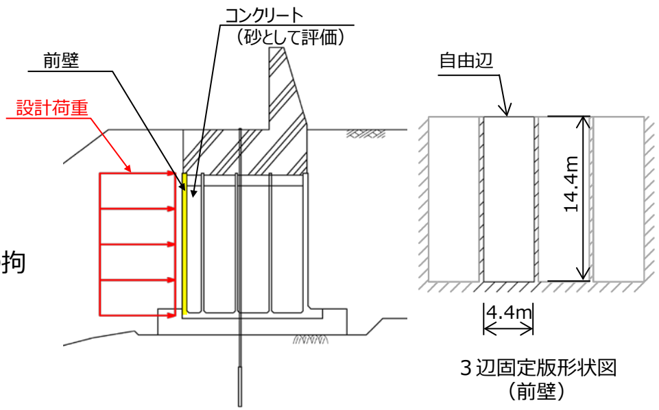
作用荷重イメージ図
