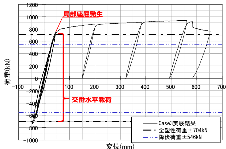
水平荷重と変形の関係
