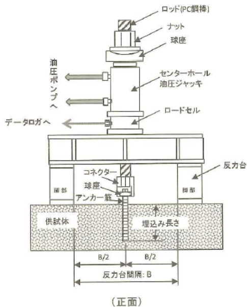
あと施工アンカーの引張試験方法の一例
