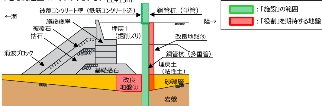
防波壁（多重鋼管杭式擁壁）（改良地盤部）における「施設」と「地盤」の区分
