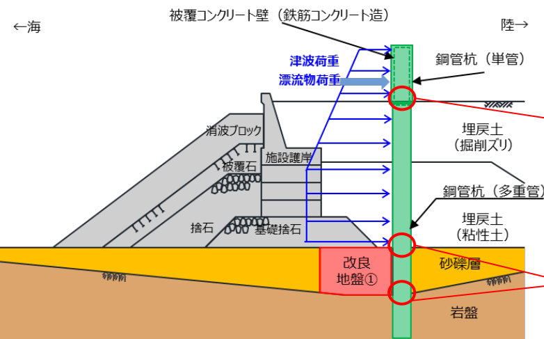
津波時
