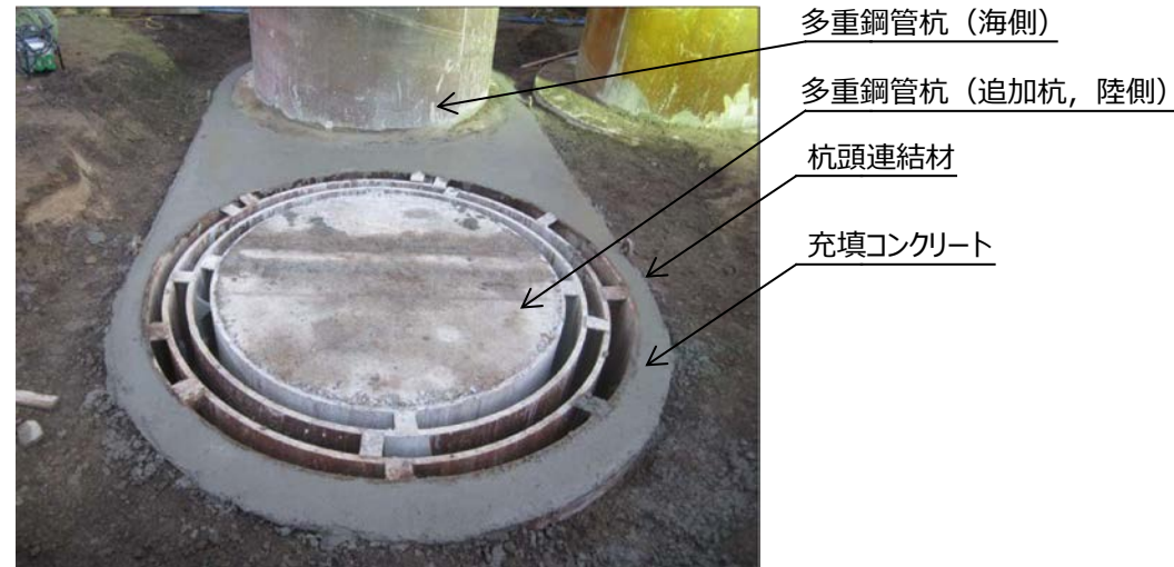
杭頭連結材設置状況 (間詰めコンクリート打設前)
