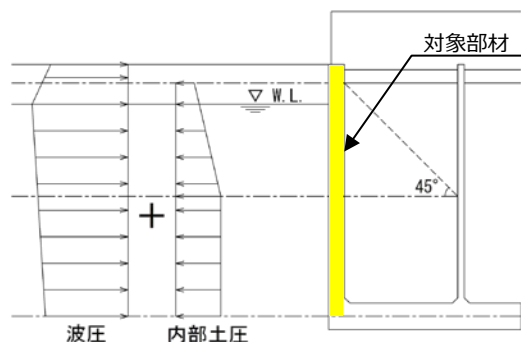
側壁（前壁）に生じる作用イメージ図 （津波時、陸側への作用）
