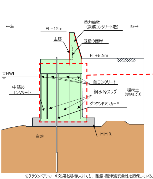
防波壁断面図 (波返重力擁壁)
