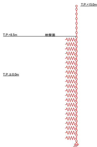
多重鋼管杭式擁壁 解析モデル図(例)
