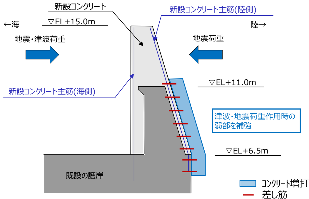
対策工の構造例
