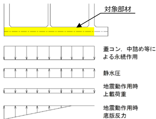
底板に生じる作用イメージ図（地震動作用時）
