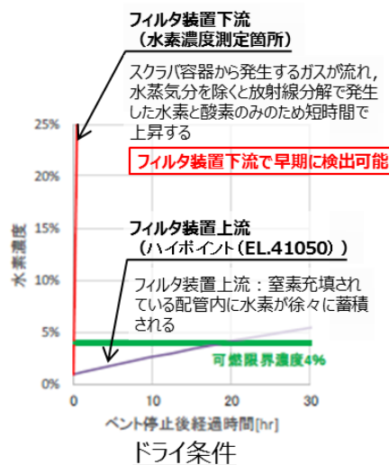
図3 D/W ベント時の格納容器フィルタベント系配管の水素濃度 (ベント停止時の窒素パーージ中断時)
