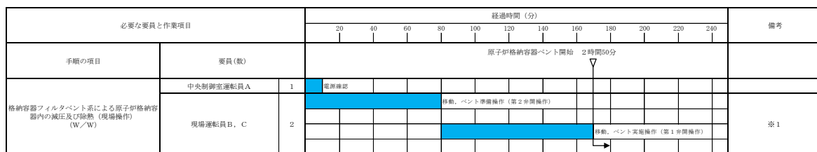
第 3.7-2 図 格納容器フィルタベント系による原子炉格納容器内の減圧及び除熱 (W/W) タイムチャート (現場操作による格納容器ベント) *
