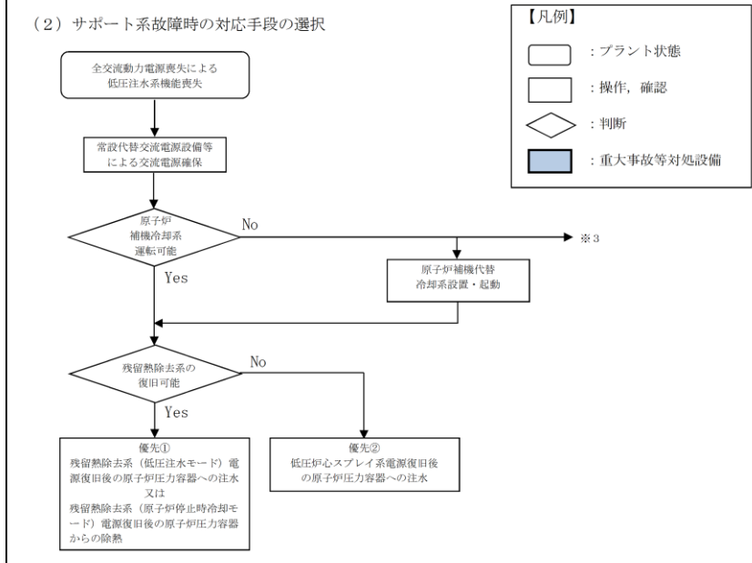
第1.4-33図 重大事故等発生時の対応手段選択フローチャート (2/3)
