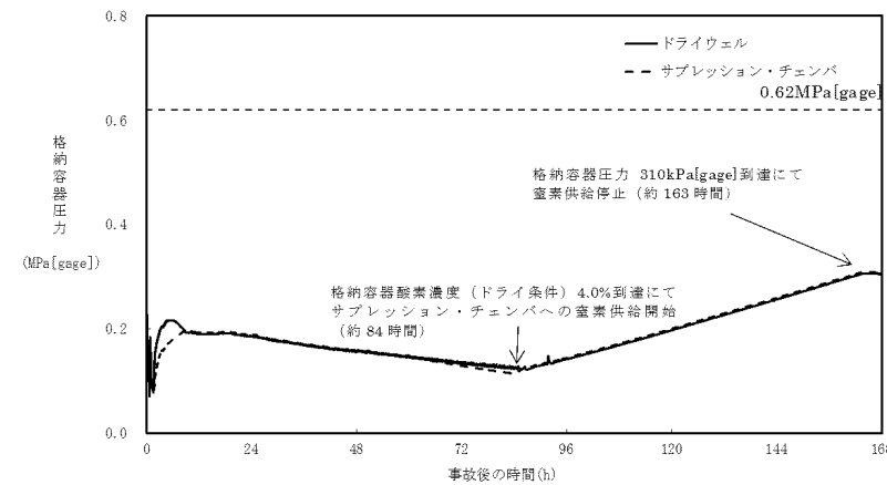
第1図 格納容器圧力
