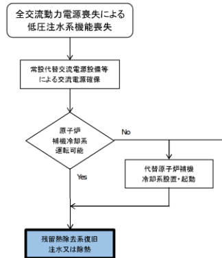
第 1.4.32 図 重大事故等発生時の対応手段選択フローチャート (1/2)
