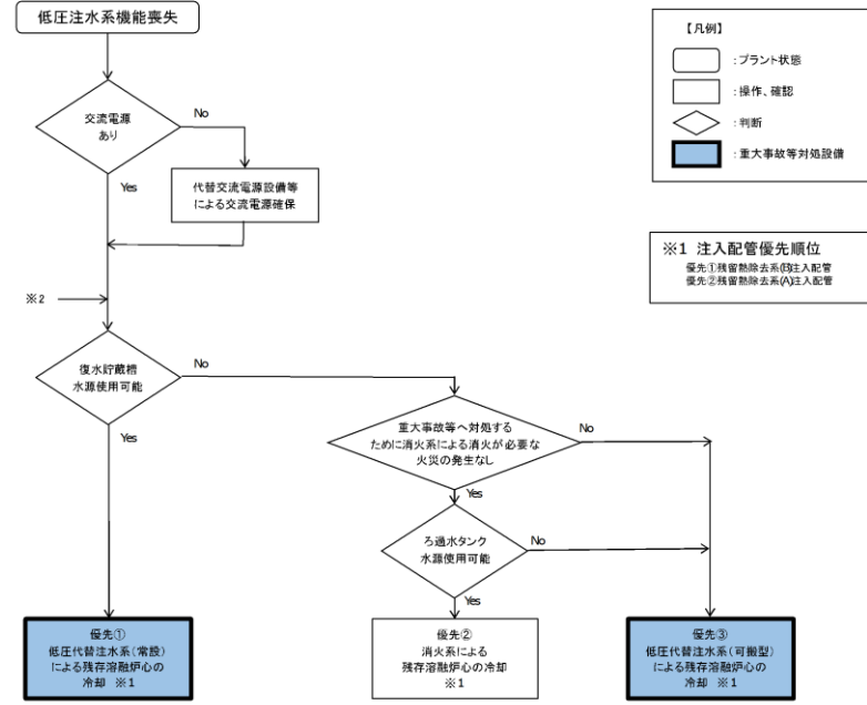
第 1. 4. 32 図 重大事故等発生時の対応手段選択フローチャート
