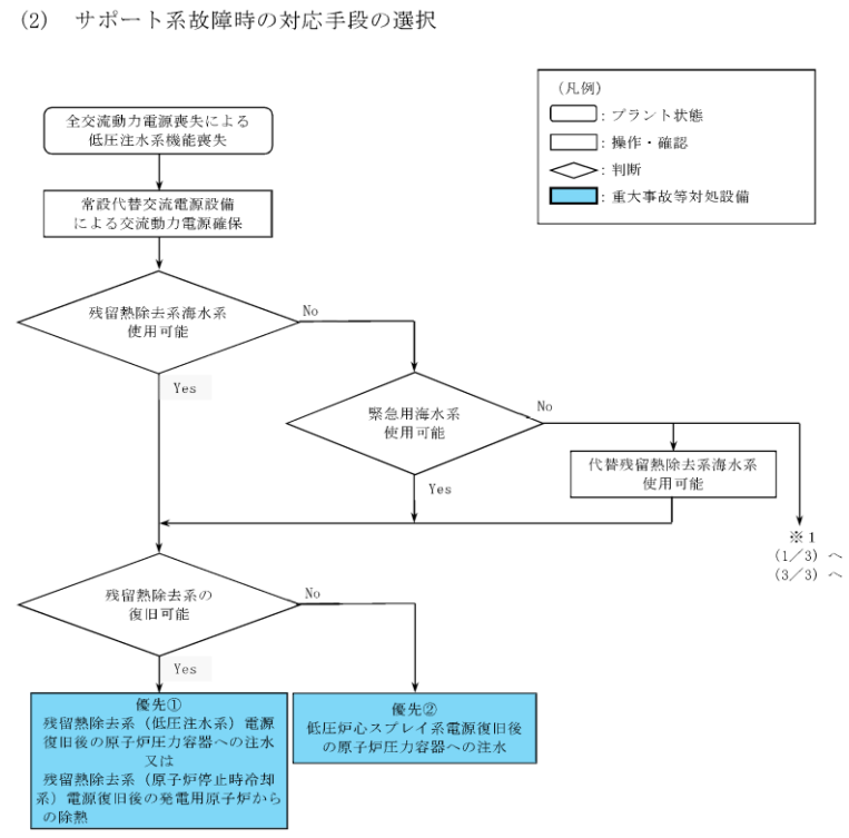
第1.4-35図 重大事故等時の対応手段選択フローチャート (2/3)
