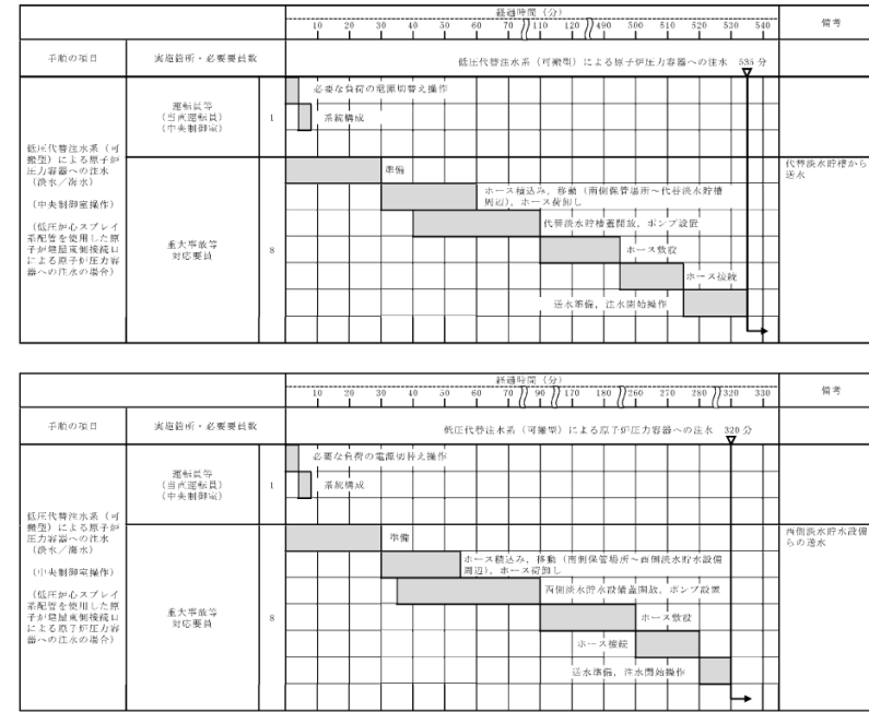
【ホース敷設(代替淡水貯槽から原子炉建屋東側接続口)の場合は542m, ホース敷設(西側淡水貯水設備から原子炉建屋東側接続口)の場合は881m】
