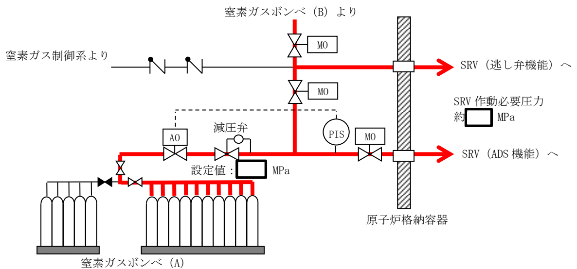
b. 系統压力低下時またはSA時(炉心損傷前)の窒素ガスポンベによる窒素ガス供給
